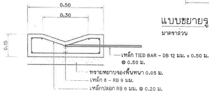
ขยายตัดรางวี คสล. มาตรฐาน 1 : 10
