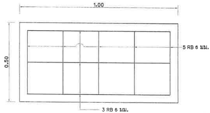
แบบขยายแปลนแผ่นพื้นรองท้อ มาตรฐาน 1 : 10
