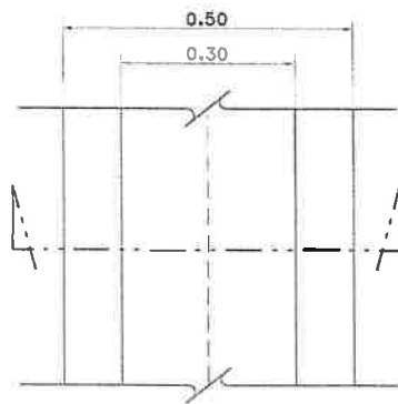
แบบขยายแปลนรางวี คสล. มาตรฐาน 1 : 10
