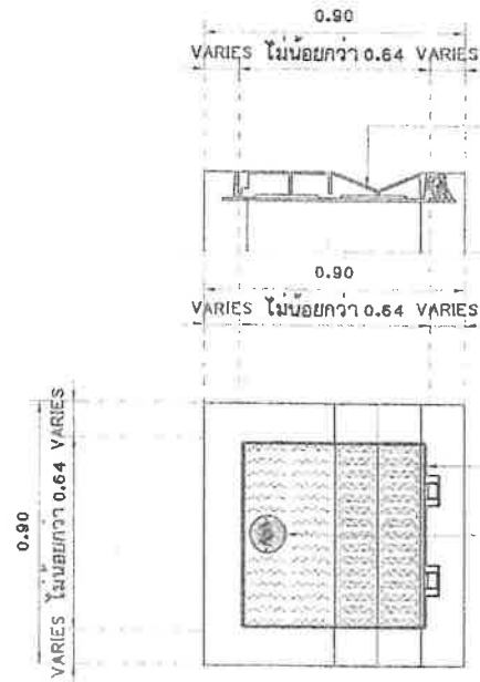
แบบขยายฝาบ่อพักเหล็กหล่อเหนียว 1 มาตราส่วน 1:20
