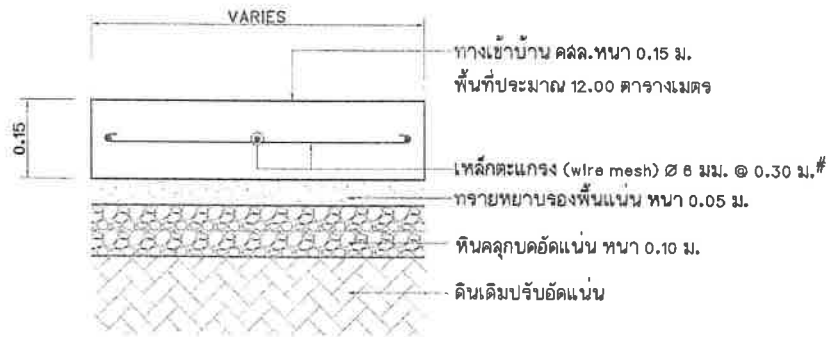
แบบขยายรูปตัดทางเข้าบ้าน คสล.หนา 0.15 ม. มาตรฐาน 1 : 10
