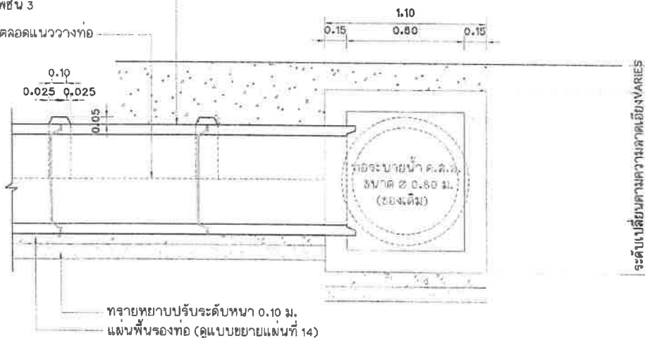
รูปตัดการเชื่อมต่อระบายน้ำของเดิม มาตราส่วน 1:25
