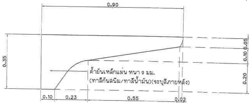
แบบขยายแผ่นเหล็กค้ำยันระยะความกว้างหลังคา 2.00 เมตร
