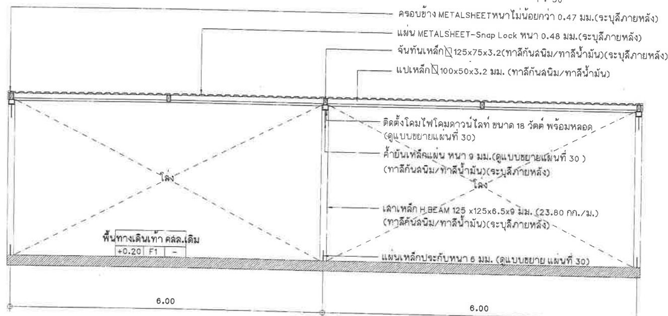
รูปตัดปรับปรุงหลังคาชั้นลาดคลุมทางเดินระยะห่างระหว่างเสา 6.00 เมตร มาตราส่วน 1 : 50
