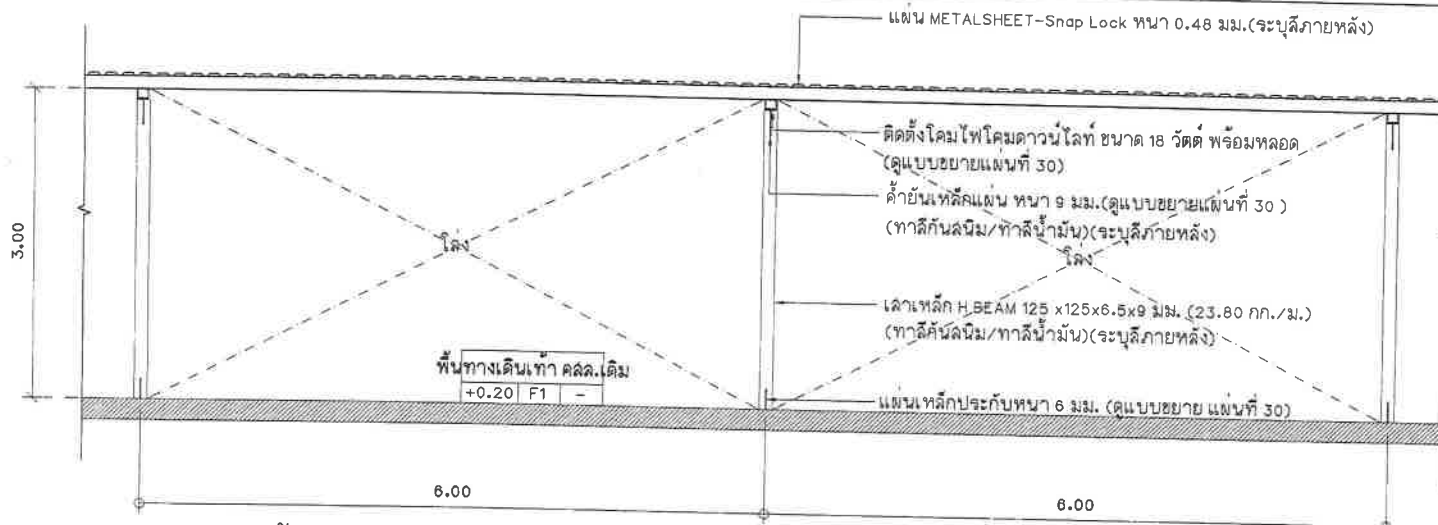
รูปด้านปรับปรุงหลังคาชั้นลาดคลุมทางเดินระยะห่างระหว่างเสา 6.00 เมตร มาตราส่วน 1 : 50
