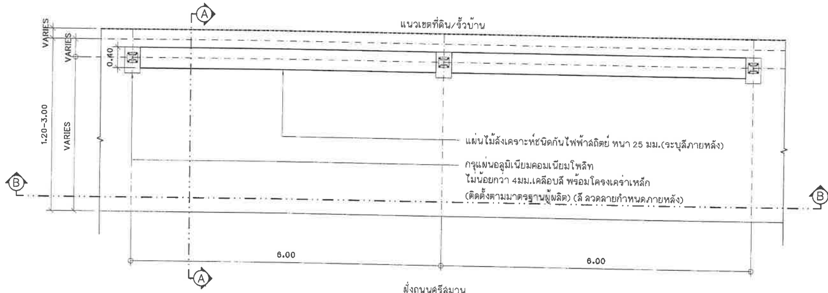
แปลนพื้นที่จุดพักคอยรถประจำทาง มาตราส่วน 1:50
