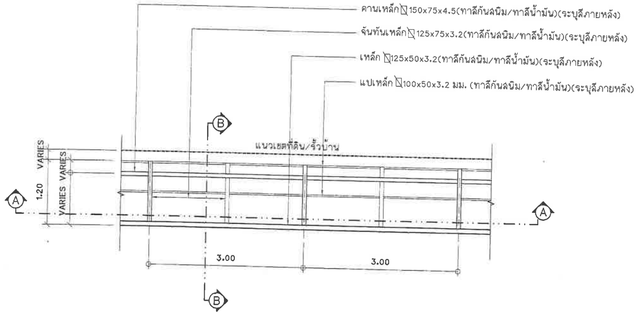
แปลนปรับปรุงโครงสร้างหลังคาถนนลาดคลุมทางเดินระยะห่างระหว่างเสา 3.00 เมตร มาตราส่วน
