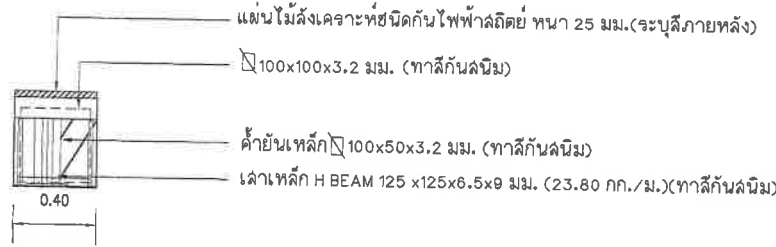
แบบขยายโครงสร้างป้ายจุดพักคอยรถประจำทาง/กรุที่นั่งพักคอย มาตรฐาน 1:25
