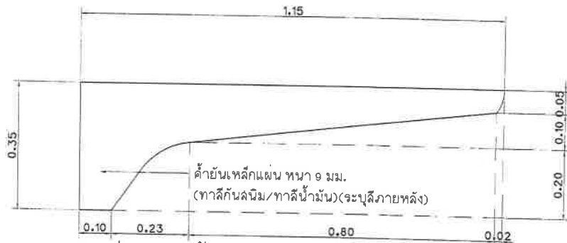
แบบขยายแผ่นเหล็กค้ำยันระยะความกว้างหลังคา 3.00 เมตร
