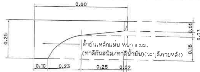
แบบขยายแผ่นเหล็กค้ำยันระยะความกว้างหลังคา 1.20 เมตร
