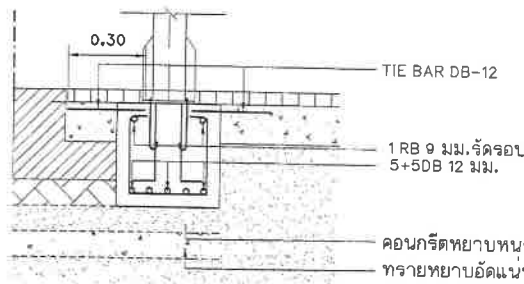
แบบขยายรูปตัดฐานราก 2 มาตราส่วน 1 : 20
