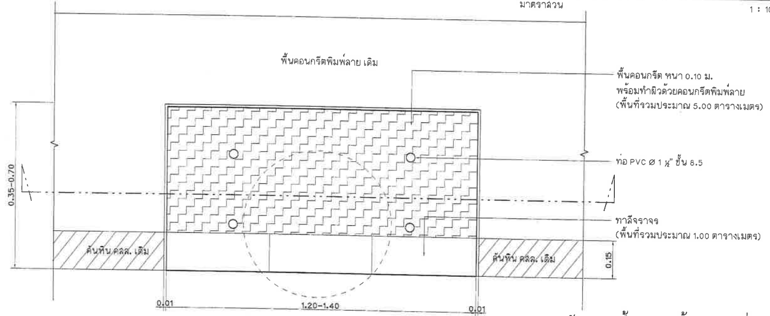
แบบขยายปรับปรุงพื้นทางเท้า (มีฝาบ่อ)
