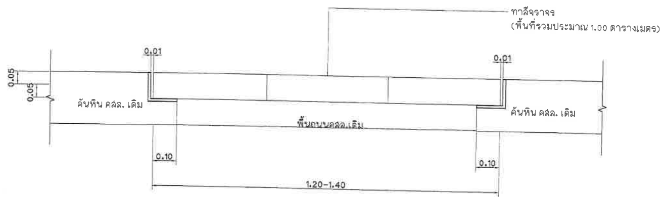
รูปด้านแบบขยายปรับปรุงพื้นทางเท้า (มีฝาบ่อ) มาตราส่วน 1 : 10
