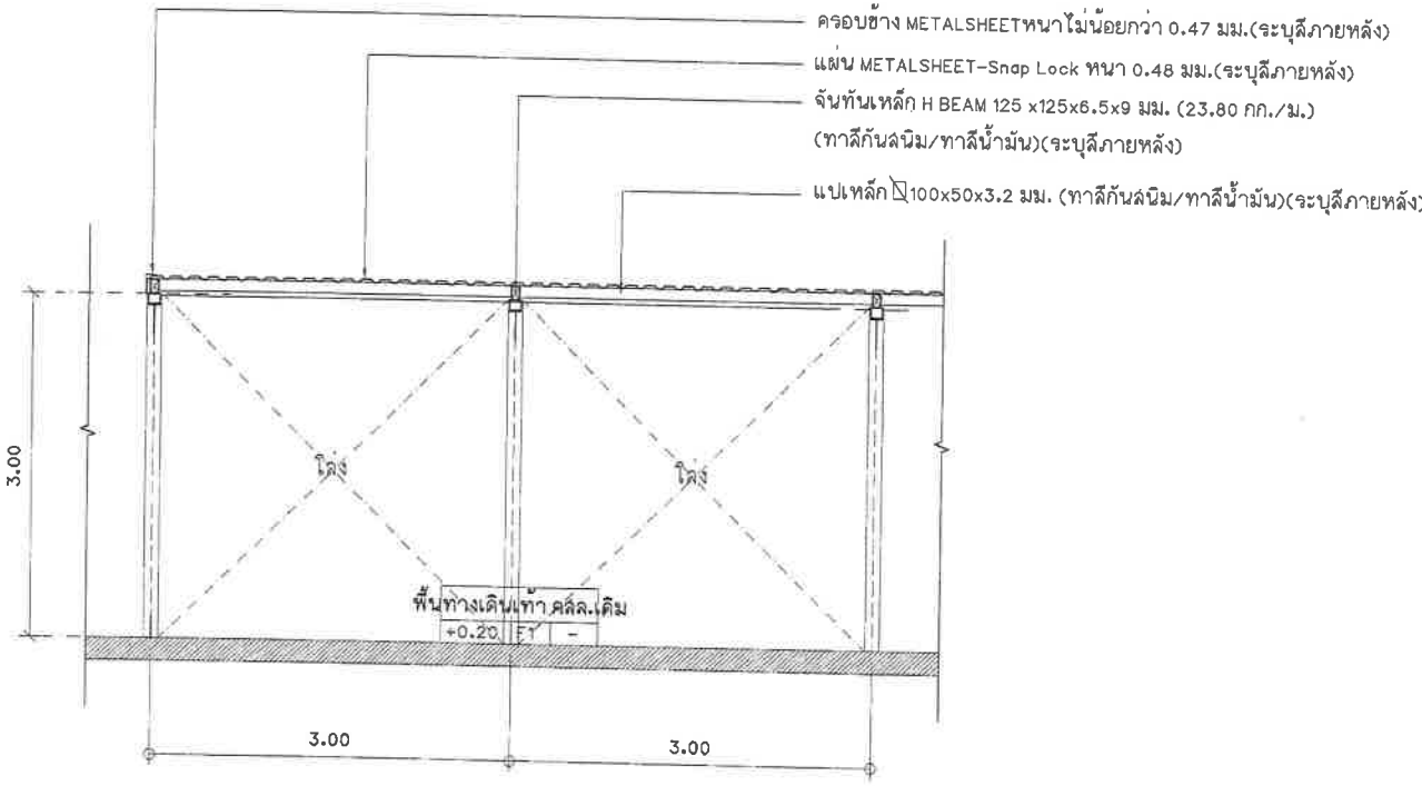
รูปตัดปรับปรุงหลังคาถ้ำกันล่าตงทางเดินเท้าระยะห่างระหว่างเสา 3.00 เมตร มาตราส่วน 1 : 50
