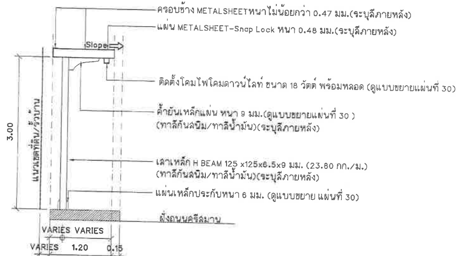
รูปด้านระยะหลังคากว้าง 1.20 เมตร
