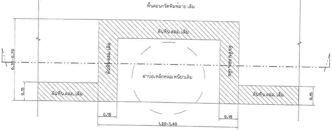
แบบขยายพื้นทางเท้าเดิม (มีฝาบ่อ)
