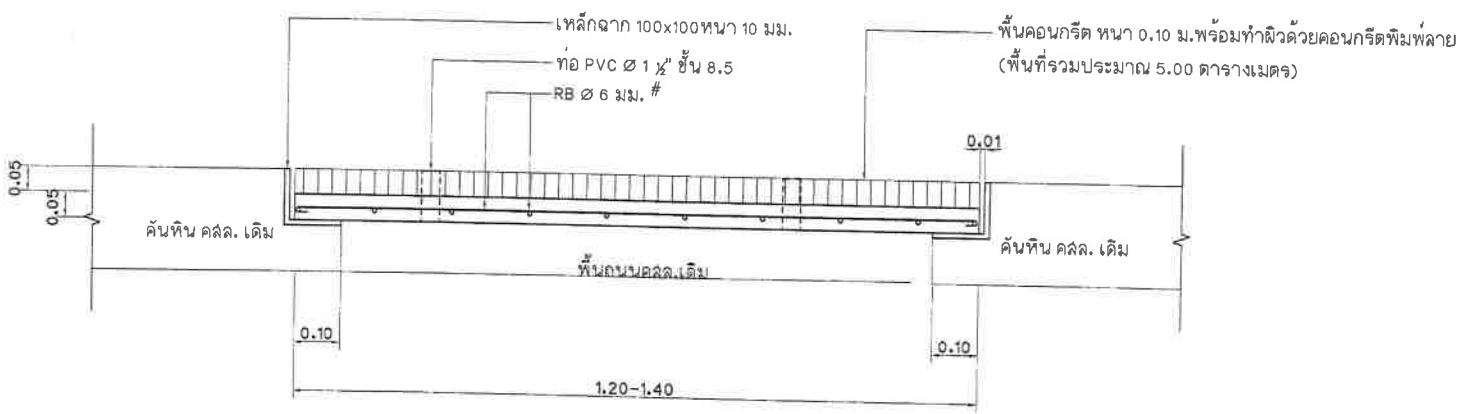
รูปตัดแบบขยายปรับปรุงพื้นทางเท้า (มีฝาบ่อ) มาตราส่วน 1 : 10
