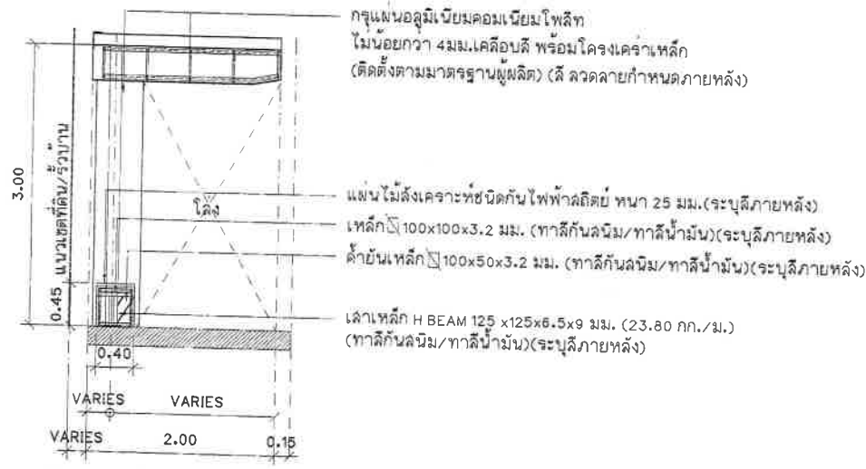
รูปตัด 2 จุดพักคอยรถประจำทาง มาตรฐาน 1:50
