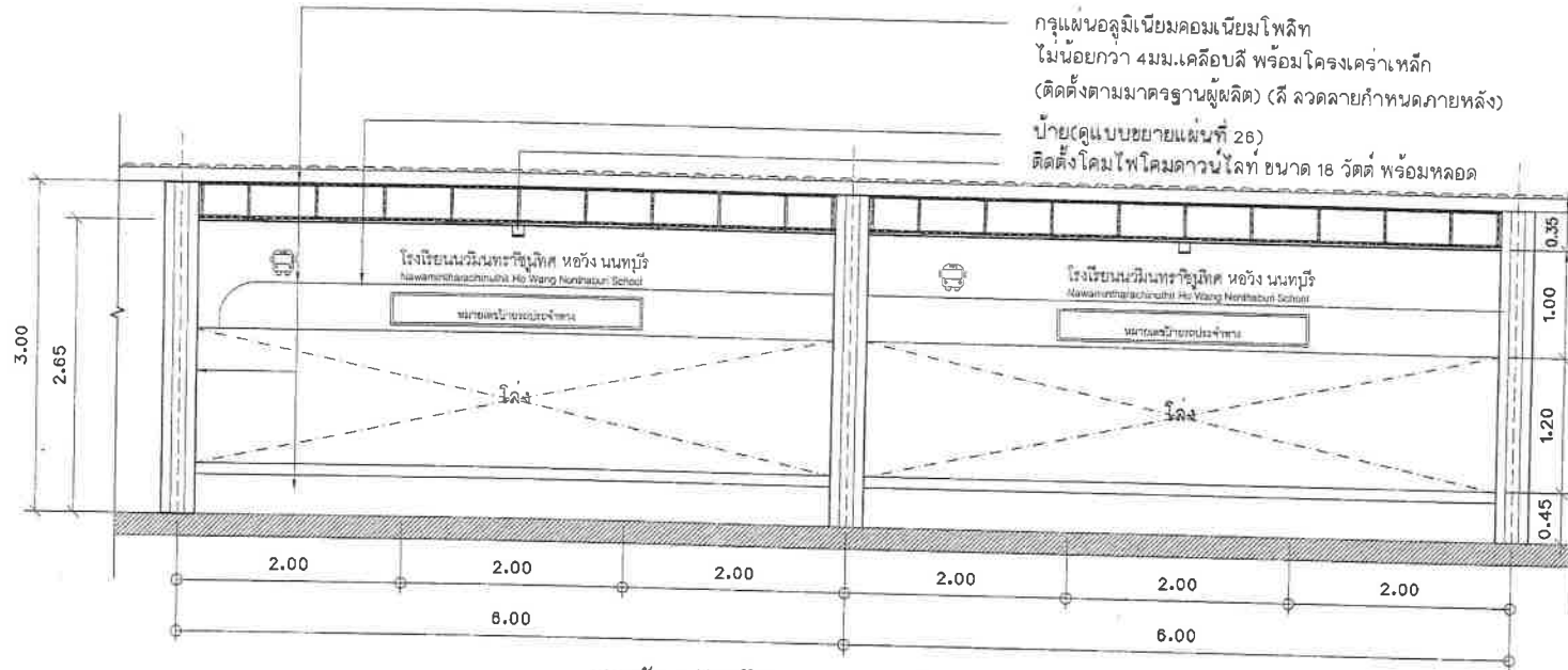
รูปตัด 1 จุดพักคอยรถประจำทาง มาตรฐาน 1:50
