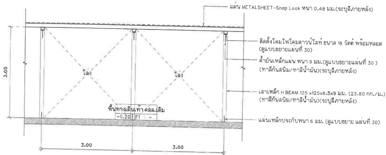
รูปด้านปรับปรุงหลังคากันลาดคลุมทางเดินระยะห่างระหว่างเสา 3.00 เมตร
