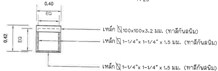
แบบขยายโครงสร้างป้ายจุดพักคอยรถประจำทาง/กรุที่นั่งพักคอย มาตรฐาน 1:25
