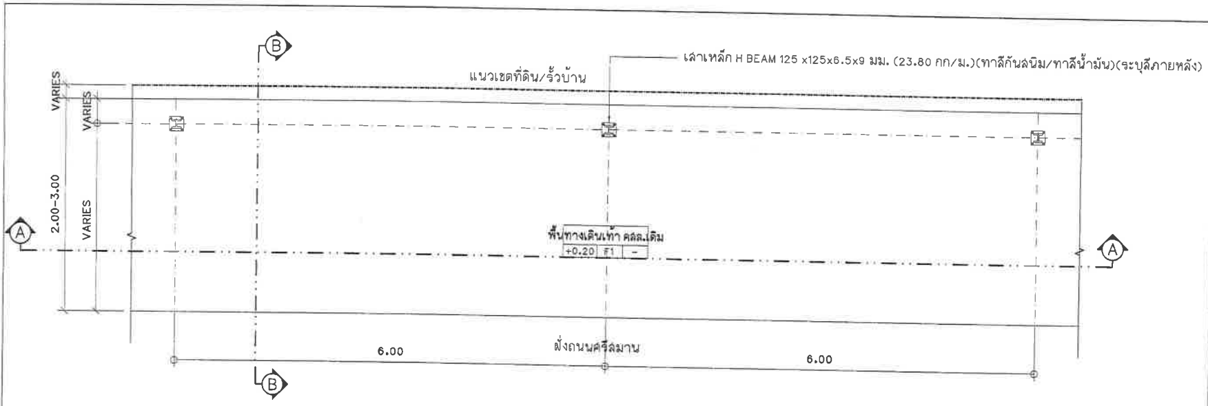
แปลนพื้นทางเดินคสล.ระยะห่างระหว่างเสา 6.00 เมตร มาตรฐาน 1:50
