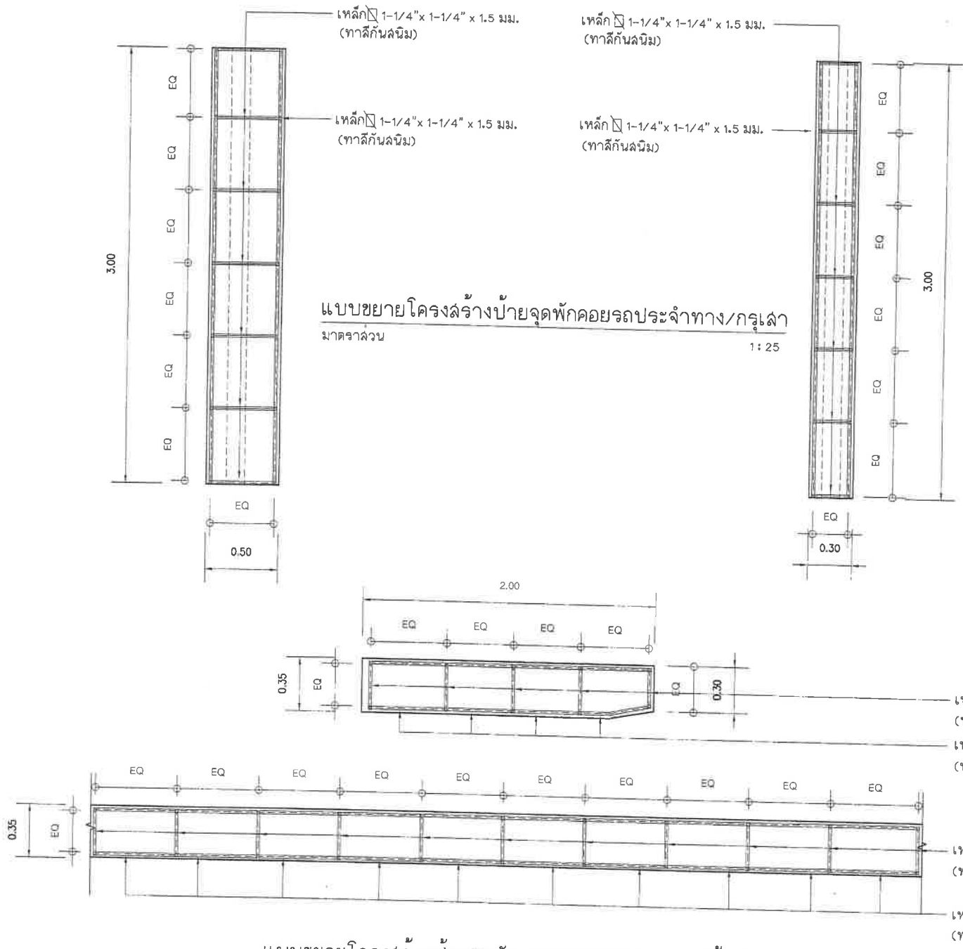
แบบขยายโครงสร้างป้ายจุดพักคอยรถประจำทาง/กรุใต้หลังคา มาตราส่วน 1:25
