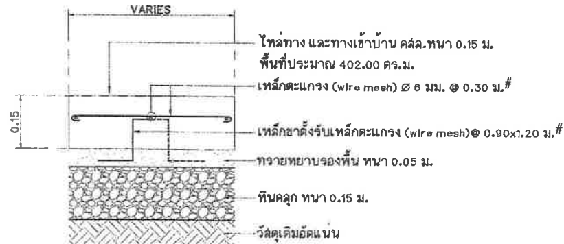
ไหล่ทาง และทางเข้าบ้าน คสล.หนา 0.15 ม. มาตราส่วน 1 : 10
