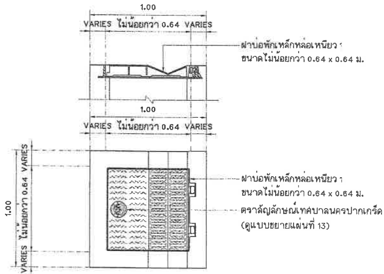
แบบขยายฝาบ่อพักเหล็กหล่อเหนียว 1 มาตราส่วน 1:20
