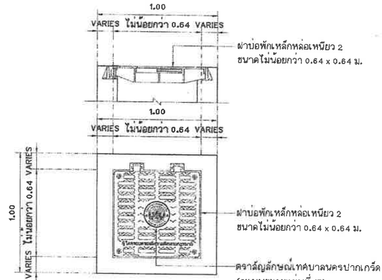
แบบขยายฝาบ่อพักเหล็กหล่อเหนียว 2 มาตราส่วน 1:20 (ฝาบ่อพัก และกรอบเป็นชนิดกันเสียงโดยเฉพาะ)
