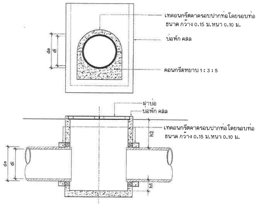
การประสาณท่อ HDPE เข้าบ่อ คลล.
