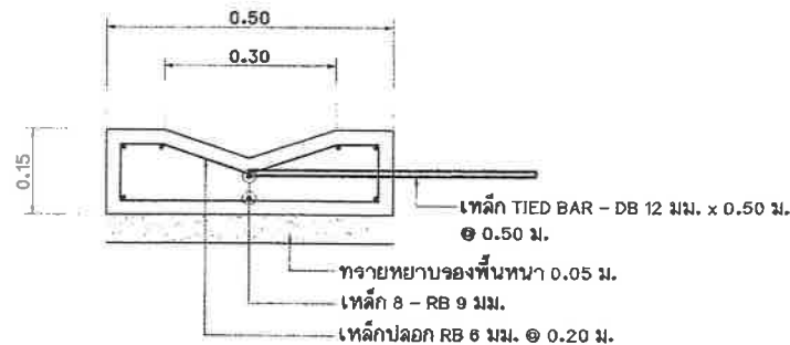
ขยายตัดรางวี คสล. มาตราส่วน 1 : 10
