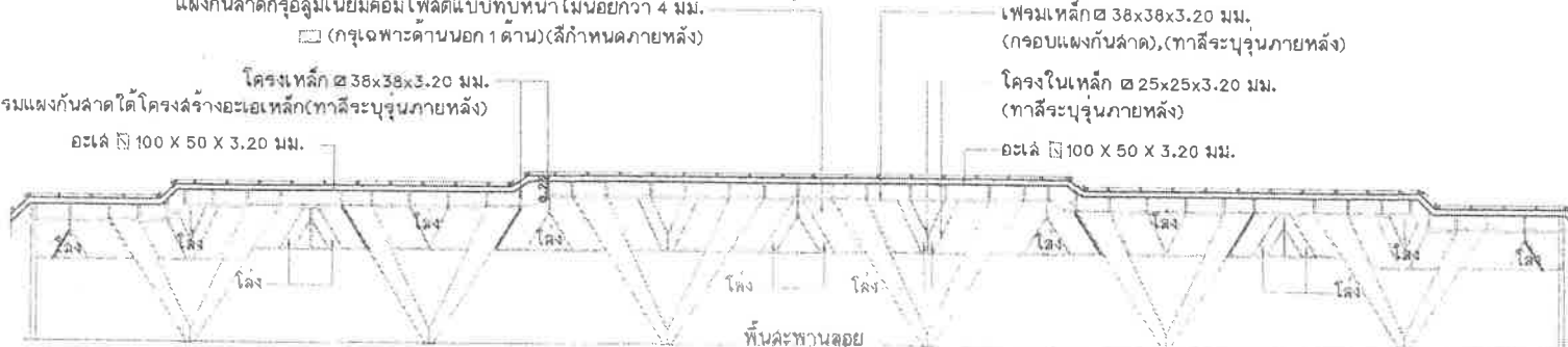
แผงกันล้าดรูปด้าน A (บนสะพานลอย)
