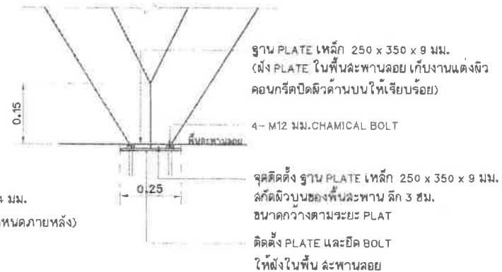
รูปตัดขยาย PLATE-1 ยึดเสา (บนละพานลอย) มาตรฐาน 1 : 10
