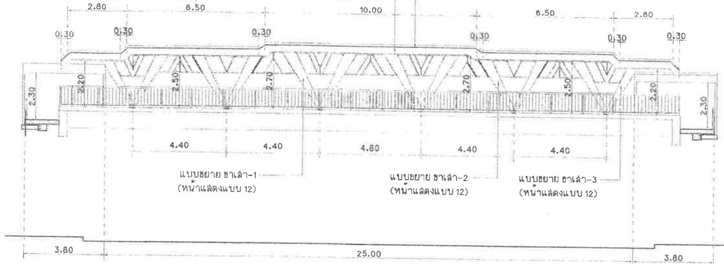
รูปด้าน ③ มาตรฐาน 1 : 125
