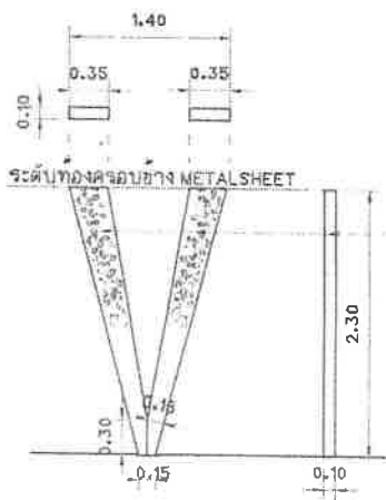
แบบขยาย ขาเสา (ข้ามพีกสะพานลอย) มาตราส่วน 1 : 50
