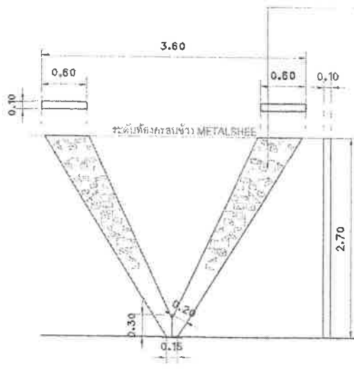
แบบขยาย ขาเสา-1 (สะพานลอย) มาตราส่วน 1 : 50
