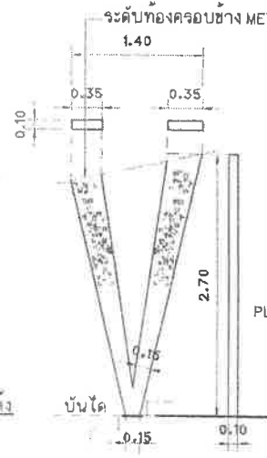
แบบขยาย ขาเสา (บันได) มาตราส่วน 1 : 50
