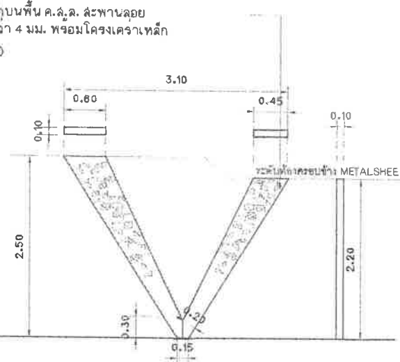
แบบขยาย ขาเสา-3 (สะพานลอย) มาตราส่วน 1 : 50
