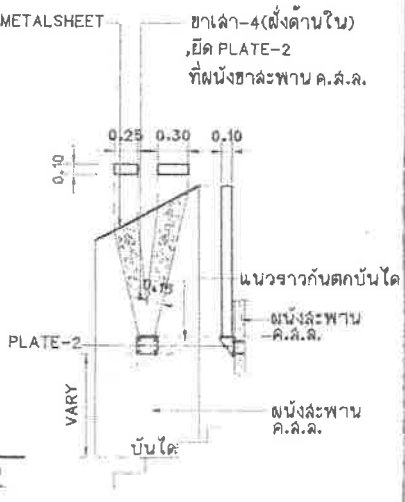
แบบขยาย ขาเสา-4 (ฝั่งด้านใน) มาตราส่วน 1 : 50
