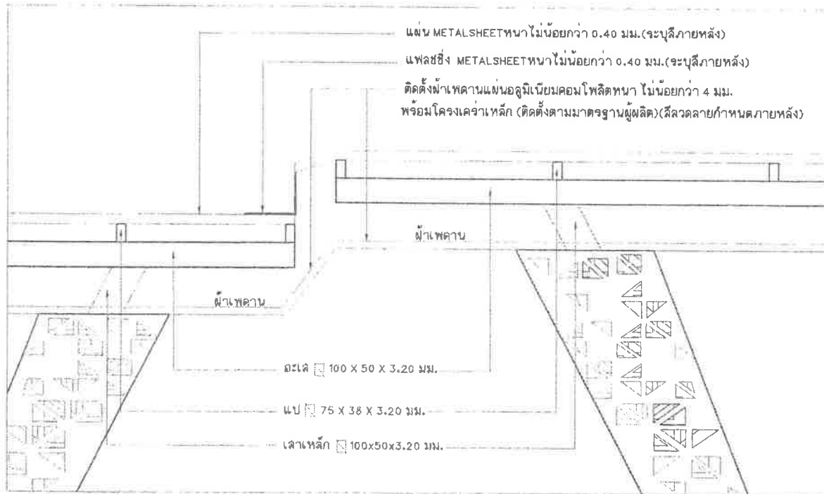
แบบขยายการติดตั้งโครงหลังคา มาตรฐาน 1 : 10
