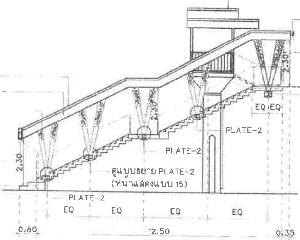
รูปด้าน ④ มาตรฐาน 1 : 125
