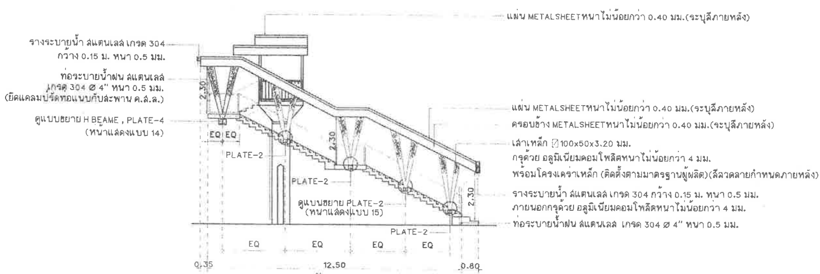
รูปด้าน ② มาตราส่วน 1 : 125
