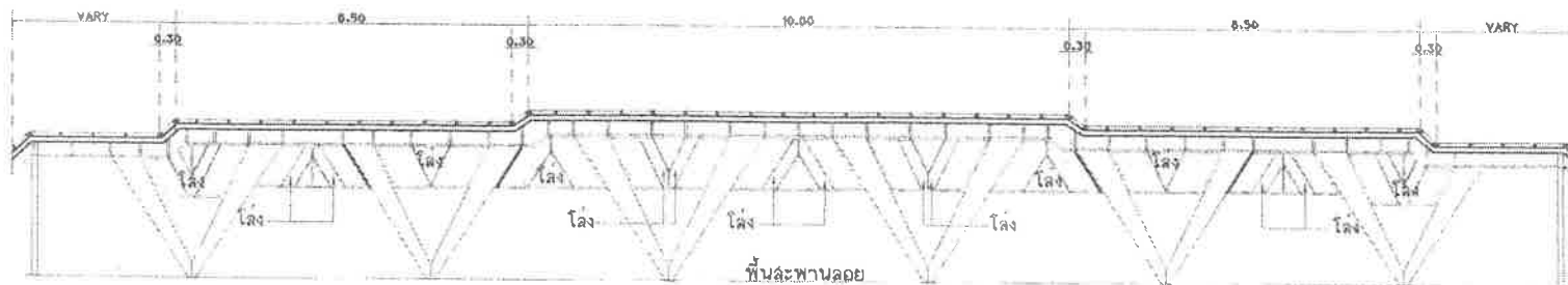
แผงกันล้าดรูปด้าน B (บนสะพานลอย)
