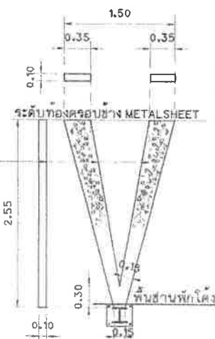
แบบขยาย ขาเสา (ข้ามพีกโค้ง) มาตราส่วน 1 : 50
