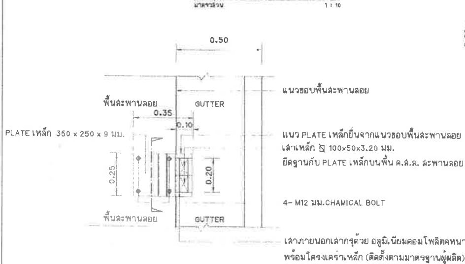
แบบขยายการติดตั้งโครงหลังคา มาตรฐาน 1 : 10
