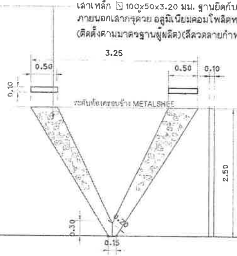
แบบขยาย ขาเสา-2 (สะพานลอย) มาตราส่วน 1 : 50
