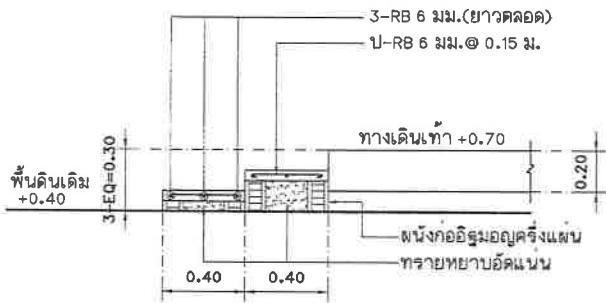
แบบขยายรูปตัดบันได ST1 (สะพานที่ 2) มาตรฐาน 1: 25
