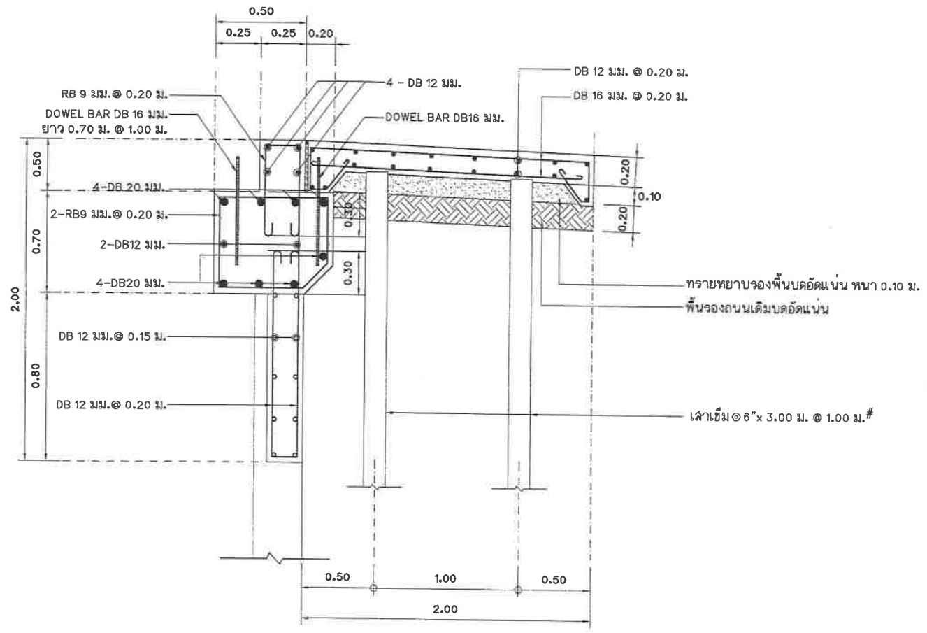
รูปตัดการเชื่อมสะพาน และผิวถนน คสล. (ฝั่งถนนสามัคคี)
