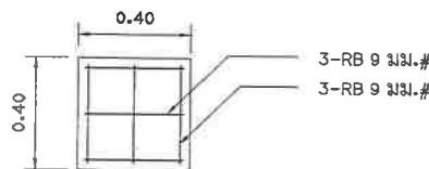
แบบขยายฐานเสา CX-2 มาตราส่วน 1:20
