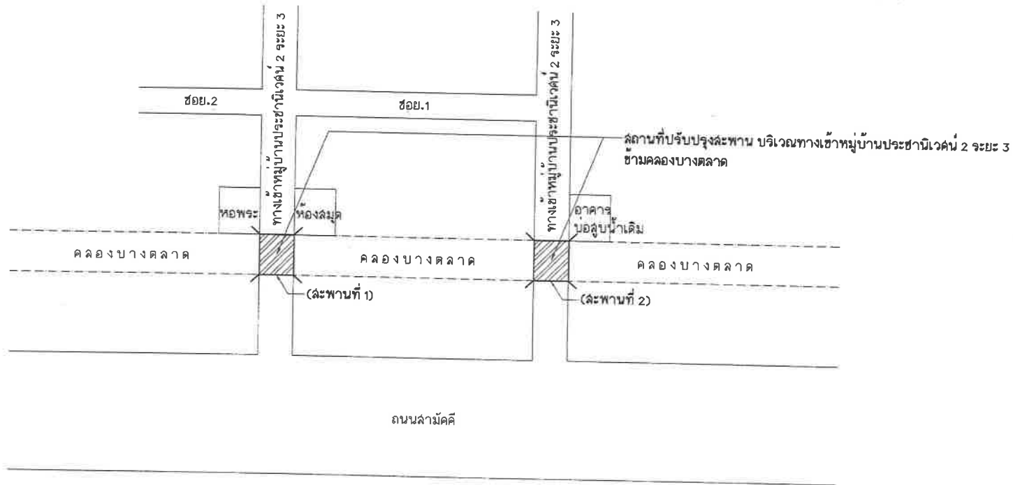
ผังตำแหน่งปรับปรุงสะพาน (สะพานที่ 1 และ สะพานที่ 2)
