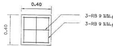
แบบขยายฐานเสา CX-2
