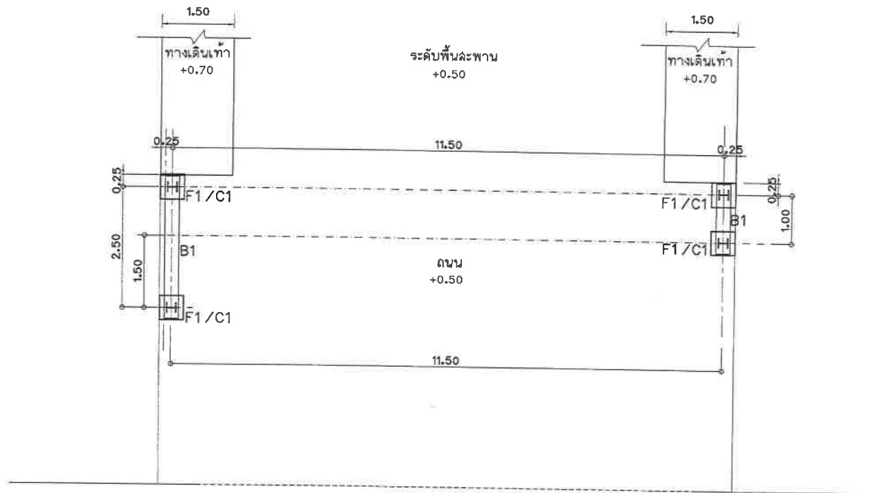
ผังฐานราก F1/C1
