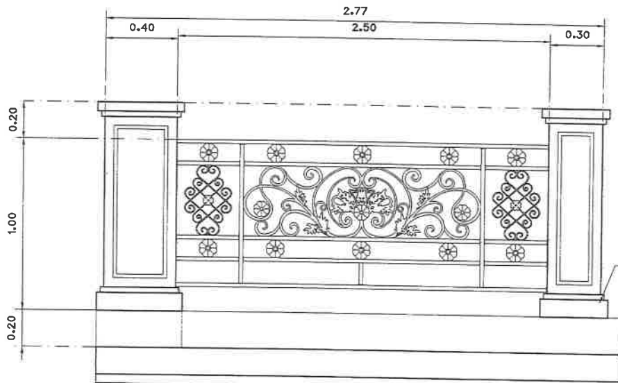
แบบขยายรูปด้านหน้าราวสะพานเหล็กคัตอิतालีย์ (สะพานที่ 2)
