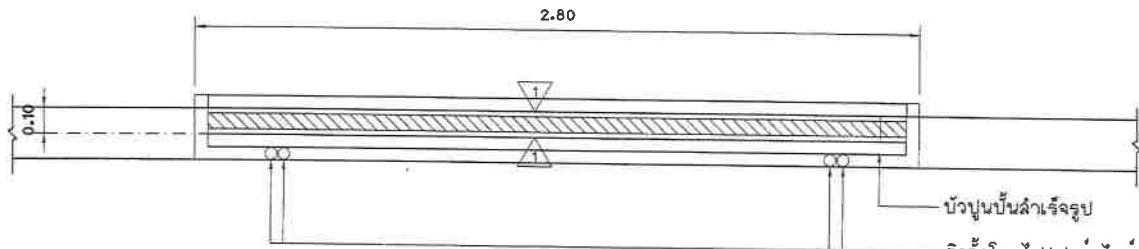
แบบขยายแปลนป้ายสะพาน คสล.(สะพานที่ 1) มาตราส่วน 1:20
