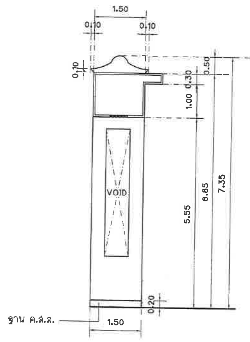
รูปตัดขาซุ้ม (ฝั่งขวาด้านใน) มาตราส่วน 1:75
