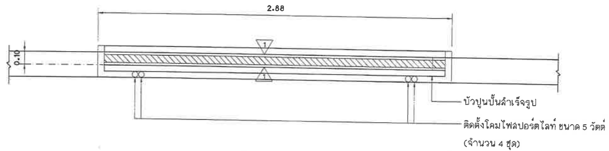
แบบขยายแปลนป้ายสะพาน คสล. (สะพานที่ 1) มาตราส่วน 1: 20
