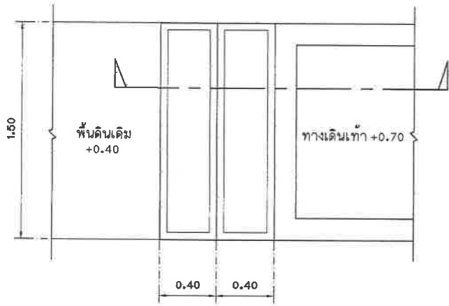
แบบขยายแปลนบันได ST1 (สะพานที่ 2) มาตรฐาน 1: 25
