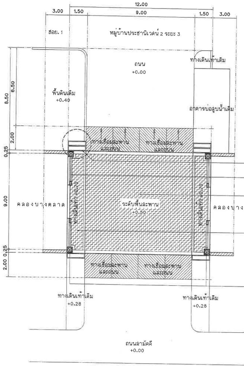
แปลนสะพาน คสล. (สะพานที่ 2) มาตรฐาน 1:125
