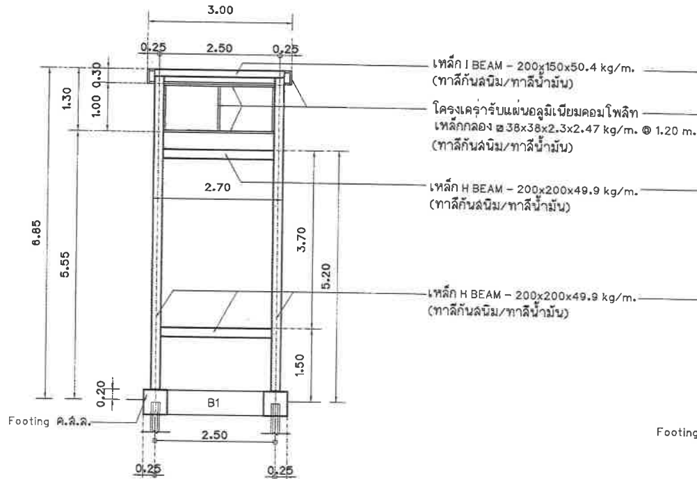
รูปตัดโครงสร้างเหล็ก A มาตราส่วน 1:75
