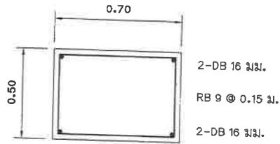
แบบขยาย B1 มาตราส่วน 1:20
