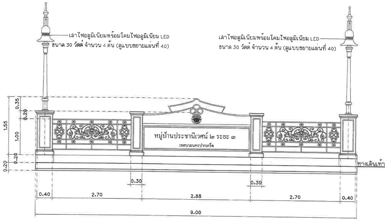
รูปด้านหน้าราวสะพาน คลล.พร้อมป้าย (สะพานที่ 2)
