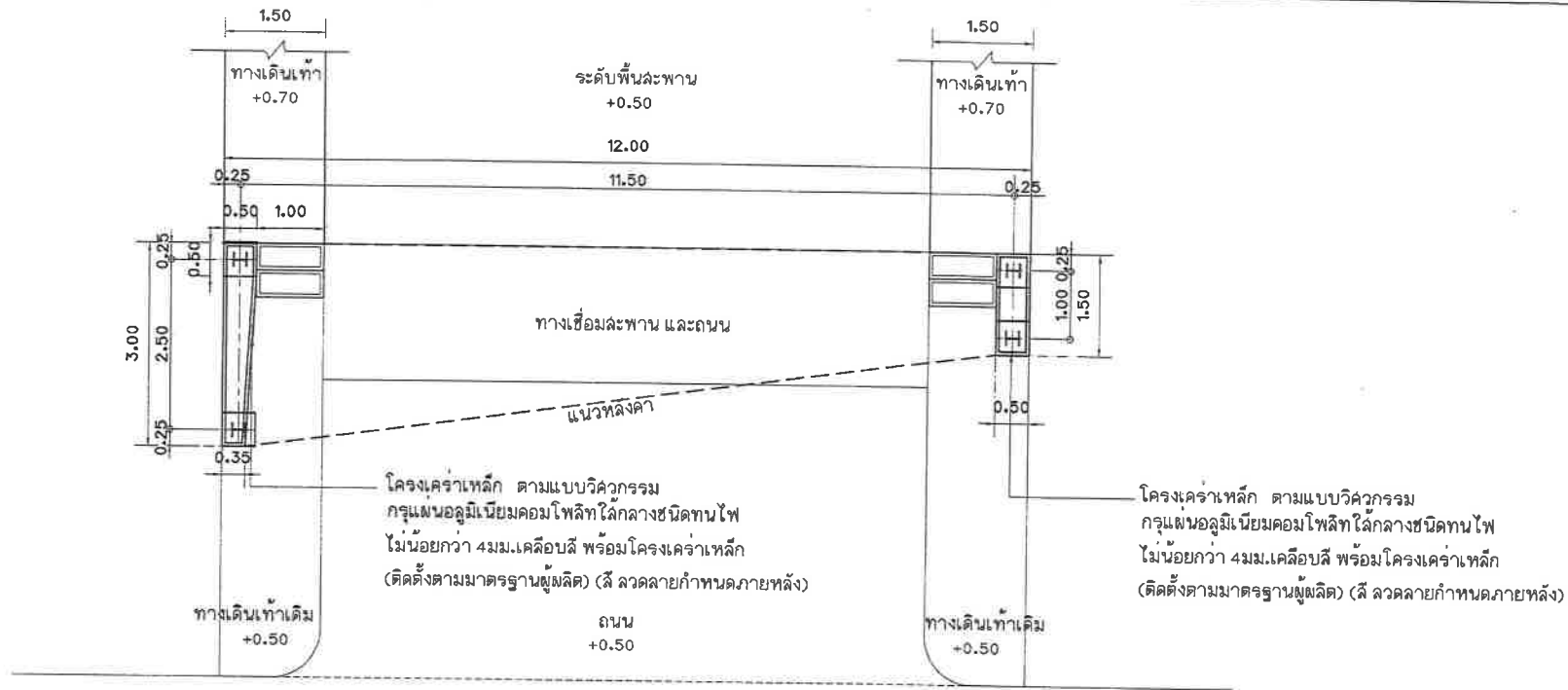
แปลนชุมทางเข้าหมู่บ้าน มาตราส่วน 1:75
