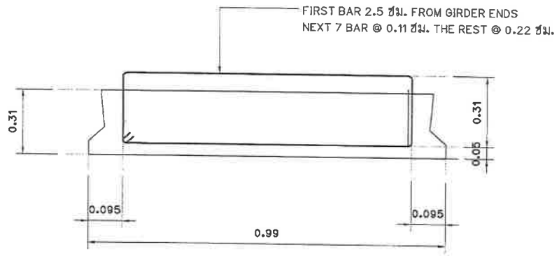
PLANK 9.00 ม. SPAN
