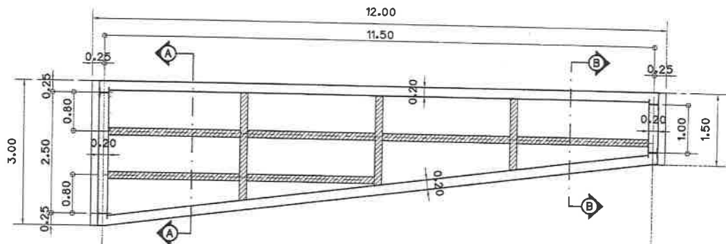
โครงสร้างเหล็กหลังคา มาตราส่วน 1:75
