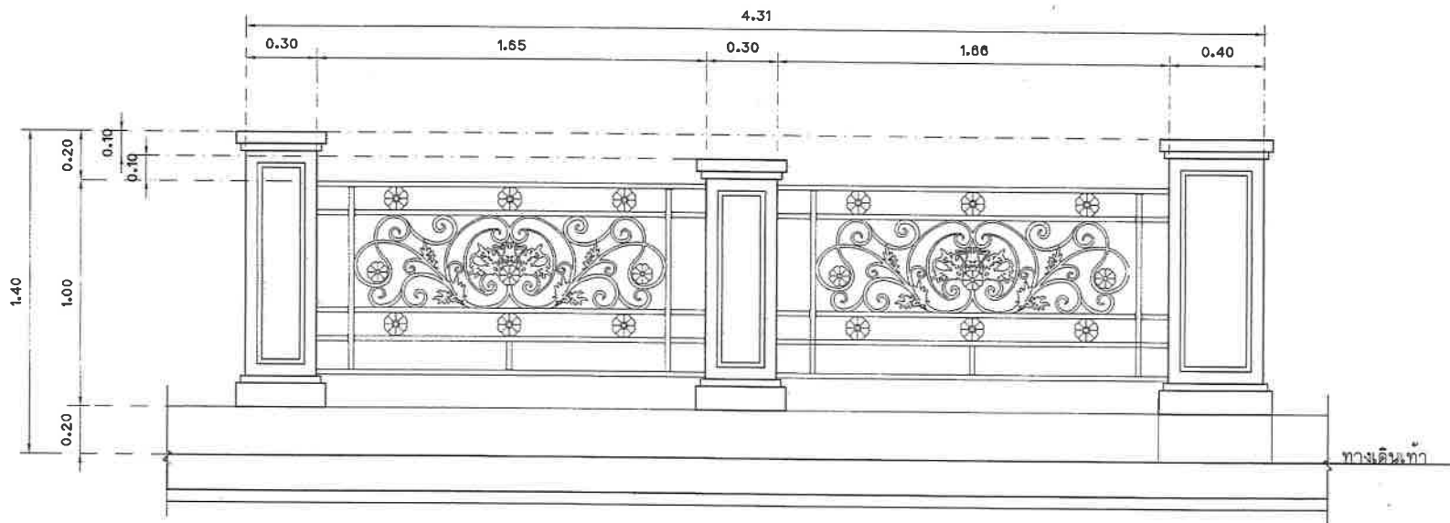
แบบขยายรูปด้านหน้าราวสะพานเหล็กคัตอิตาลี (สะพานที่ 1) มาตราส่วน 1:20
