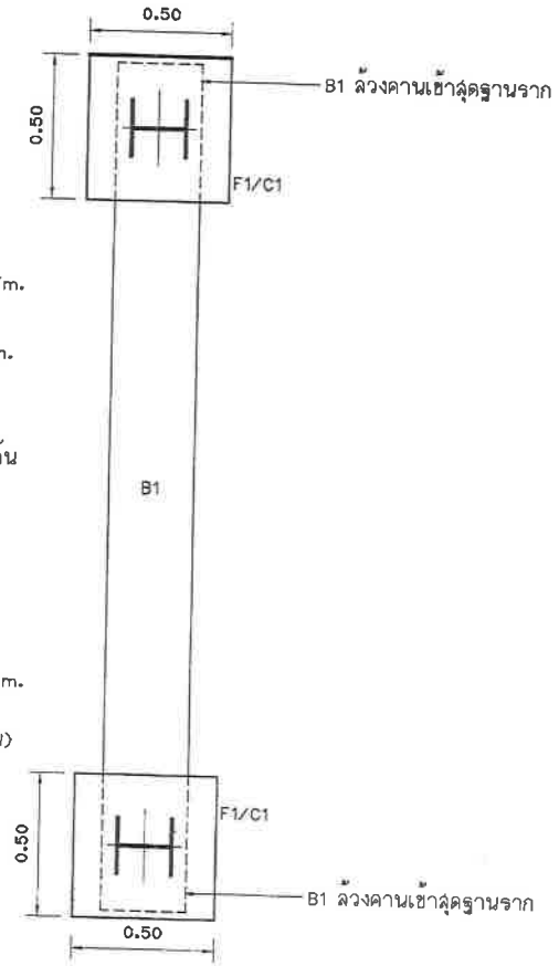
แปลนขยาย B1 (ฐานขาขั้วมทางเข้าฝั่งซ้าย) มาตราส่วน 1:20
