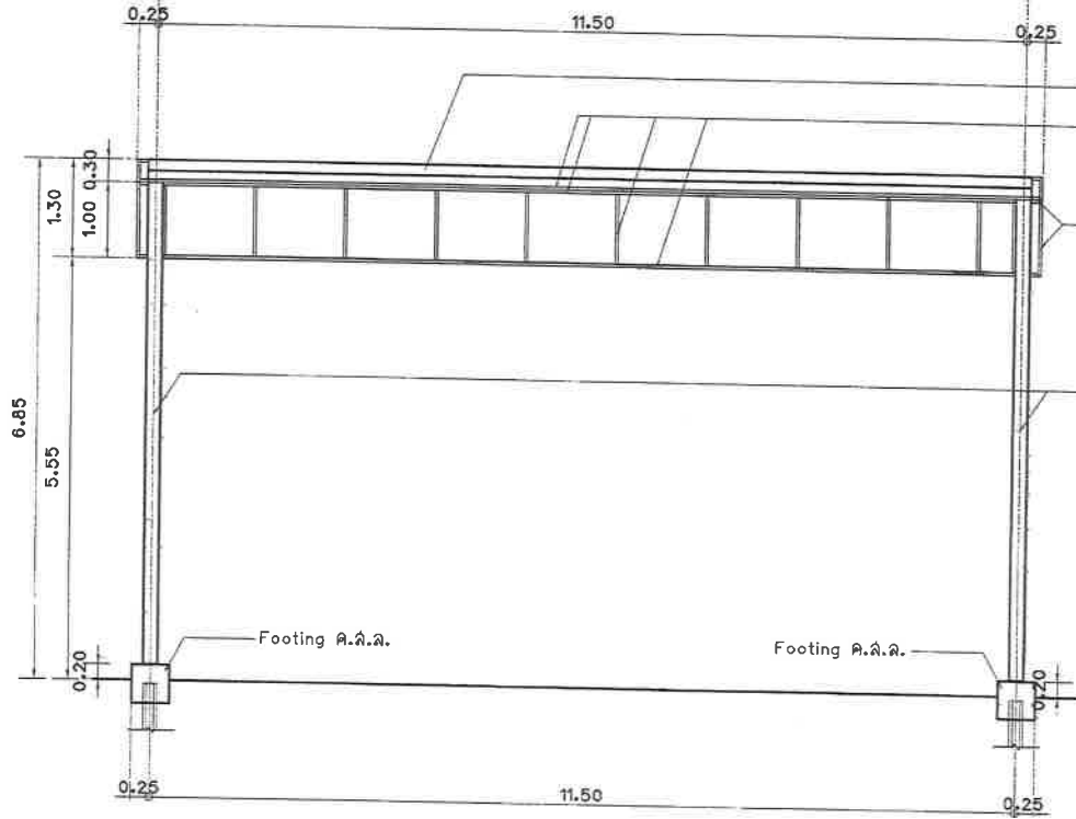
รูปด้านโครงสร้างเหล็กรูปพรรณ มาตราส่วน 1:75
