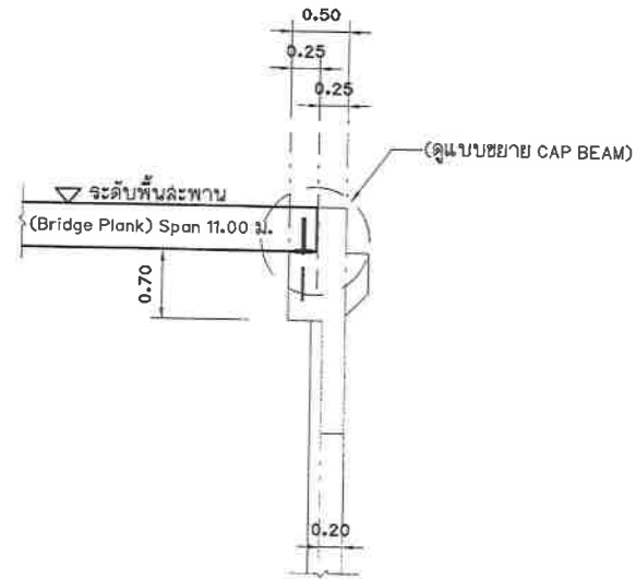
CAP BEAM มาตราส่วน 1:50
