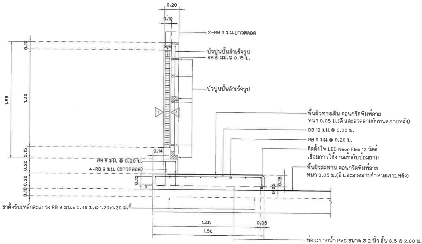
แบบขยายรูปตัดโครงสร้างป้ายสะพาน คสล.พื้นทางเดินเท้า (สะพานที่ 1) มาตราส่วน 1:20
