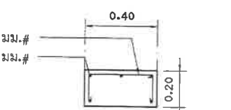
รูปตัดขยายฐานเสา CX-2
