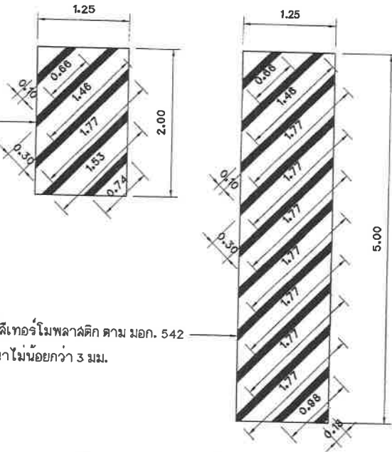
แบบขยายตีเส้นจราจรทางเชื่อมสะพาน และถนน คสล. มาตราส่วน 1:50
