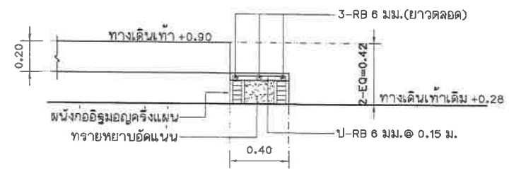
แบบขยายรูปตัดบันได ST2 (สะพานที่ 2) มาตรฐาน 1: 25
