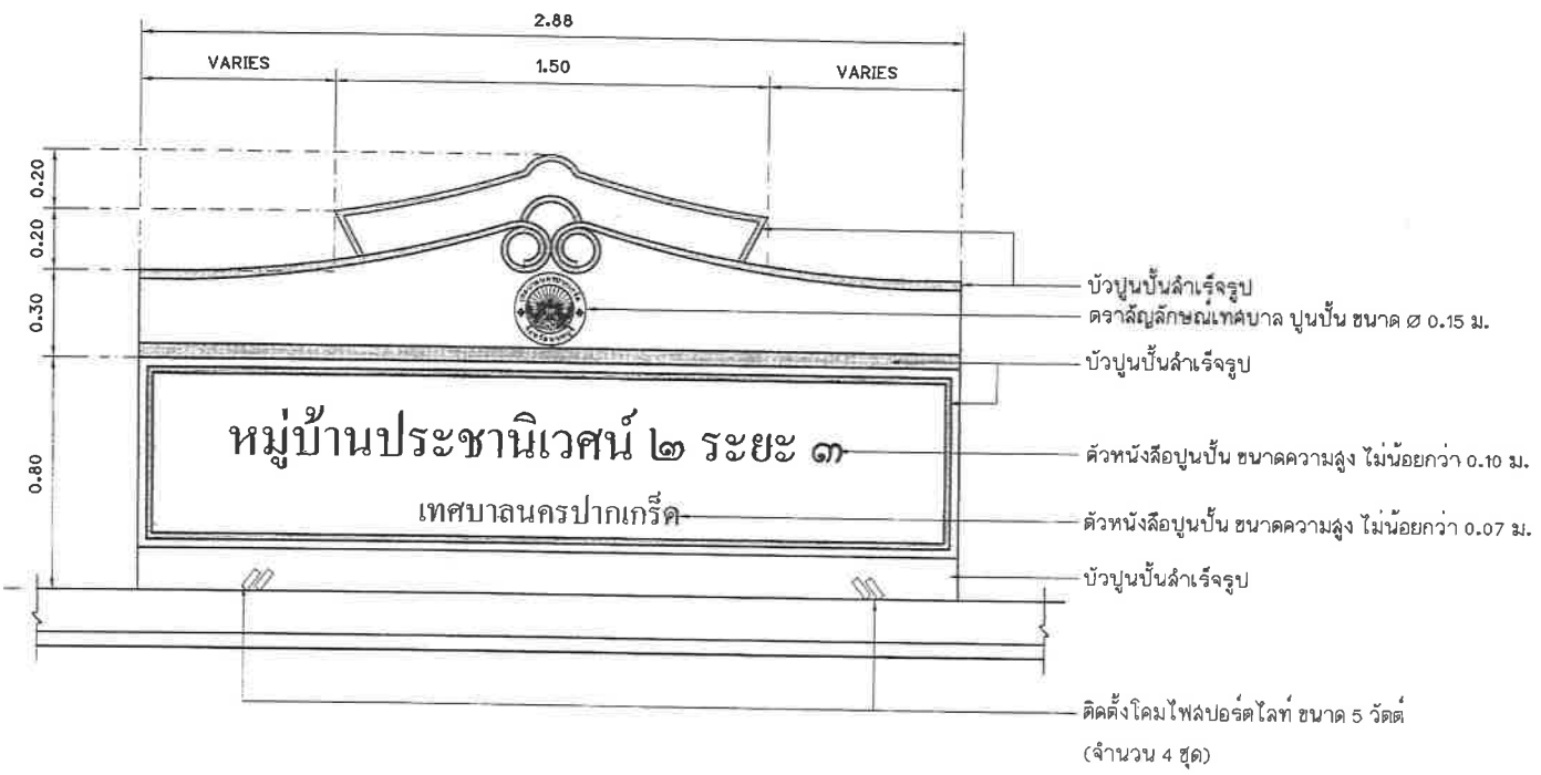
แบบขยายป้ายสะพาน คสล. (สะพานที่ 1) มาตราส่วน 1: 20
