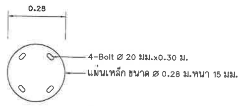
แบบขยายแปลนฐานเสาไฟอลูมิเนียม มาตราส่วน 1 : 10
