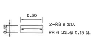
แบบขยายเสา CX-1 มาตราส่วน 1:20
