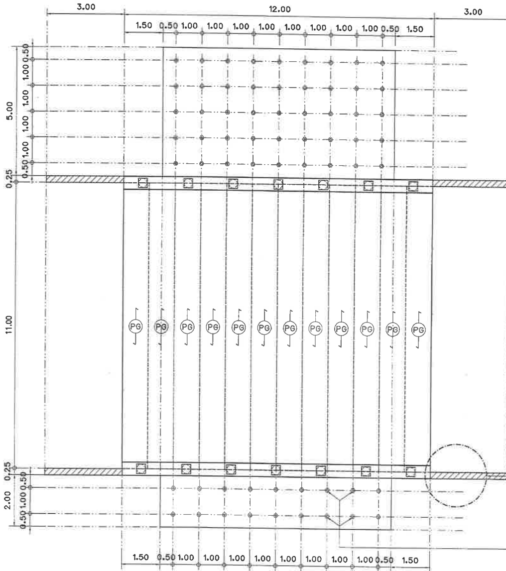
แปลนโครงสร้างสะพาน คสล. (สะพานที่ 1) มาตราส่วน 1:100
