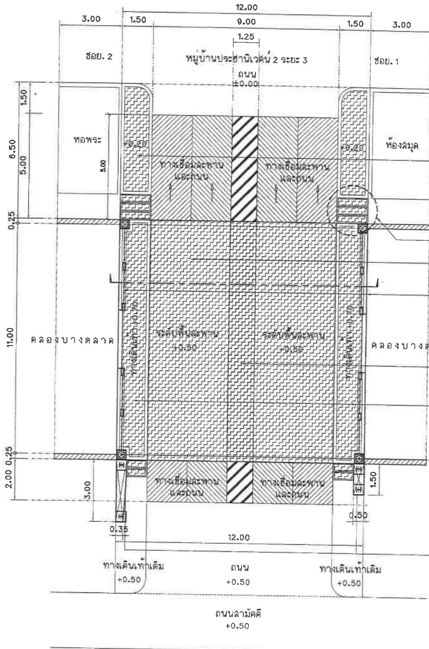
แปลนสะพาน คสล. (สะพานที่ 1) ขนาดจาล้วน 1:125
