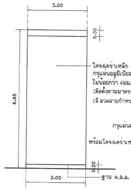
รูปด้าน 2 (ขาซุ้มฝั่งซ้าย) มาตราส่วน 1:75
