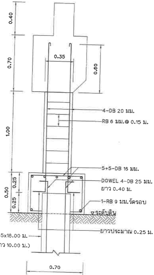
รูปตัดเสา C1 มาตราส่วน 1:20
