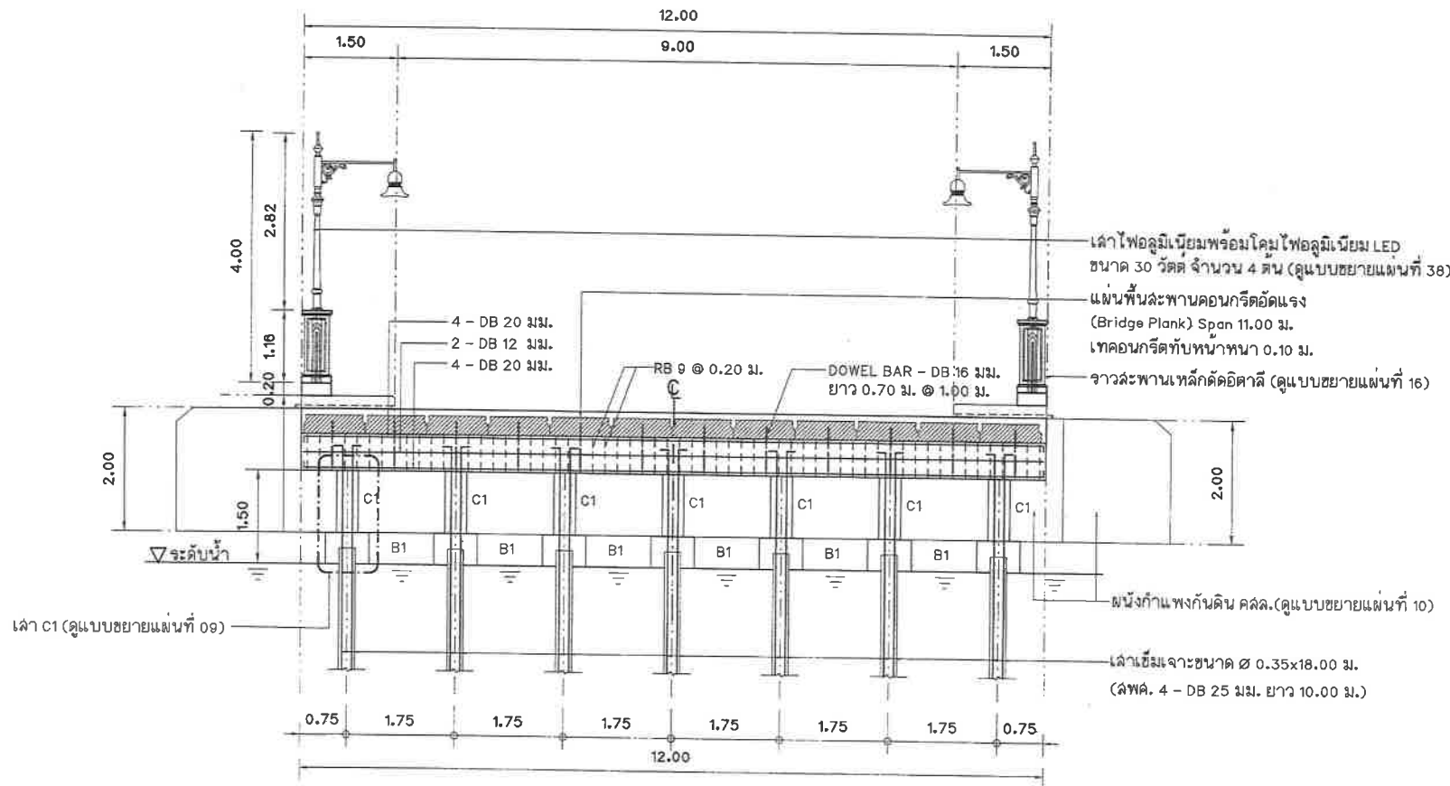
รูปตัดโครงสร้าง A - A (สะพานที่ 1) มาตราส่วน 1:75
