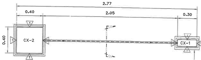
แบบขยายแปลนโครงสร้างราวสะพาน คสล. (สะพานที่ 2)
