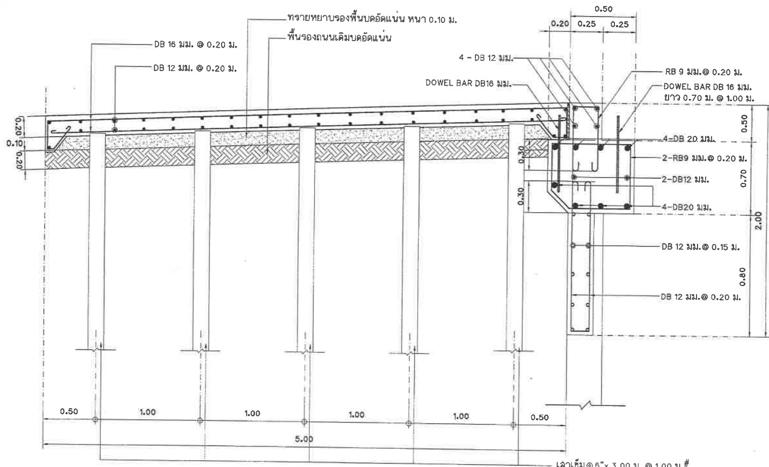
รูปตัดการเชื่อมสะพาน และผิวถนน คสล. (ฝั่งหมู่บ้านประชาชนิเวณ 2 ระยะ 3 )
