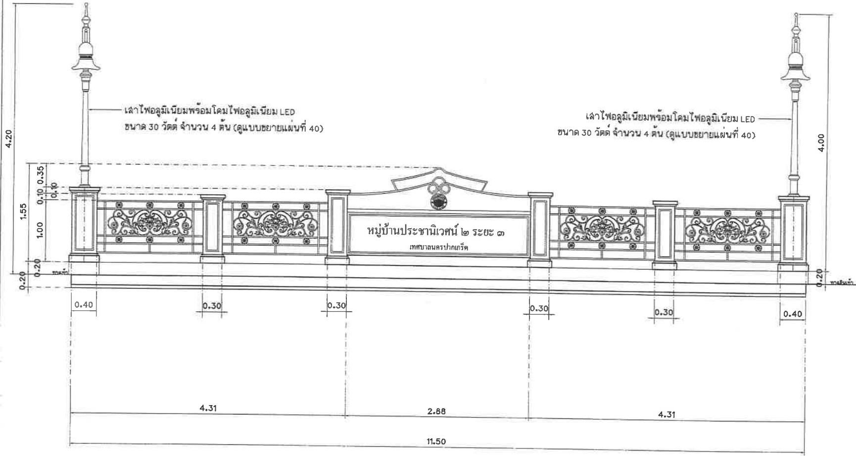
รูปด้านหน้าราวสะพาน คสล.พร้อมป้าย (สะพานที่ 1) มาตรฐาน 1 : 40
