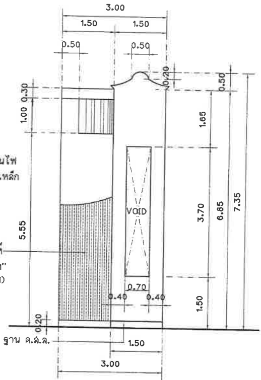
รูปด้าน 3 (ขาซุ้มฝั่งขวา) มาตราส่วน 1:75
