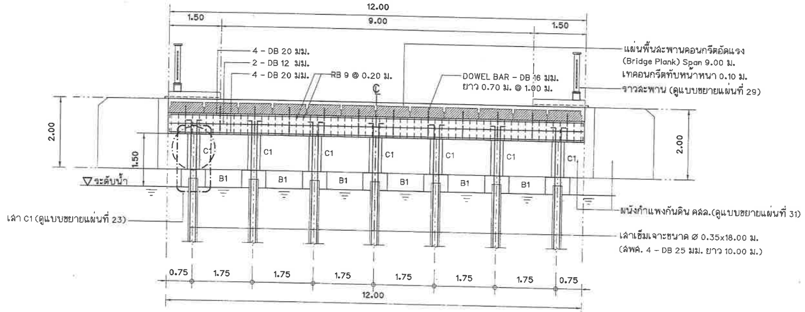
รูปตัดโครงสร้าง A - A (สะพานที่ 2) มาตราส่วน 1:75
