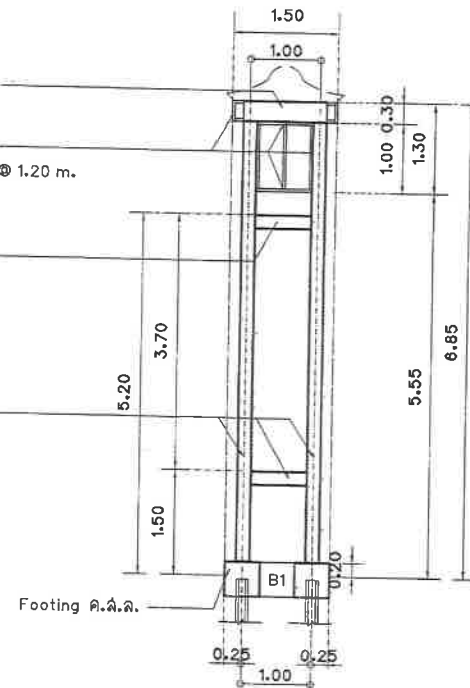
รูปตัดโครงสร้างเหล็ก B มาตราส่วน 1:75
