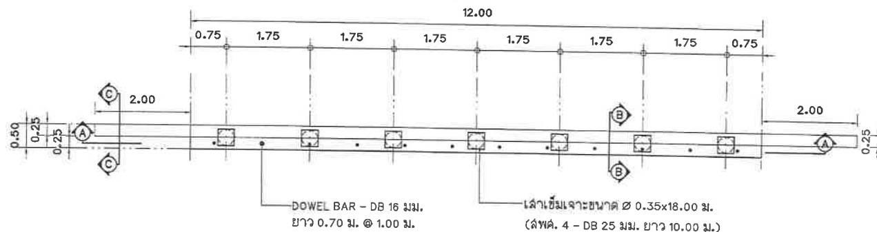
ขยายโครงสร้างสะพาน (สะพานที่ 1) มาตราส่วน 1:75
