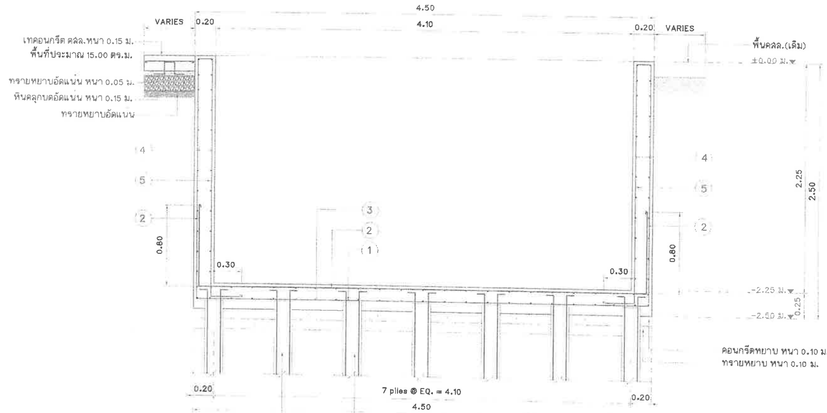
รูปตัดหลักเสาริมาดาดห้องคลอง คสล. ① มาตราส่วน 1:25
