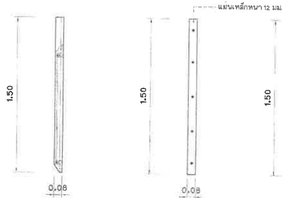
แบบขยายเหล็กเสริม มาตราส่วน 1 : 25
