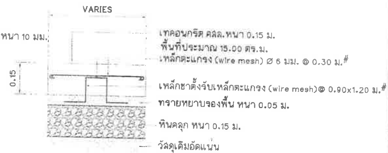
คอนกรีต คสล.หนา 0.15 ม. มาตราส่วน 1 : 10
