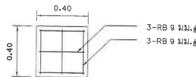
แบบขยายฐานเล้า CX-2
