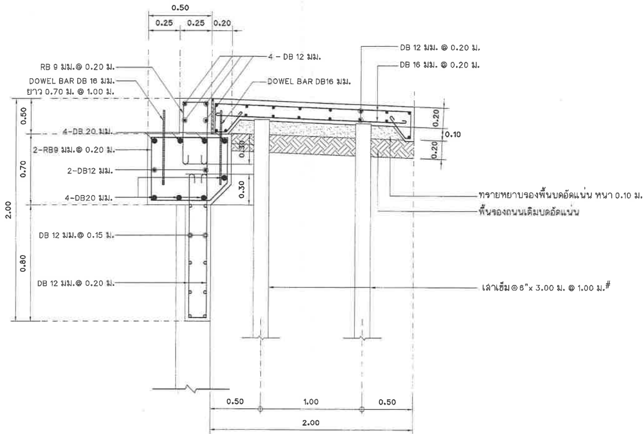
รูปตัดการเชื่อมสะพาน และพัวถน คสล. (ฝั่งถนนลำผักคี่)
