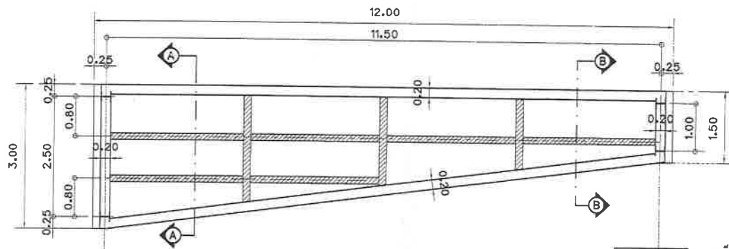
โครงสร้างเหล็กหลังคา มาตราส่วน 1 : 75
