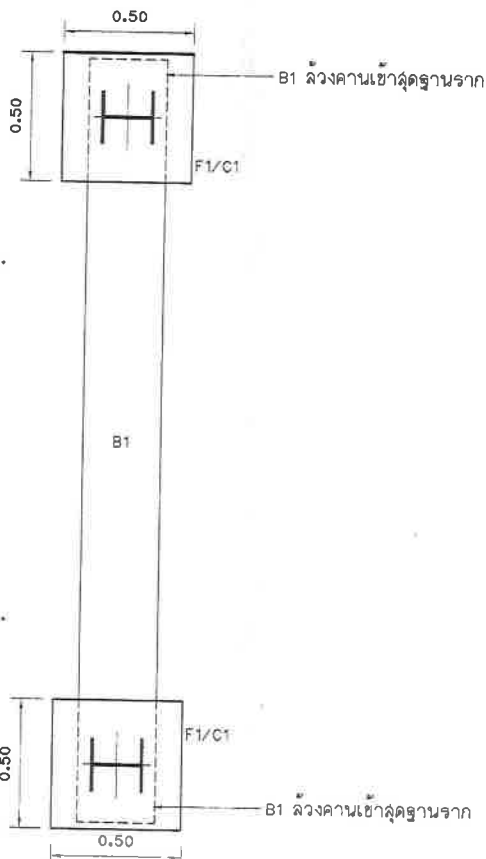
แปลนขยาย B1 (ฐานขาเข็มทางเข้าฝั่งซ้าย)
