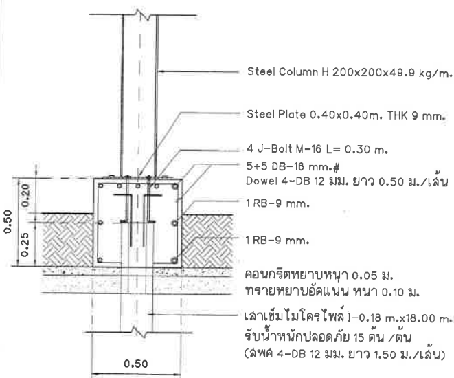
รูปตัดฐานราก F1
