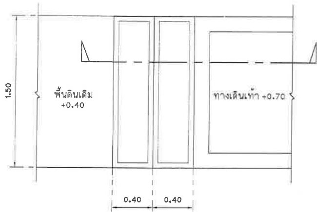
แบบขยายแปลนบันได ST1 (สะพานที่ 2)
