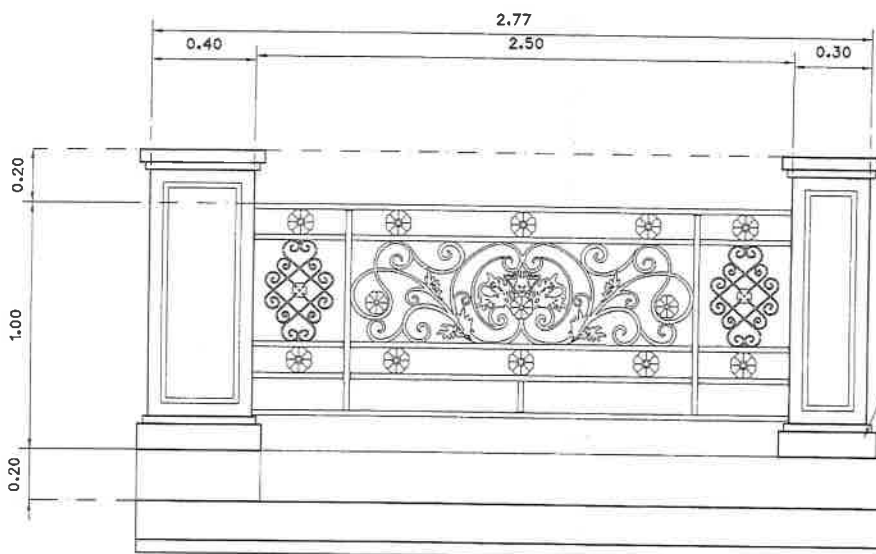
แบบขยายรูปด้านหน้าราวสะพานเหล็กดัดอิตาลี (สะพานที่ 2)
