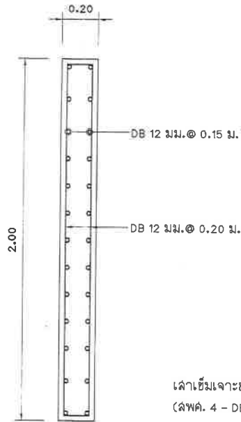
รูปตัดโครงสร้าง C - C (สะพานที่ 2)
