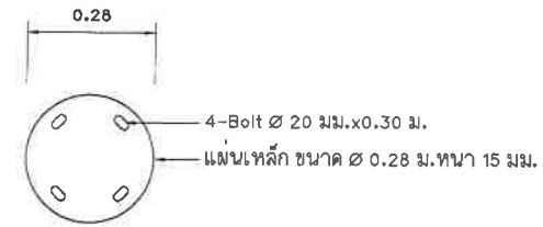
แบบขยายแปลนฐานเสาไฟอลูมิเนียม มาตราส่วน 1 : 10
