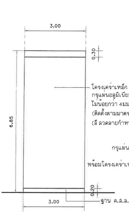
รูปด้าน 2 (ขาซุ้มฝั่งซ้าย) มาตราส่วน 1 : 75
