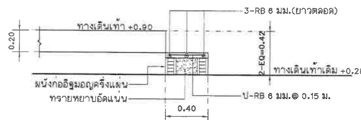
แบบขยายรูปตัดบันได ST2 (สะพานที่ 2)
