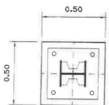
แปลนฐานราก F1
