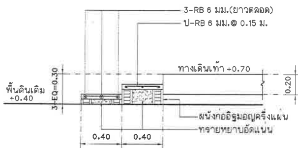
แบบขยายรูปตัดบันได ST1 (สะพานที่ 2)
