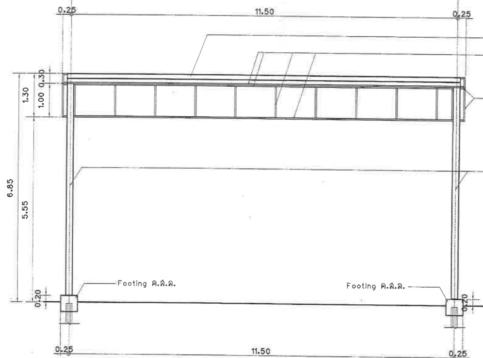
รูปดํานโครงสร้างเหล็กรูปพรรณ มาตราส่วน 1 : 75
