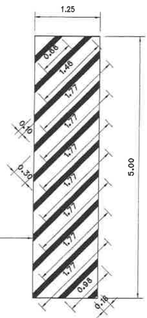
แบบขยายตีเส้นจราจรทางเชื่อมสะพาน และถนน คสล. มาตราส่วน 1:50
