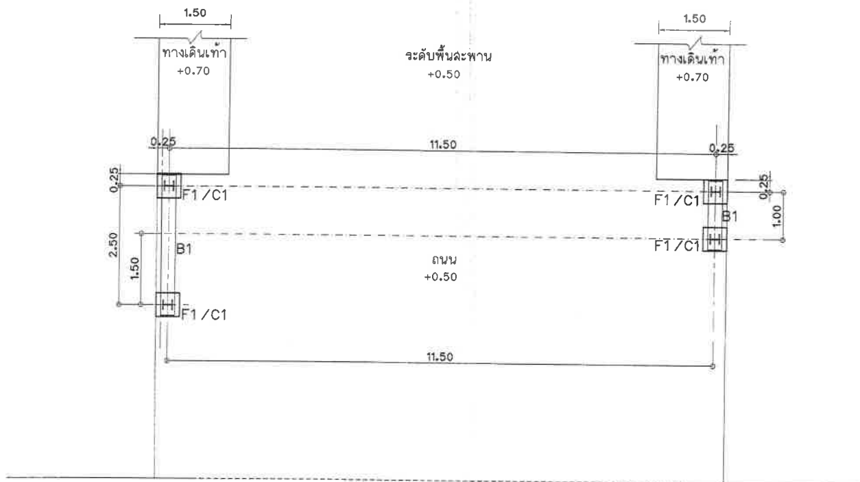
ผังฐานราก F1/C1 มาตราส่วน 1:75
