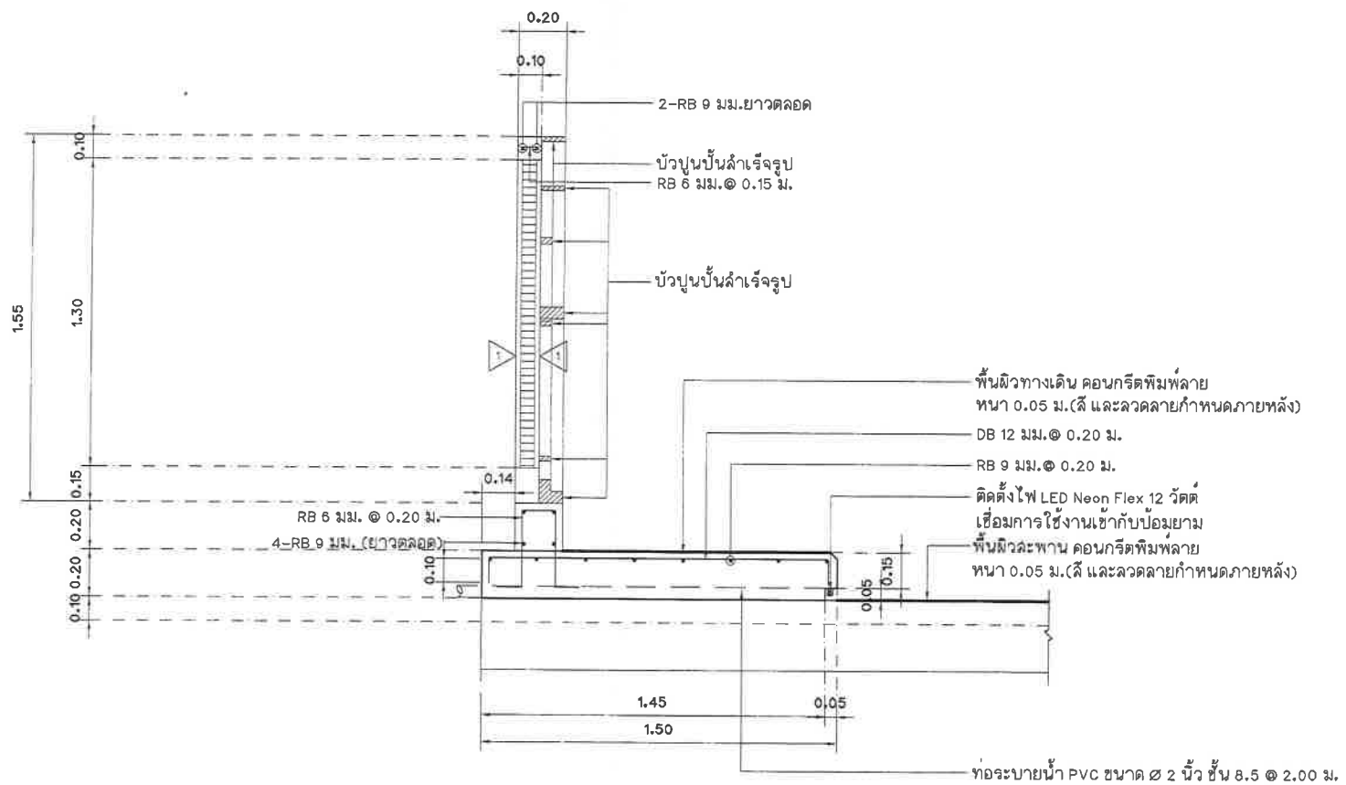
แบบขยายรูปตัดโครงสร้างป้ายสะพาน คสล. พื้นทางเท้า มาตราส่วน 1:20
