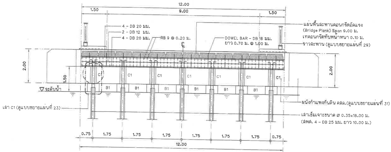
รูปตัดโครงสร้าง A - A (สะพานที่ 2) มาตรฐาน 1:75
