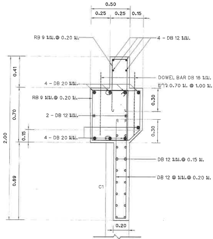
รูปตัดโครงสร้าง B - B (สะพานที่ 2)
