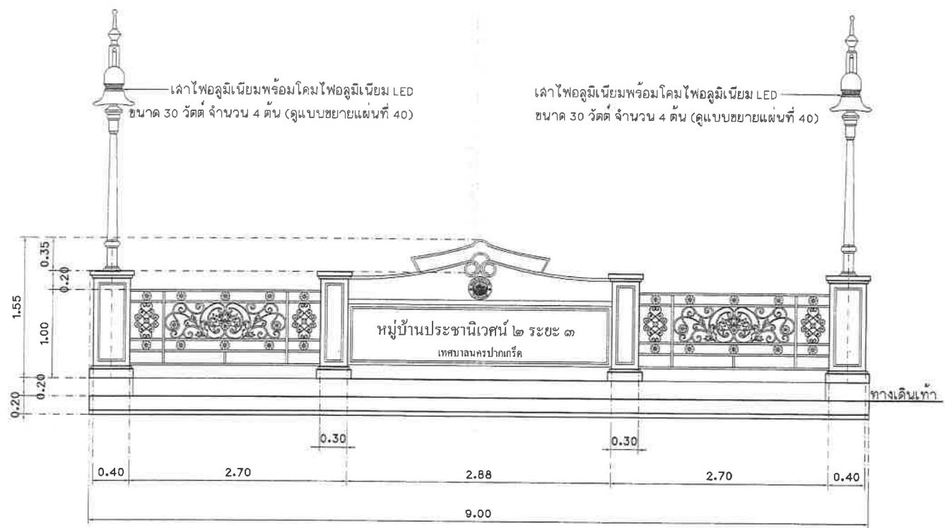
รูปด้านหน้าราวสะพาน คสล.พร้อมป้าย (สะพานที่ 2) มาตรฐาน 1:40
