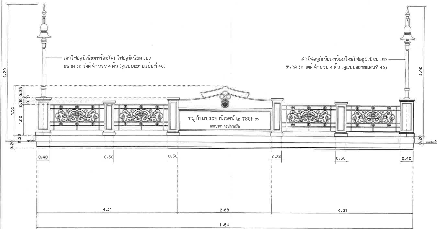
รูปด้านหน้าราวสะพาน คสล.พร้อมป้าย (สะพานที่ 1) มาตราส่วน 1:40
