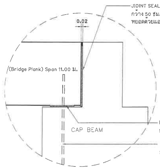
แบบขยาย CAP BEAM มาตราส่วน 1:10
