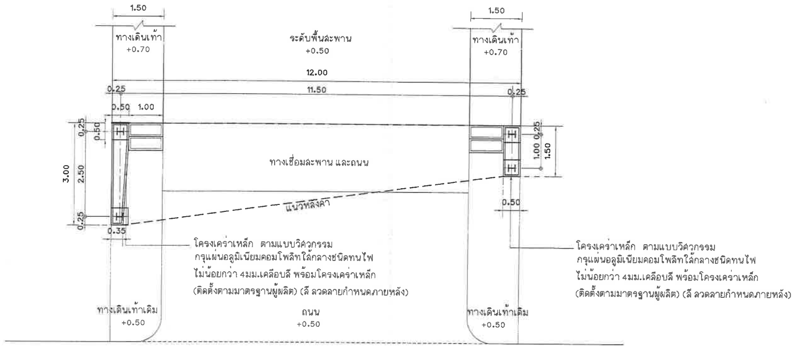
แปลนซุ้มทางเข้าหมู่บ้าน มาตราส่วน 1 : 75
