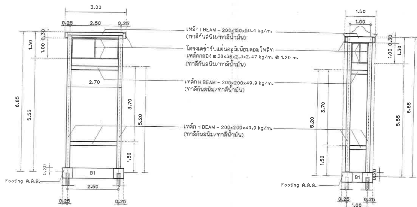
รูปตัดโครงสร้างเหล็ก A มาตราส่วน 1:75
