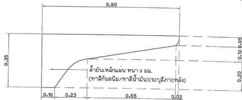
แบบขยายแผ่นเหล็กค้ำยันระยะความกว้างหลังคาค 2.00 เมตร
