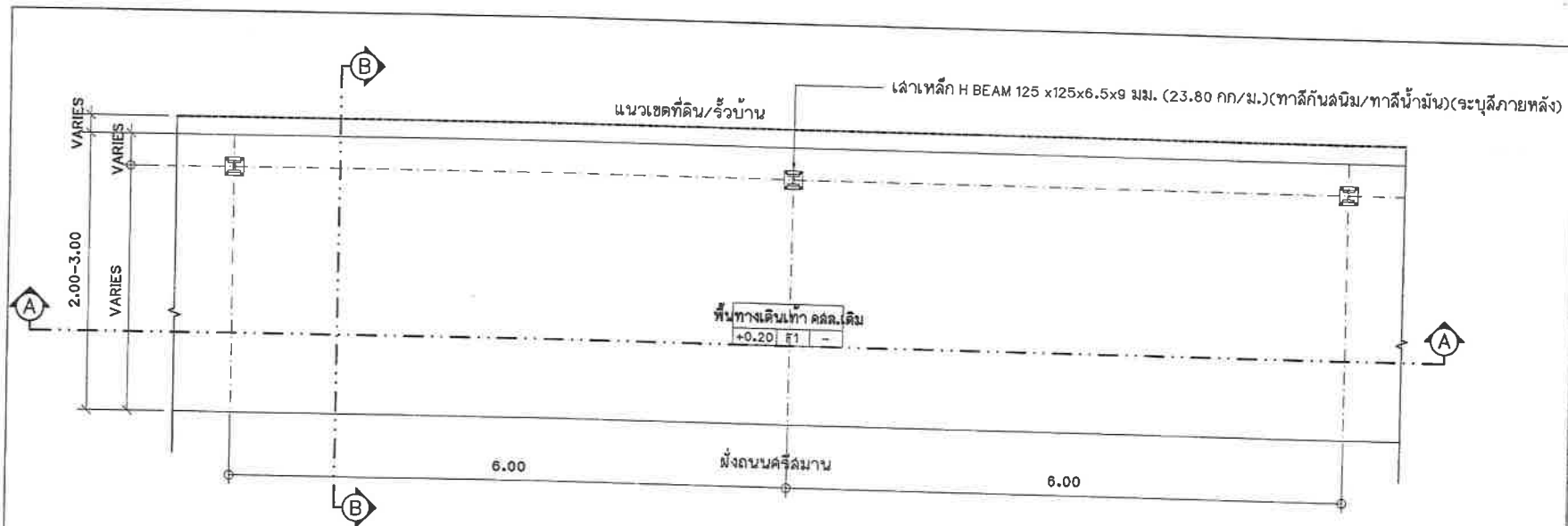
แปลนพื้นทางเดินคสล.ระยะทางระหว่างเสา 6.00 เมตร มาตราส่วน 1:50
