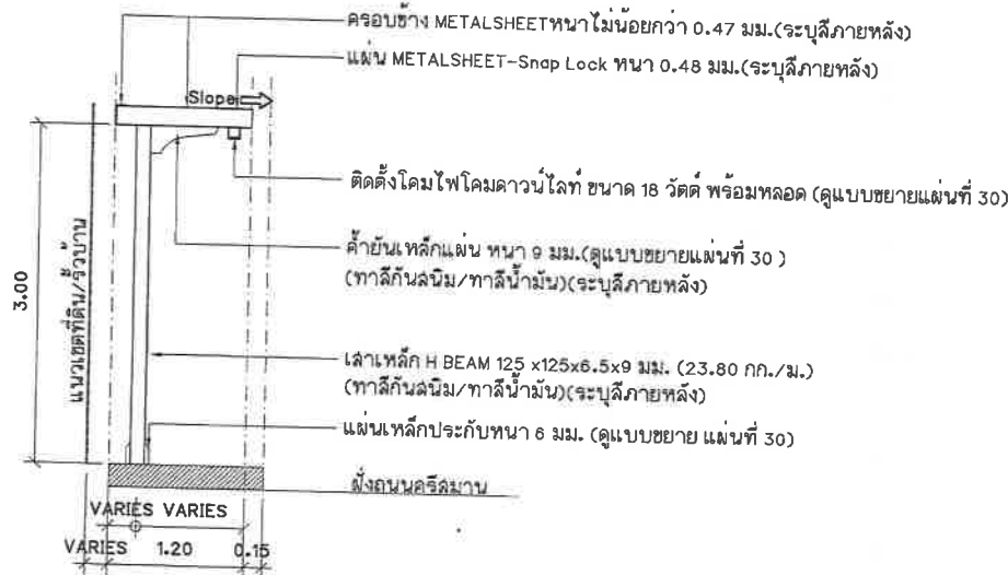
รูปด้านระยะหลังคากว้าง 1.20 เมตร
