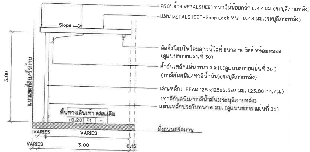
รูปด้านระยะหลังคากว้าง 3.00 เมตร
