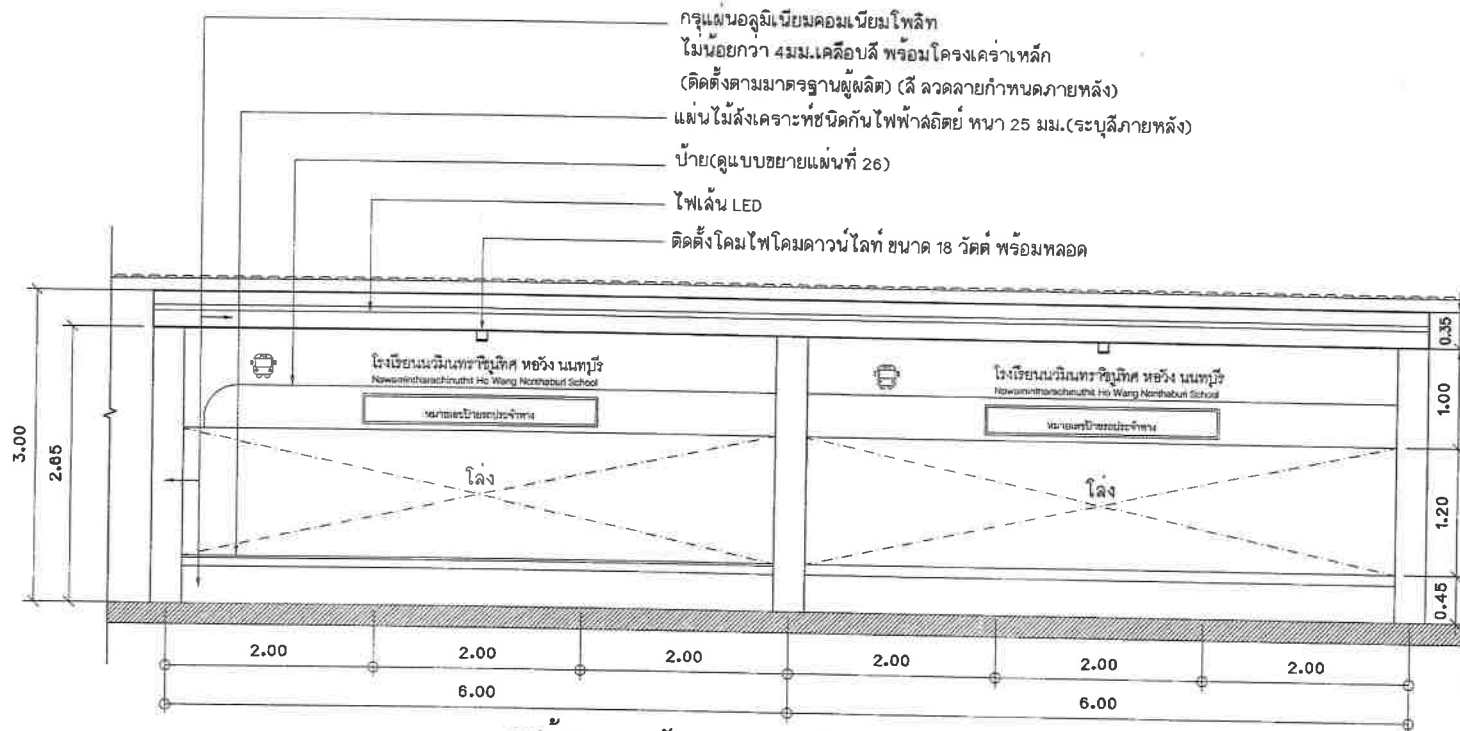
รูปด้าน 1 จุดพักคอยรถประจำทาง
