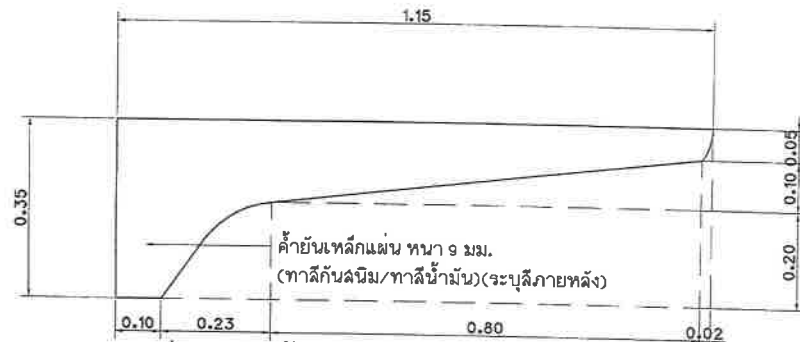
แบบขยายแผ่นเหล็กค้ำยันระยะความกว้างหลังคาค 3.00 เมตร
