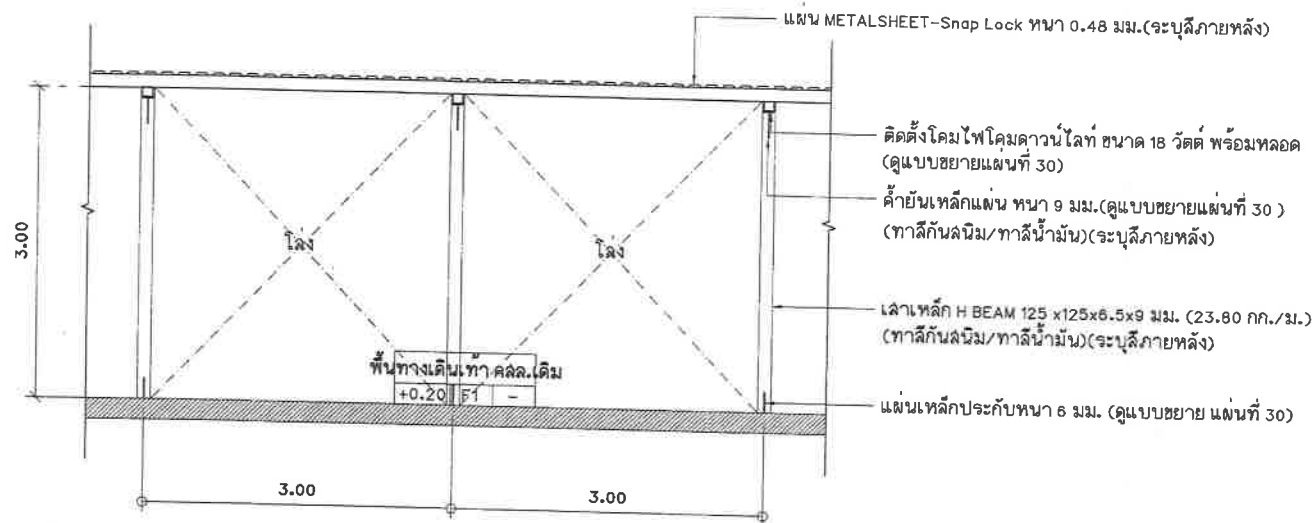
รูปด้านปรับปรุงหลังคาทั้งหลังคลุมทางเดินระยะห่างระหว่างเสา 3.00 เมตร
