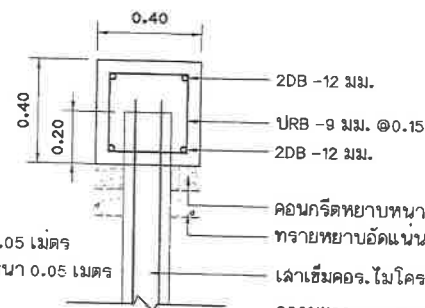
แบบขยายรูปตัดฐานราก 2 มาตราส่วน 1 : 20
