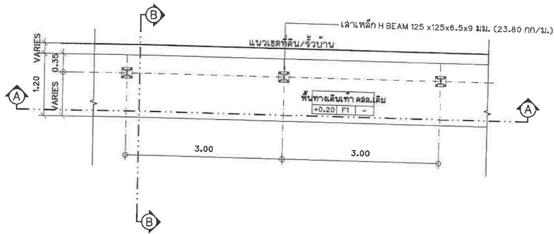
แปลนพื้นที่เดินเท้า คสล.เดิม ระยะห่างระหว่างเสา 3.00 เมตร มาตราส่วน 1:50
