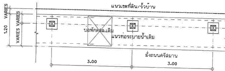
แปลนฐานรากคูลล์.แบบที่ 3
