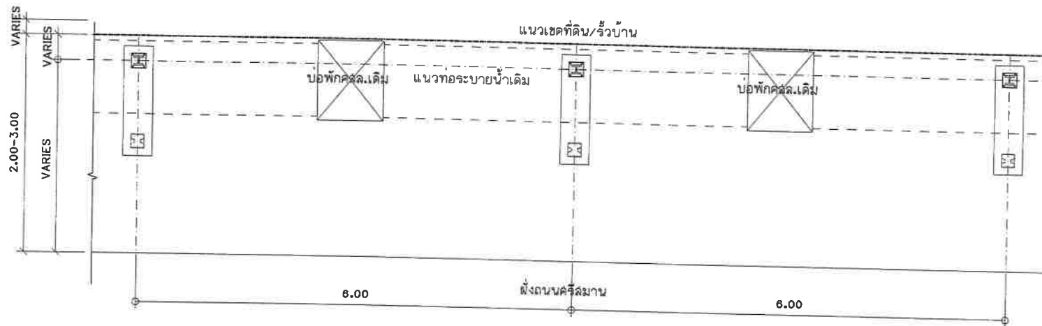
แปลนฐานรากคสล.แบบที่ 2
