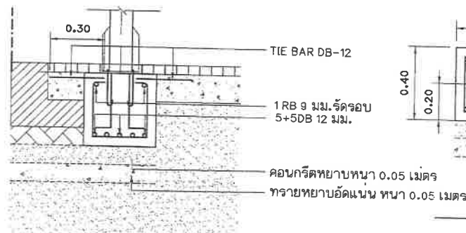
แบบขยายรูปตัดฐานราก 3 มาตราส่วน 1 : 20
