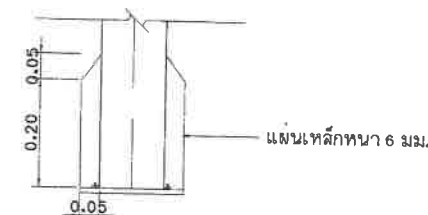
แบบขยายการยึดเสาเหล็ก
