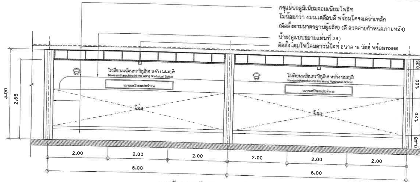
รูปตัด 1 จุดพักคอยรถประจำทาง
