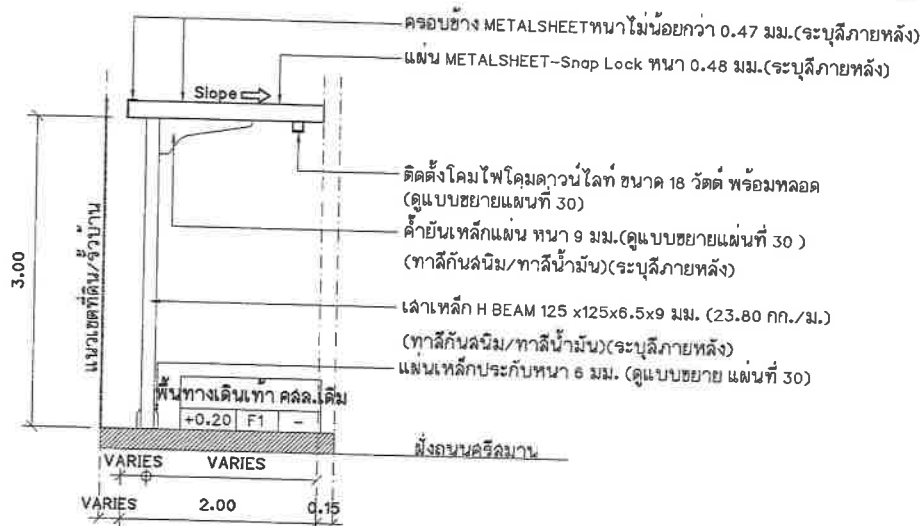
รูปด้านระยะหลังคากว้าง 2.00 เมตร
