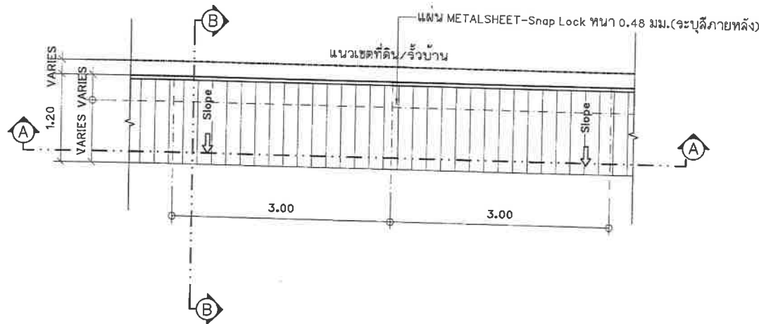
แปลนปรับปรุงหลังคากันลัดคลุมทางเดิน ระยะห่างระหว่างเสา 3.00 เมตร มาตราส่วน 1:50
