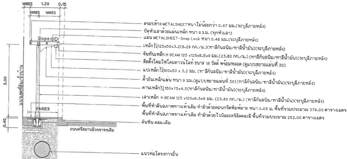
รูปตัดขยาย 3
