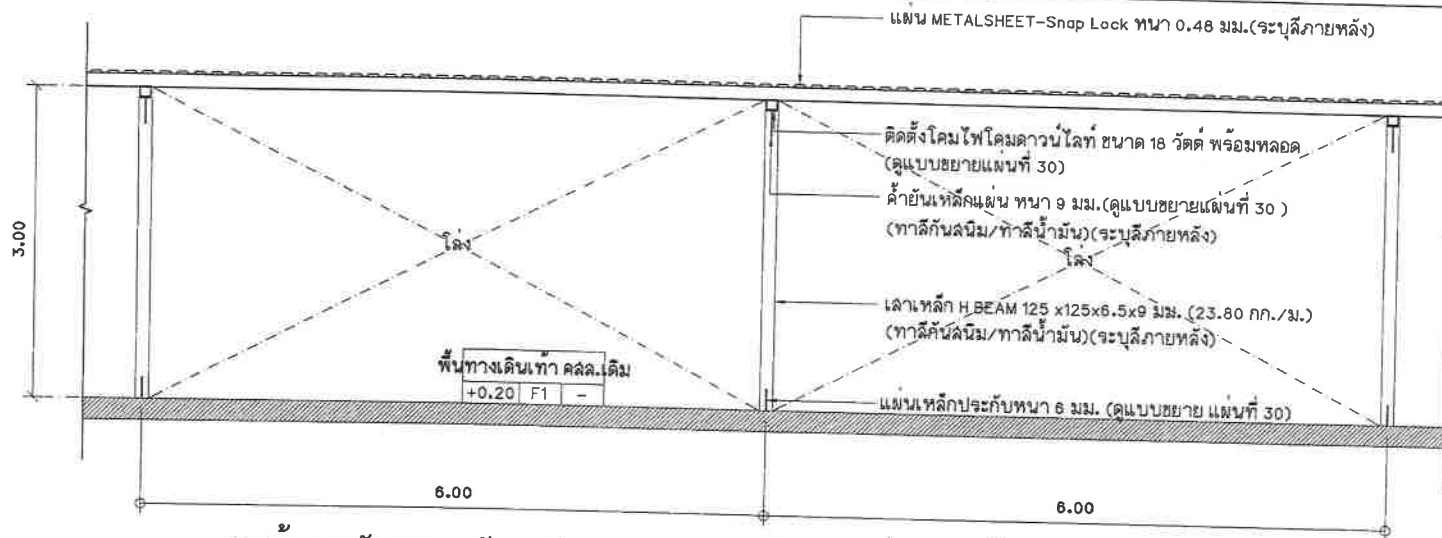
รูปด้านปรับปรุงหลังคาหลังคาคลุมทางเดินระยะห่างระหว่างเสา 6.00 เมตร มาตราส่วน 1 : 50
