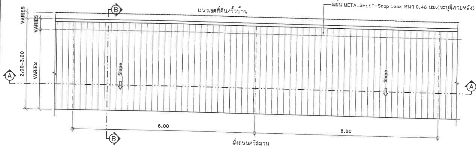
แปลนปรับปรุงหลังคากันลวดคลุมทางเดินระยะทางระหว่างเสา 6.00 เมตร มาตราส่วน 1:50
