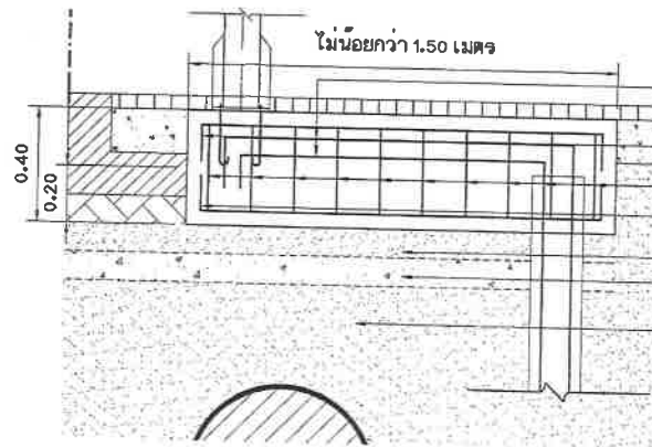
แบบขยายรูปตัดฐานราก 2 มาตราส่วน 1 : 20
