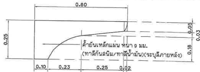
แบบขยายแผ่นเหล็กค้ำยันระยะความกว้างหลังคาค 1.20 เมตร
