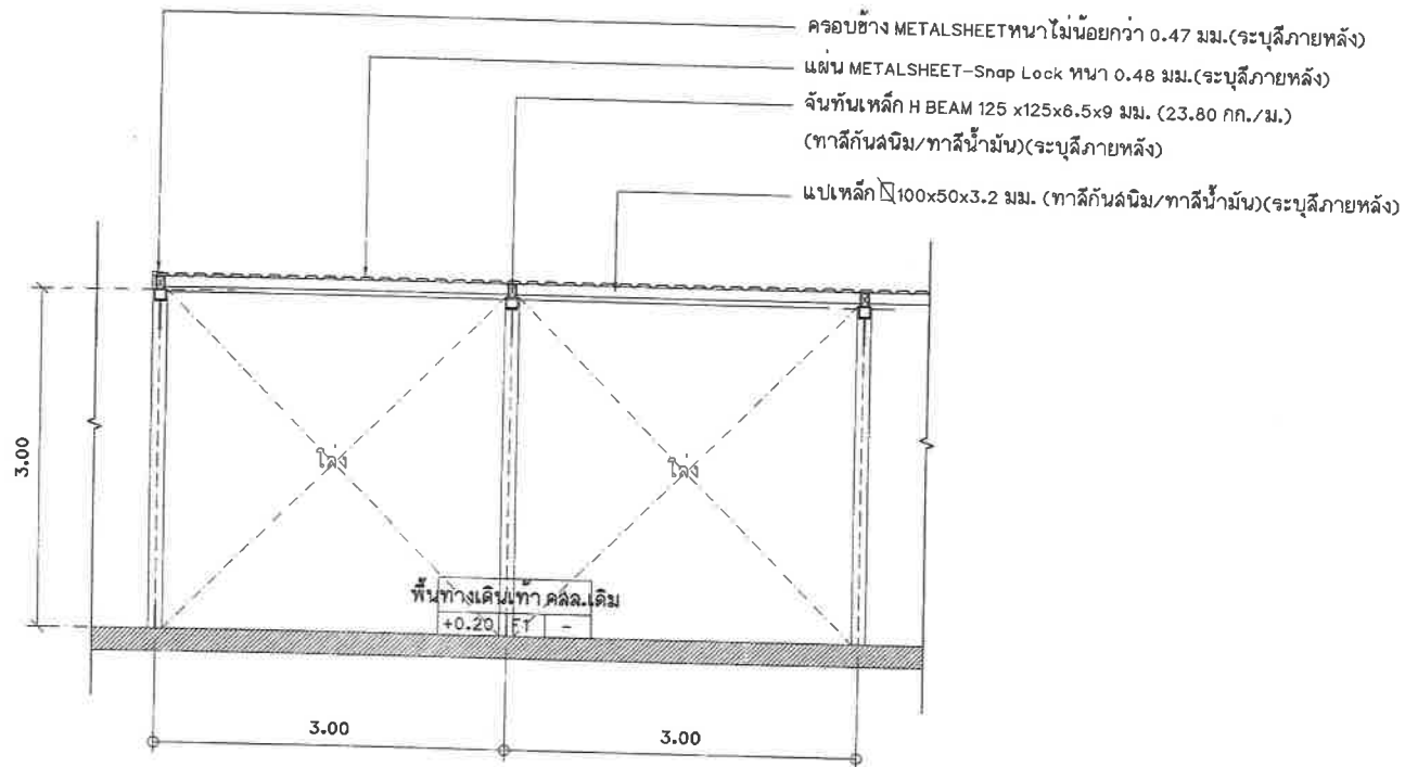
รูปตัดปรับปรุงหลังคากันลาดคลุมทางเดินระยะทางระหว่างเสา 3.00 เมตร มาตราส่วน 1 : 50
