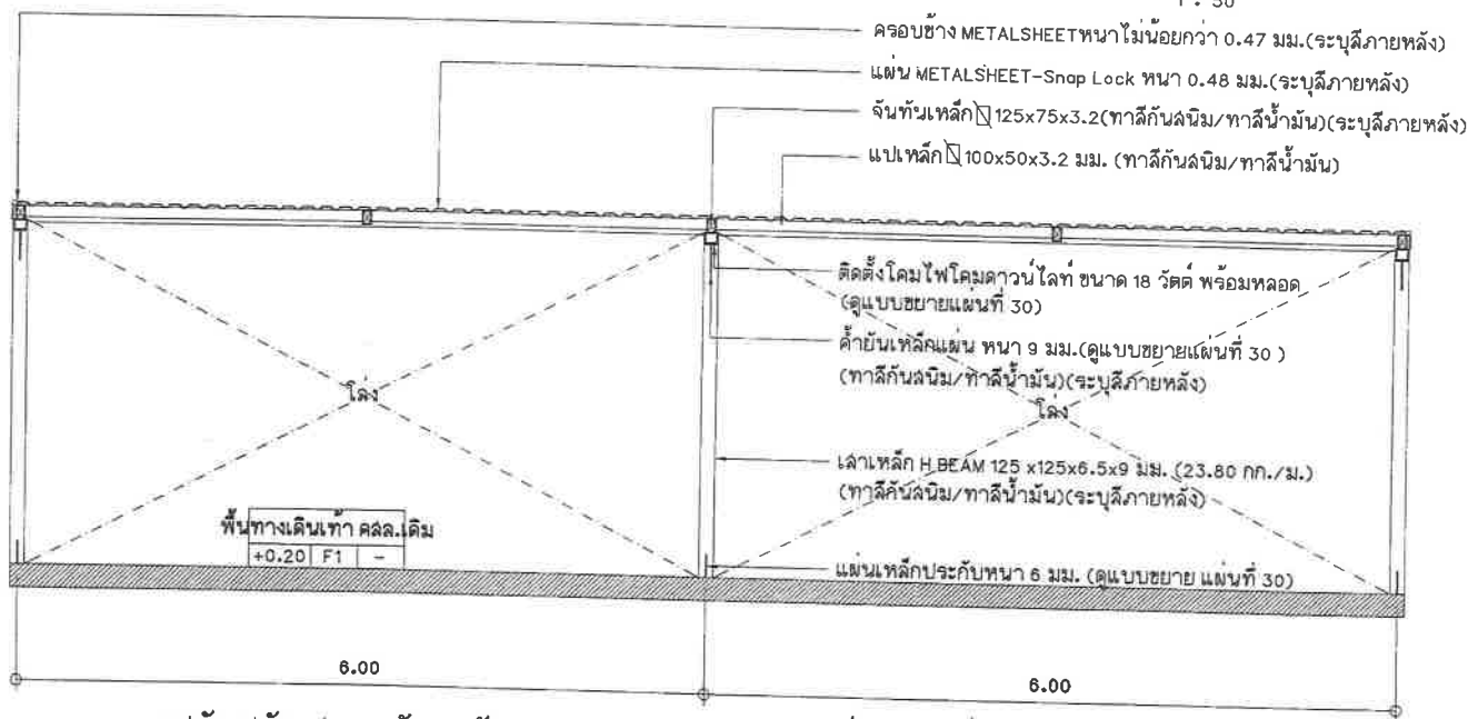
รูปตัดปรับปรุงหลังคาหลังคาคลุมทางเดินระยะห่างระหว่างเสา 6.00 เมตร มาตราส่วน 1 : 50
