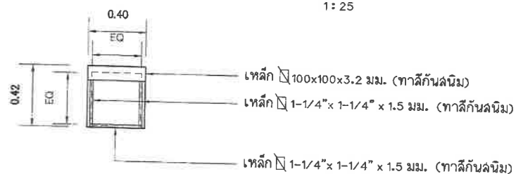
แบบขยายโครงลั้างป้ายจุดพัคคอยรลประจำทาง/กรุที่นั้งพัคคอย มาตราลั้วน 1: 25
