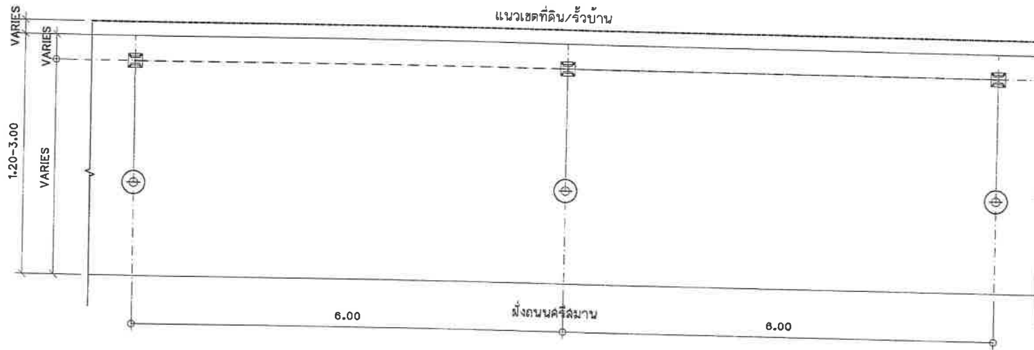
แปลนไฟฟ้าทางเดินคสล.ระยะห่างระหว่างเสา 6.00 เมตร มาตราส่วน 1:50
