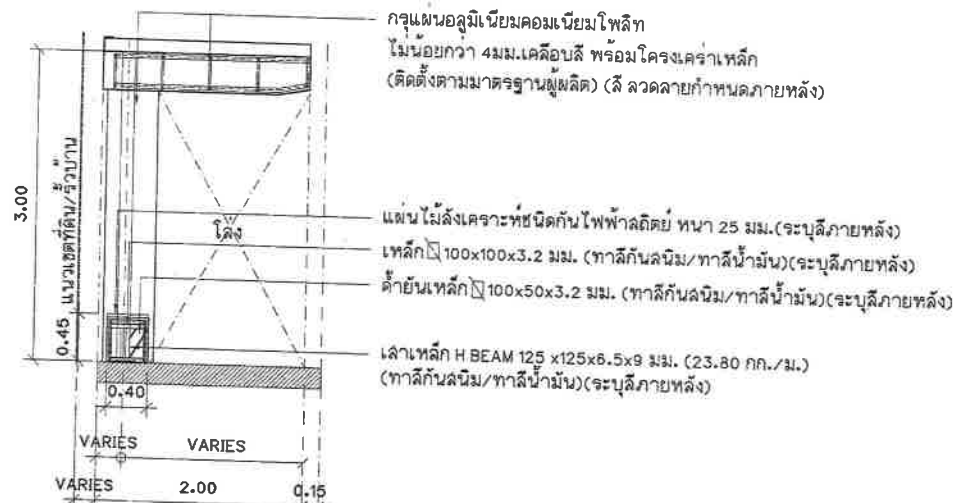
รูปตัด 2 จุดพักคอยรถประจำทาง
