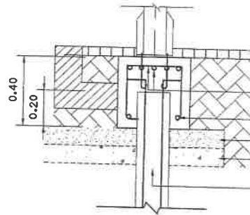
แบบขยายรูปตัดฐานราก 1 มาตราส่วน 1 : 20
