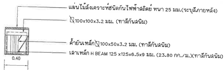
แบบขยายโครงลั้างป้ายจุดพัคคอยรลประจำทาง/กรุที่นั้งพัคคอย มาตราลั้วน 1: 25
