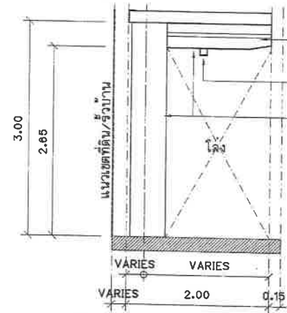
รูปด้าน 2 จุดพักคอยรถประจำทาง
