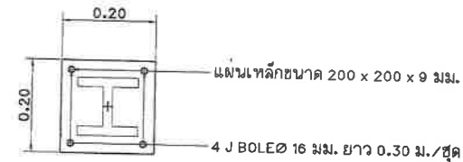
แบบแผ่นเหล็กยึดเสา
