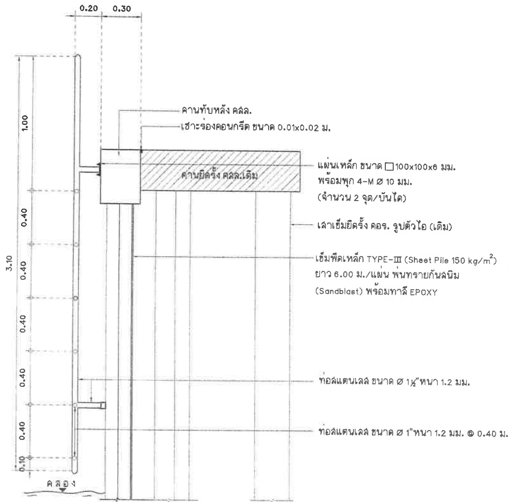
รูปตัด ด้านข้างบันไดสแตนเลส มาตราส่วน 1 : 20
