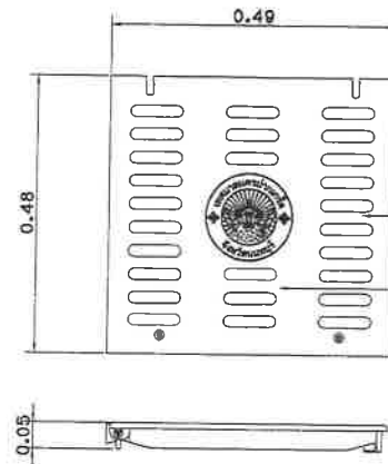
แบบขยายฝารางระบายน้ำเหล็กหล่อเหนียว
