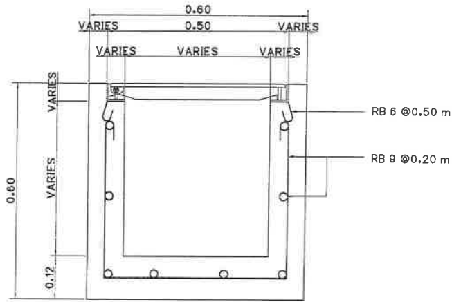
ขยายรูปตัดวางระบายน้ำ คสล.
