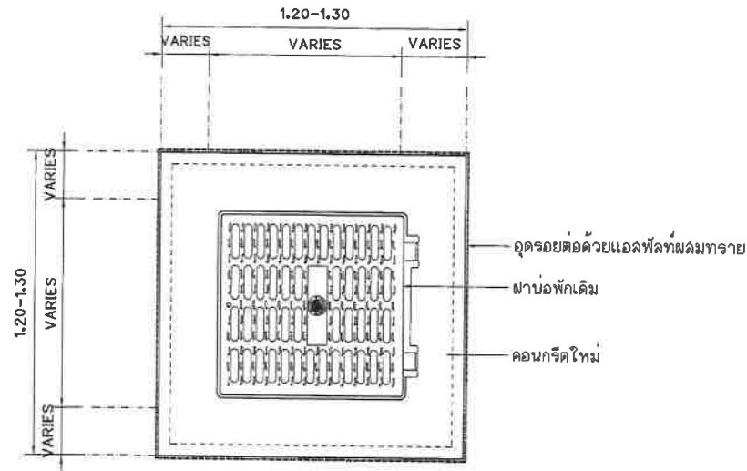
แบบขยายฝาบ่อพัก ค.ล.ล.ของเดิม (เสริมระดับปากบ่อใหม่ แบบฝาเรียบ)
