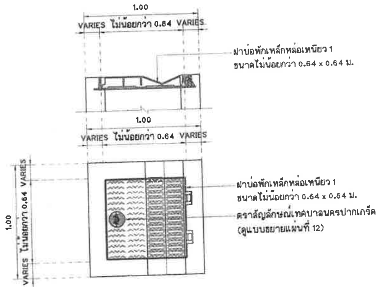
แบบขยายตู้บล็อกลูกข่าย 1 มาตราส่วน 1:20
