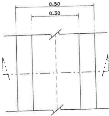
แบบขยายแปลนรางวี คสล. มาตรฐาน 1 : 10
