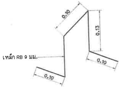
แบบขยายเหล็กขาตั้งรับเหล็กตะแกรง (ผิว คสล.หนา 0.15 ม.) มาตรฐาน 1 : 5
