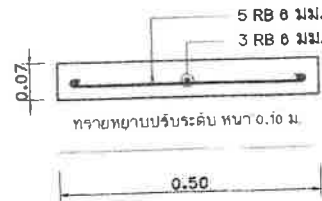
แบบขยายรูปตัดแผ่นพื้นรองท้อ มาตรฐาน 1 : 10
