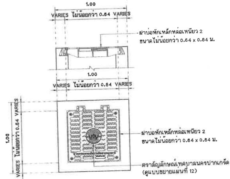
แบบขยายตู้บล็อกลูกข่าย 2 มาตราส่วน 1:20
