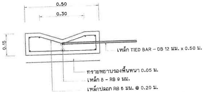
ขยายตัดรางวี คสล. มาตรฐาน 1 : 10
