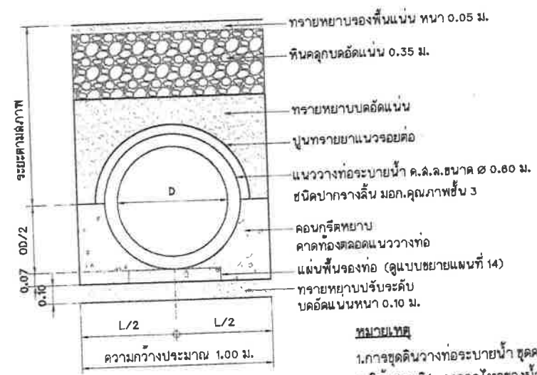
แบบขยายการวางท่อระบายน้ำ คสล. มาตราส่วน 1:20
