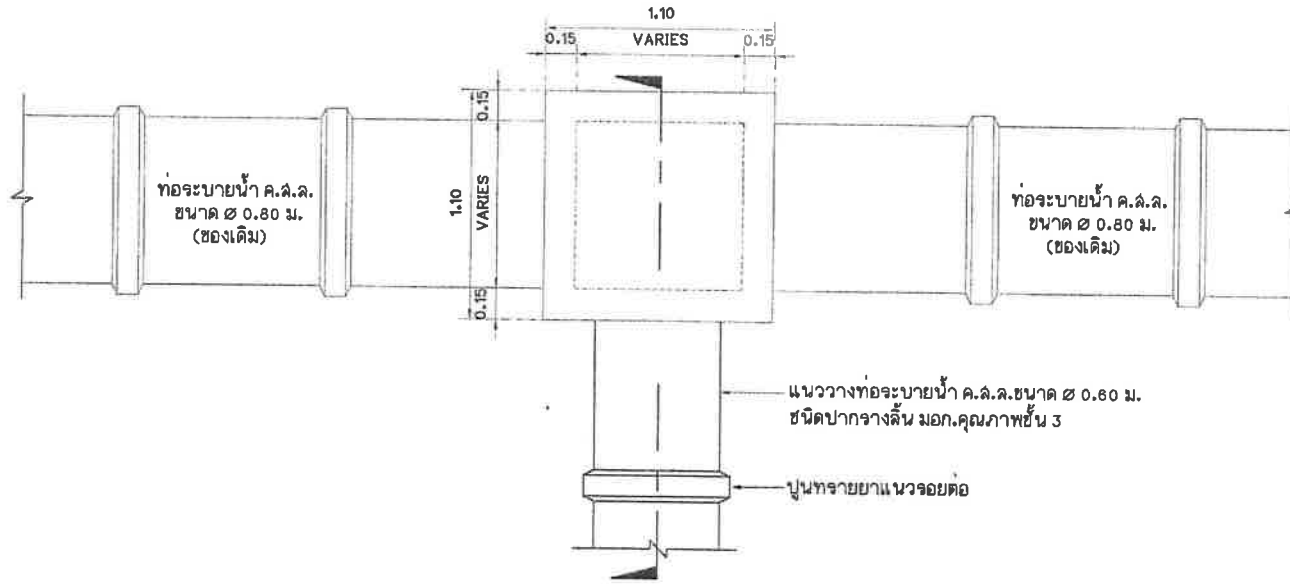
แปลนการเชื่อมต่อในกรณีเชื่อมกับท่อระบายน้ำของเดิม มาตราส่วน 1 : 25
