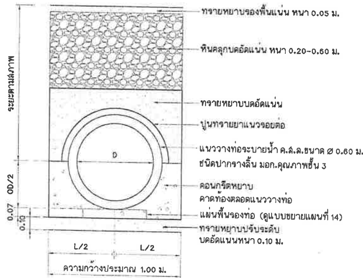
แบบขยายการวางท่อระบายน้ำ คสล. มาตราส่วน 1:20
