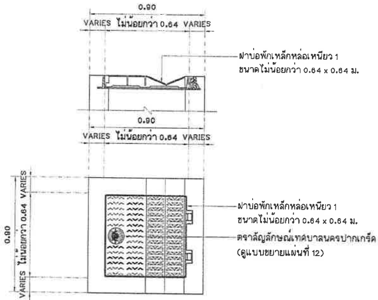
แบบขยายฝาบ่อพักเหล็กหล่อเหนียว 1 มาตราส่วน 1:20
