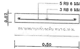
แบบขยายรูปตัดแผ่นพื้นรองท่อ มาตรฐาน 1 : 10
