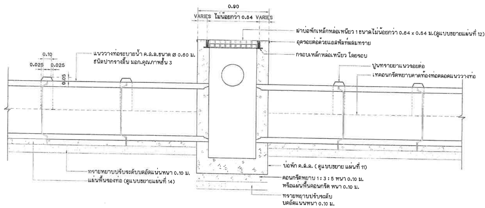
รูปตัดตามยาวการวางท่อระบายน้ำ มาตราล้วน 1:20
