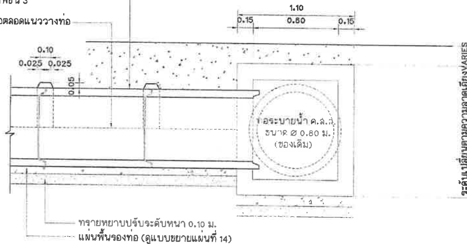
รูปตัดการเชื่อมต่อท่อระบายน้ำของเดิม มาตราส่วน 1 : 25
