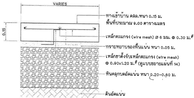
แบบขยายรูปตัดทางเข้าบ้าน คสล.หนา 0.15 ม. มาตรฐาน 1 : 10
