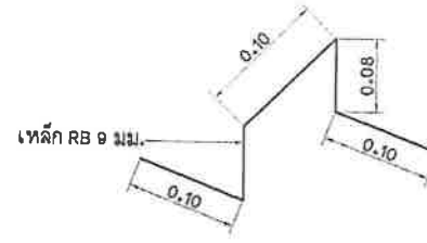
แบบขยายเหล็กขาตั้งรับเหล็ก (DOWEL BAR) มาตรฐาน 1 : 5
