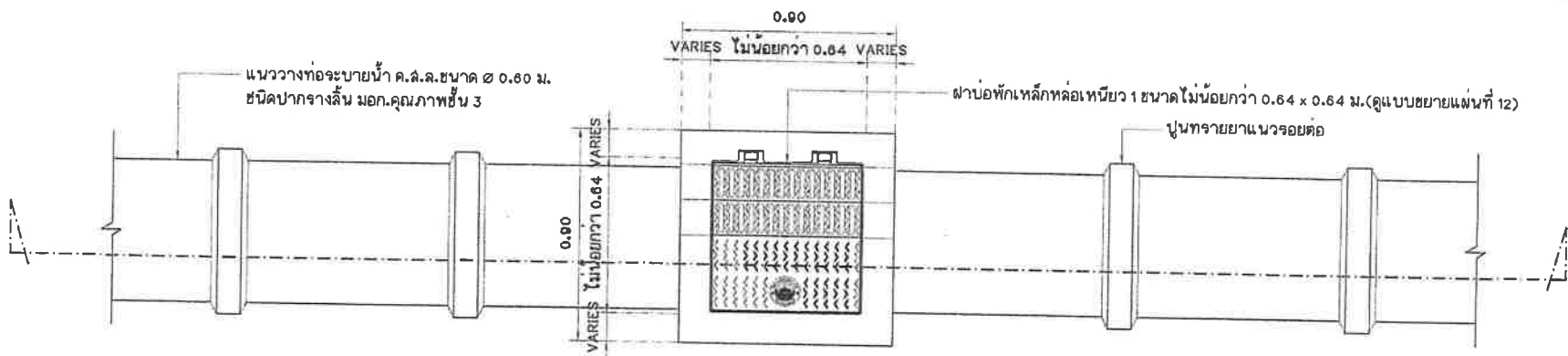
แปลนการวางท่อระบายน้ำ มาตราล้วน 1:20
