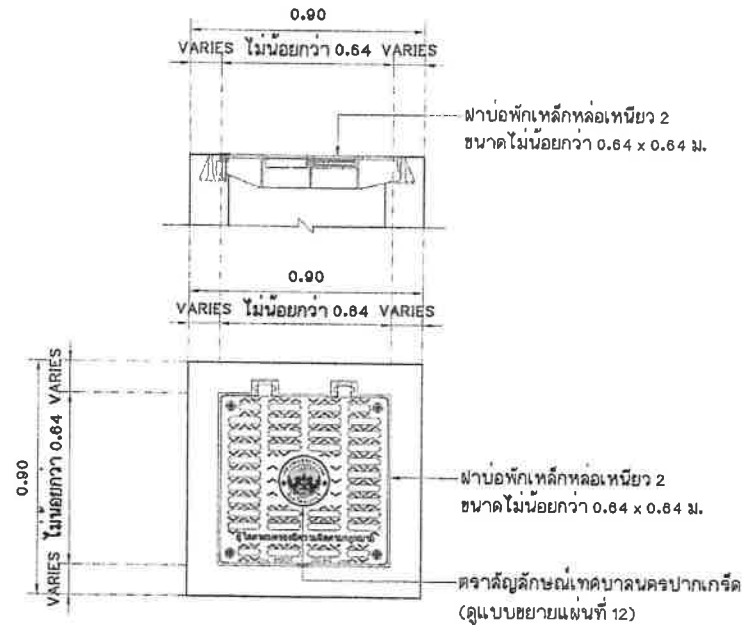
แบบขยายฝาบ่อพักเหล็กหล่อเหนียว 2 มาตราส่วน 1:20 (ฝาบ่อพัก และกรอบเป็นชนิดกันเสียงโดยเฉพาะ)
