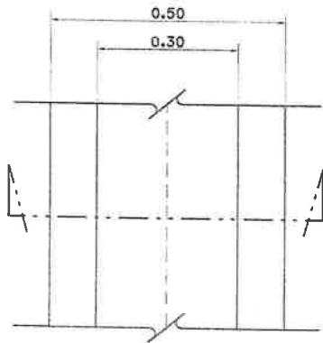
แบบขยายรูปตัดทางเข้าบ้าน คสล.หนา 0.15 ม. มาตรฐาน 1 : 10
