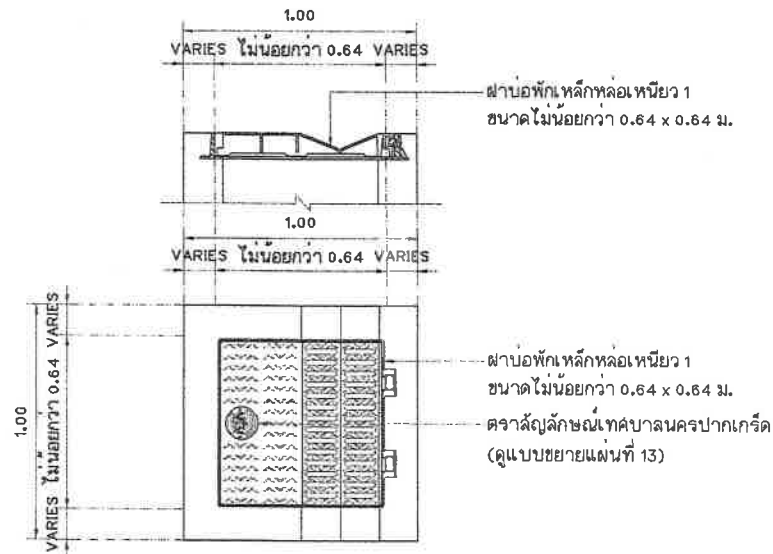
แบบขยายฝาบ่อพักเหล็กหล่อเหนียว 1
