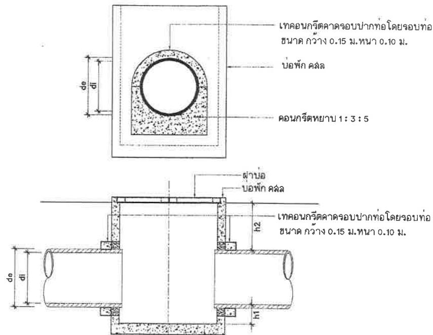
การประลันท่อ HDPE เข้าบ่อ คลัล.
