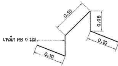
แบบขยายเหล็กขาตั้งรับเหล็ก (DOWEL BAR) มาตราส่วน 1 : 5
