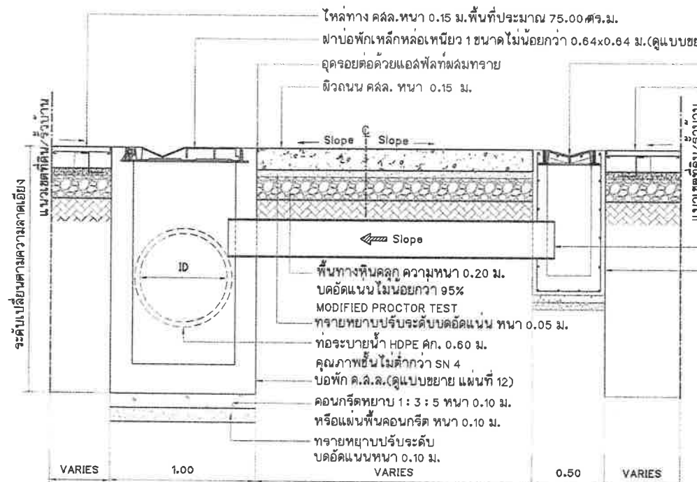
แบบขยายรูปตัด 2
