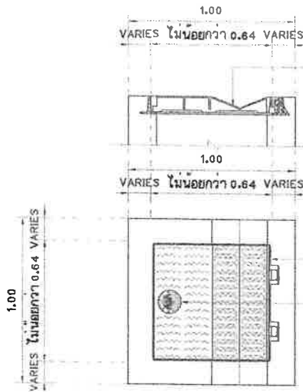
ฝาบ่อพักเหล็กหล่อเหนียว 1 ขนาดไม่น้อยกว่า 0.64 x 0.64 ม.
