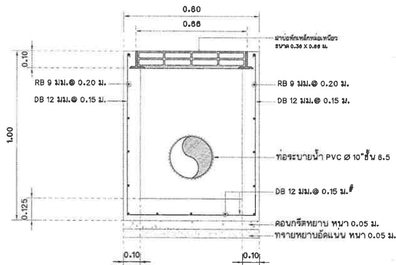
แบบขยายรูปตัด ② บ่อพักระบายน้ำ คลล. พร้อม ฝาบ่อพักรางวิเหล็กหล่อเหลี่ยม มาตราส่วน 1:15
