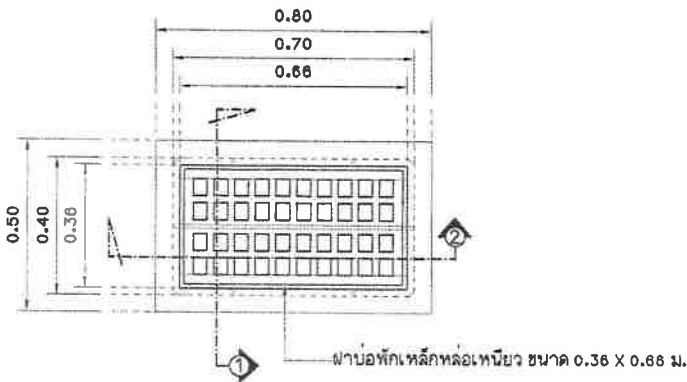
แบบขยายฝาบ่อพักรางวิเหล็กหล่อเหลี่ยม มาตราส่วน 1:15
