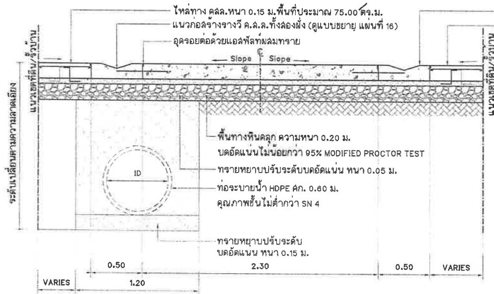
แบบขยายรูปตัด 1
