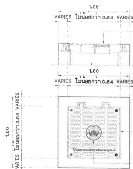
ฝาบ่อพักเหล็กหล่อเหนียว 2 ขนาดไม่น้อยกว่า 0.64 x 0.64 ม.
