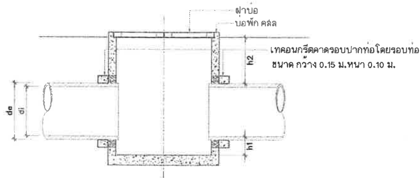
การประลันท่อ HDPE เข้าบ่อ คลล์.
