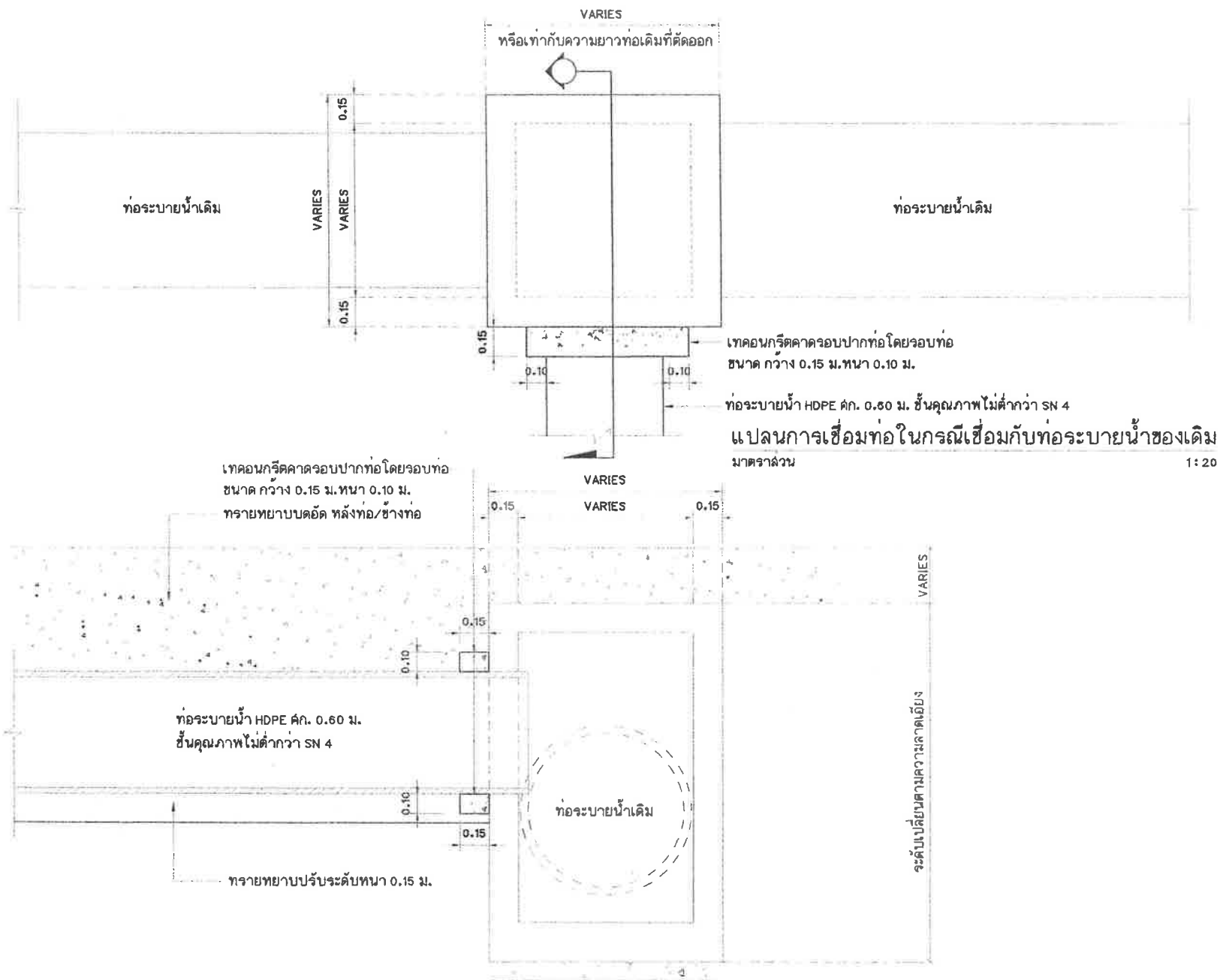
รูปตัดการเชื่อมต่อท่อระบายน้ำของเดิม มาตรฐาน
