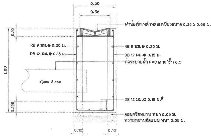
แบบขยายรูปตัด ① บ่อพักระบายน้ำ คลล. พร้อม ฝาบ่อพักรางวิเหล็กหล่อเหลี่ยม มาตราส่วน 1:15
