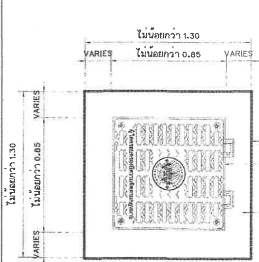
แบบขยายการเสริมระดับปากบ่อพัก ค.ล.ล. และติดตั้งบ่อพักใหม่แบบฝาเรียบ มาตราส่วน 1:20
