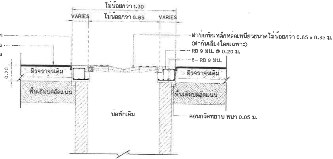
แบบขยายรูปตัดการเสัริมระดับปากบ่อพัก ค.ส.ล.และติดตั้งบ่อพักใหม่ (แบบฟารางวี) มาตราส่วน 1:20
