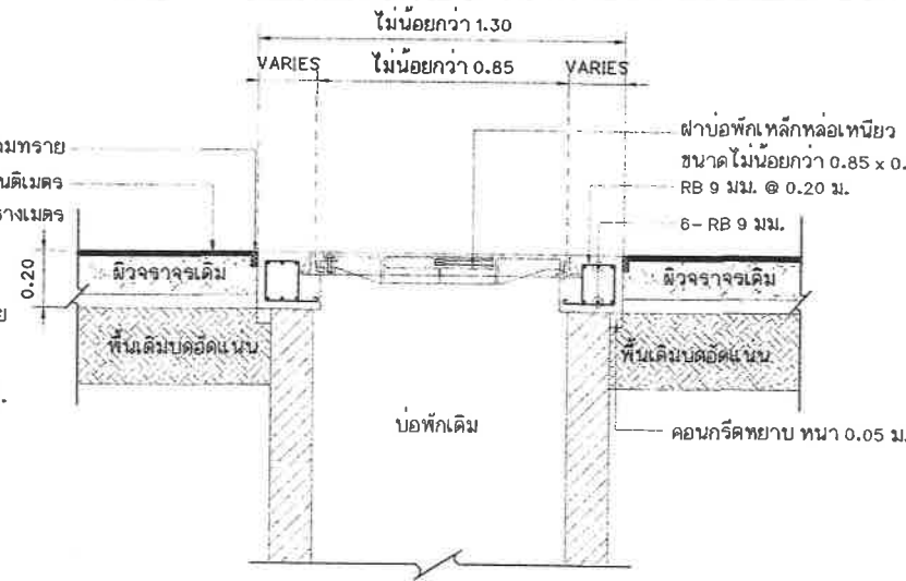
แบบขยายรูปตัดการเสริมระดับปากบ่อพัก ค.ล.ล. และติดตั้งบ่อพักใหม่แบบฝาเรียบ มาตราส่วน 1:20
