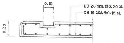
แบบขยาย ๓ (ผนังบ่อสูบน้ำ คสล.) มาตราส่วน 1:25
