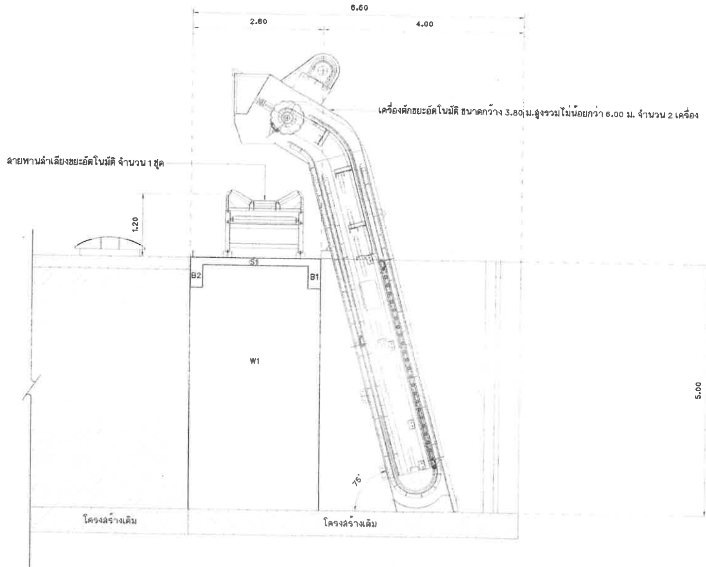
แบบขยาย รูปตัด 1
