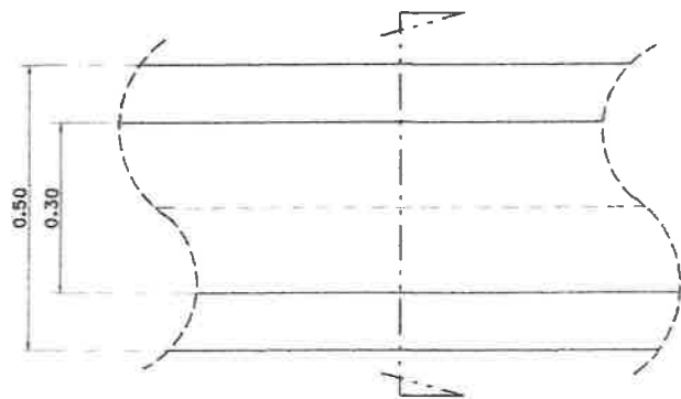
แบบขยายแปลนรางวี คสล. มาตราส่วน 1 : 10
