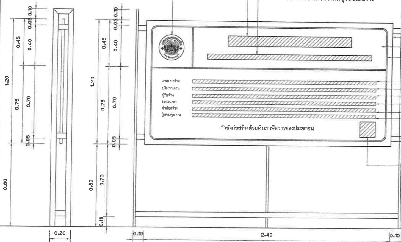
รูปด้านข้างโครงการ มาตราส่วน 1:15
