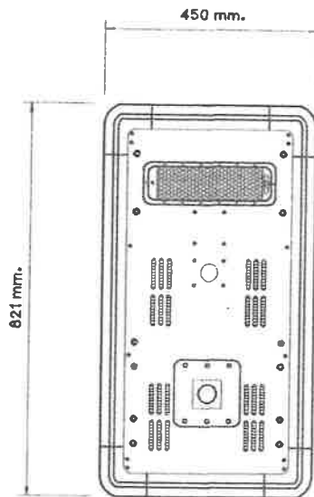
แบบขยายโคมไฟถนนโซล่าเซลล์ มาตราส่วน 1:20
