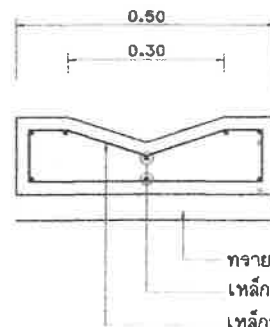
ขยายตัดรางวี คสล. มาตราส่วน 1 : 10
