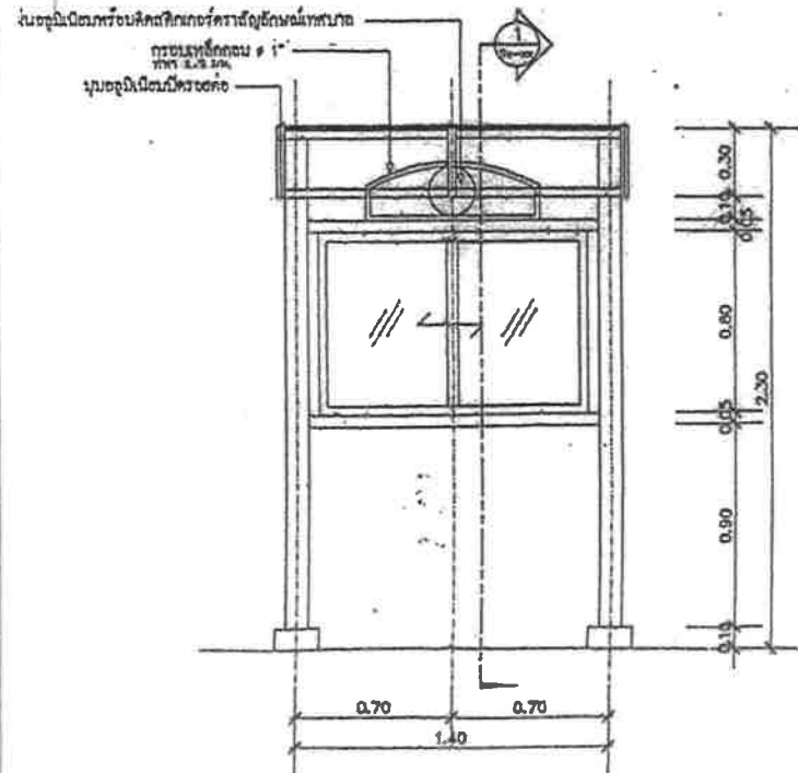
รูปด้าน SCALE 1:25
