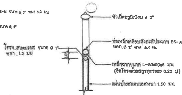
D แบบขยาย SCALE 1:10
