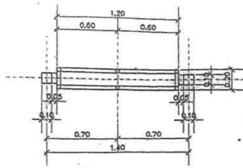
● แปลนฐานยึดประภาศ SCALE 1:25
