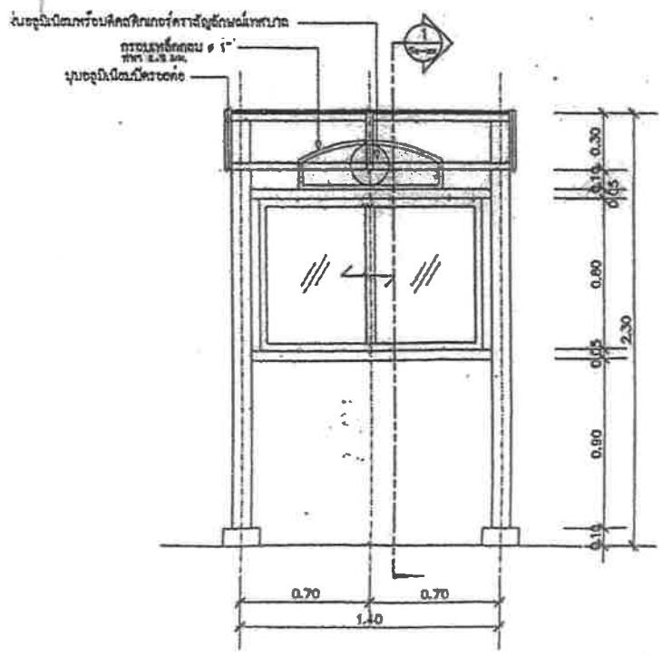
● รูปด้าน SCALE 1:25
