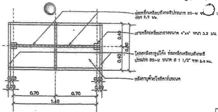
แปลนโครงสร้างคาน SCALE 1:25
