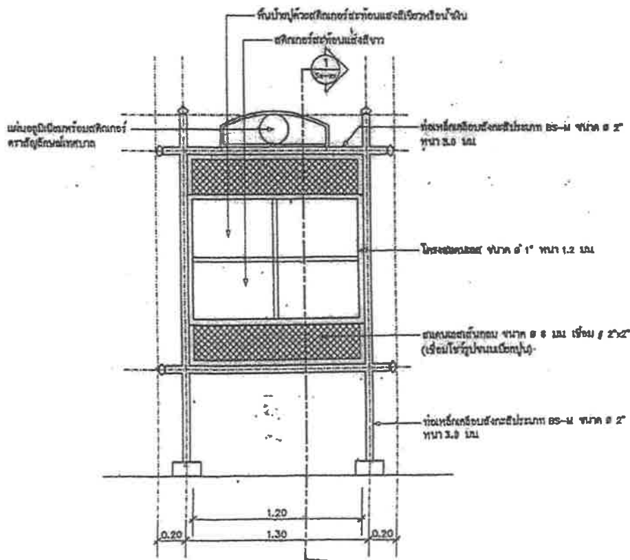
B รูปด้าน SCALE 1:25
