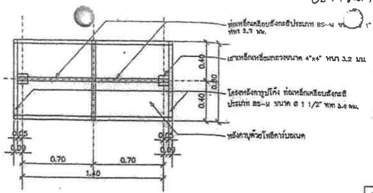
● แปลนโครงหลังคา SCALE 1:25
