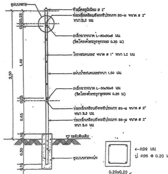
C รูปด้าน-1 SCALE 1:25
