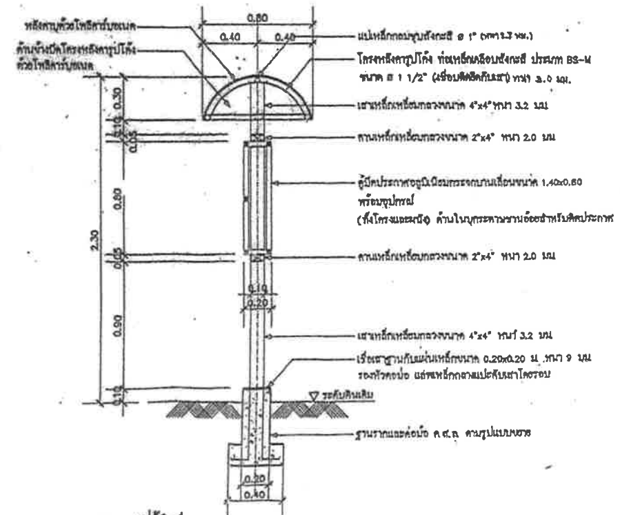
รูปตัด-1 SCALE 1:25
