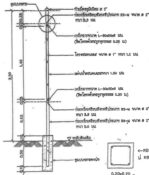
C รูปด้าน-1 SCALE 1:25
