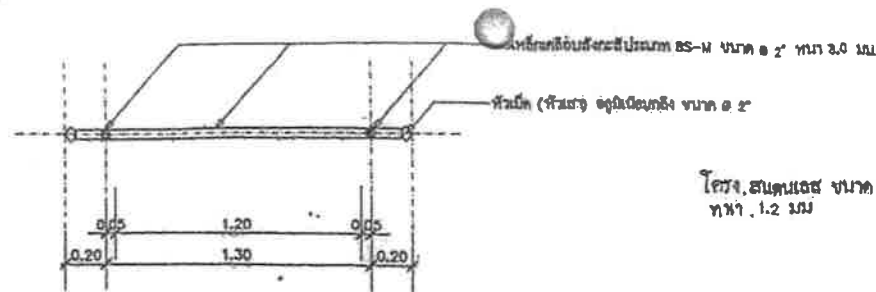
A แผนฐานฐาน SCALE 1:25
