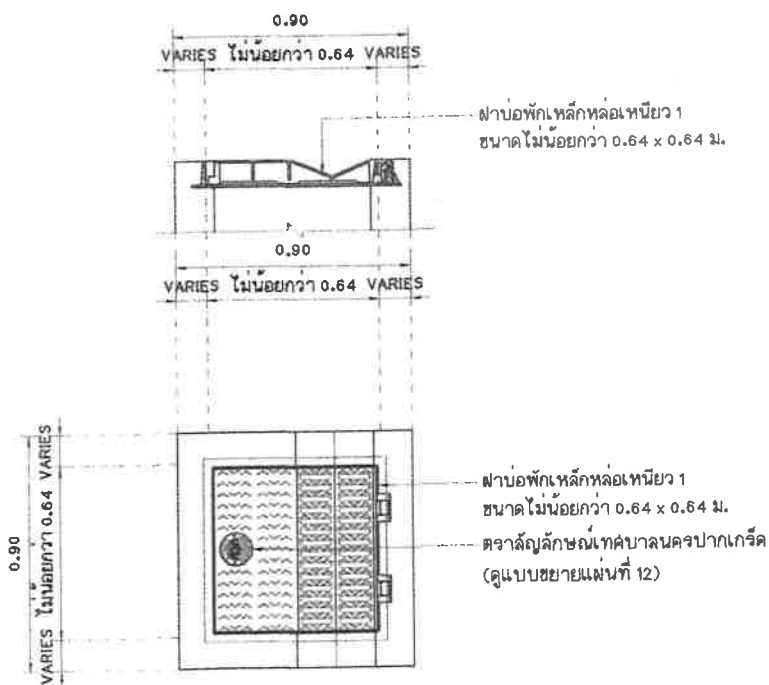
แบบขยายฝาบ่อพักเหล็กหล่อเหนียว 1
