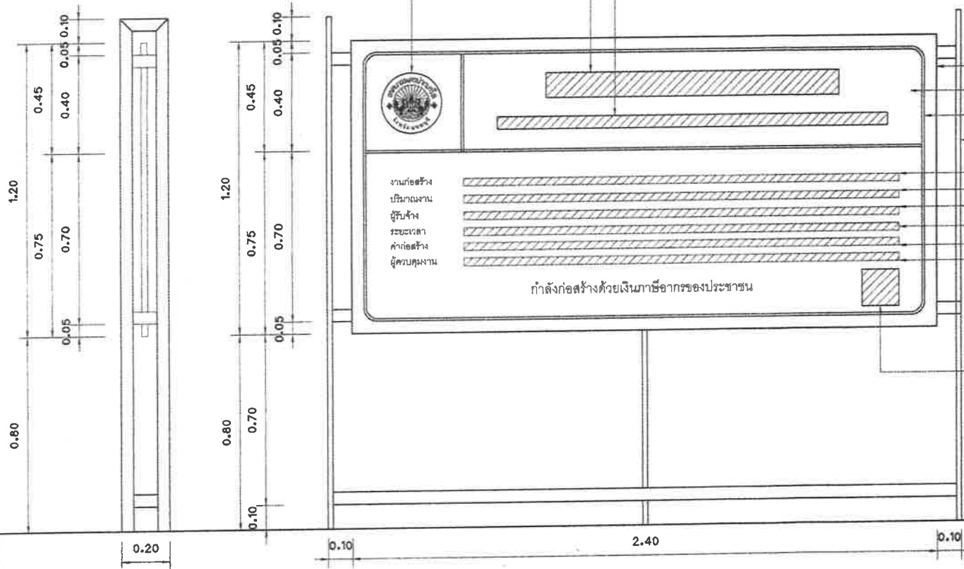
รูปด้านหน้าโครงการ มาตราส่วน 1 : 15
