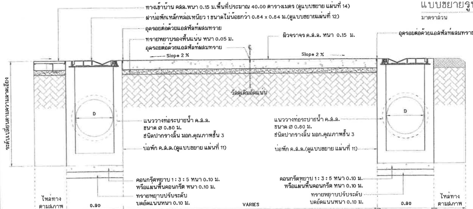
แบบขยายรูปตัด 2 มาตราส่วน 1:20
