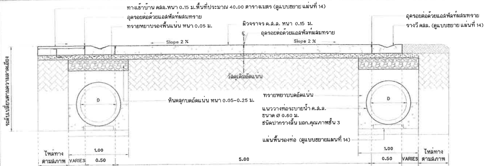
แบบขยายรูปตัด 1 มาตราส่วน 1:20
