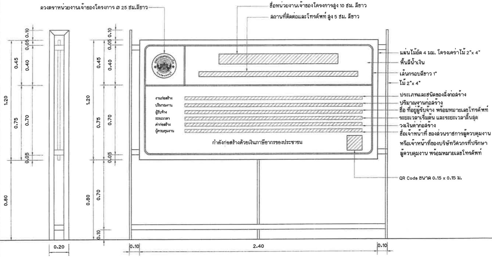
รูปด้านข้างโครงกร มาตราส่วน 1 : 15
