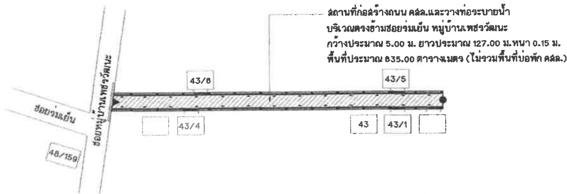
ผังบริเวณก่อสร้างถนน คสล.และวางท่อระบายน้ำ
