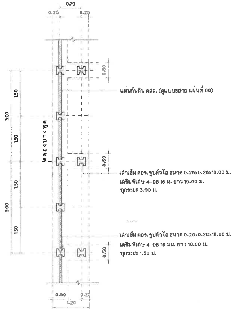
แปลนเหล้าเข็ม, คาน, พื้น คสล. มาตราส่วน 1:50
