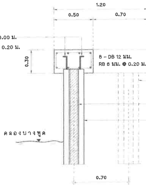
รูปตัด มาตราส่วน 1:20
