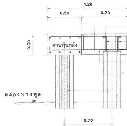
รูปตัด มาตราส่วน 1:20
