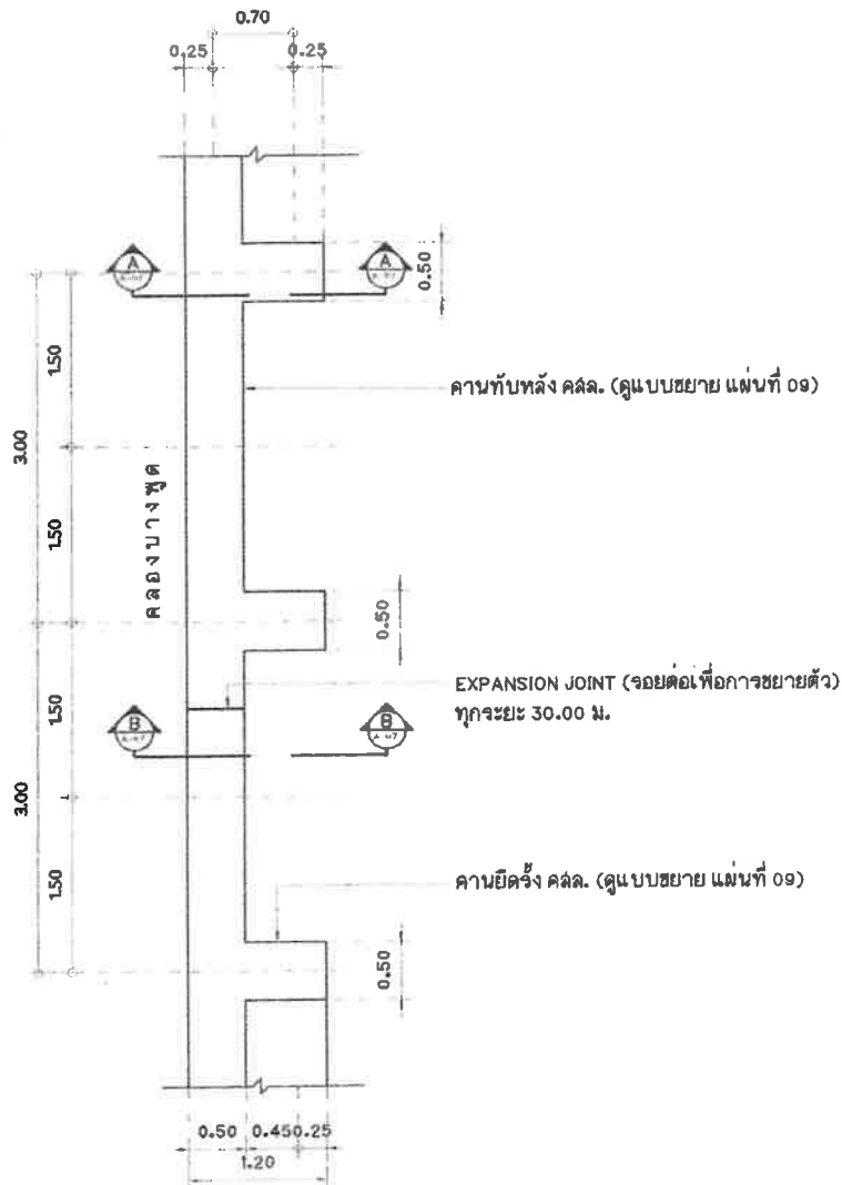
แปลนเชื่อม คสล. มาตราส่วน 1:50
