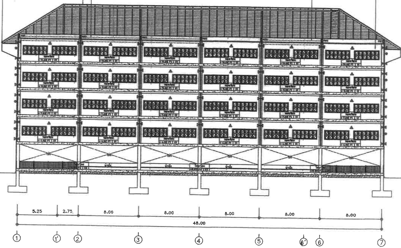
รูปตัด A มาตราส่วน 1:200
