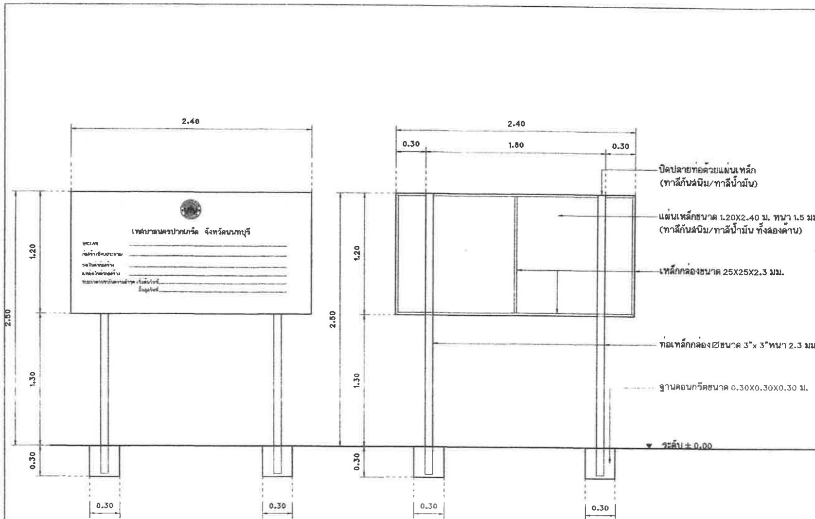
แบบแปลนโครงการ มาตราส่วน 1:25
