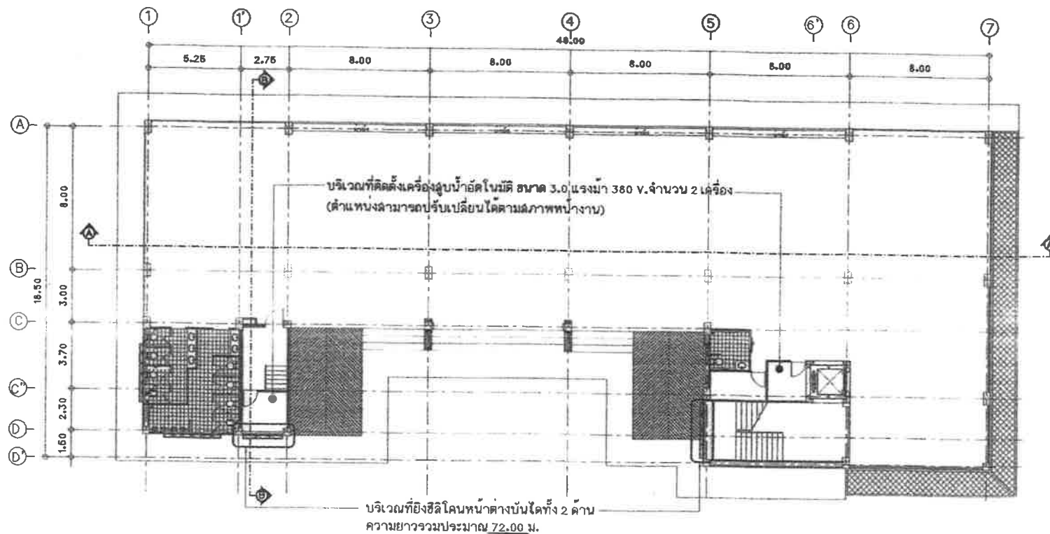
แปลนพื้นชั้น 1 มาตราส่วน 1:200
