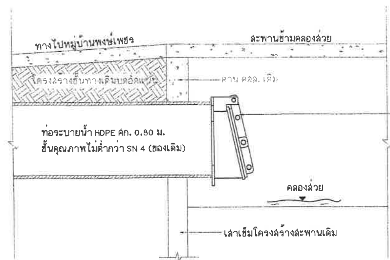
รูปตัดตามยาวการวางท่อระบายน้ำ มาตราส่วน 1:30
