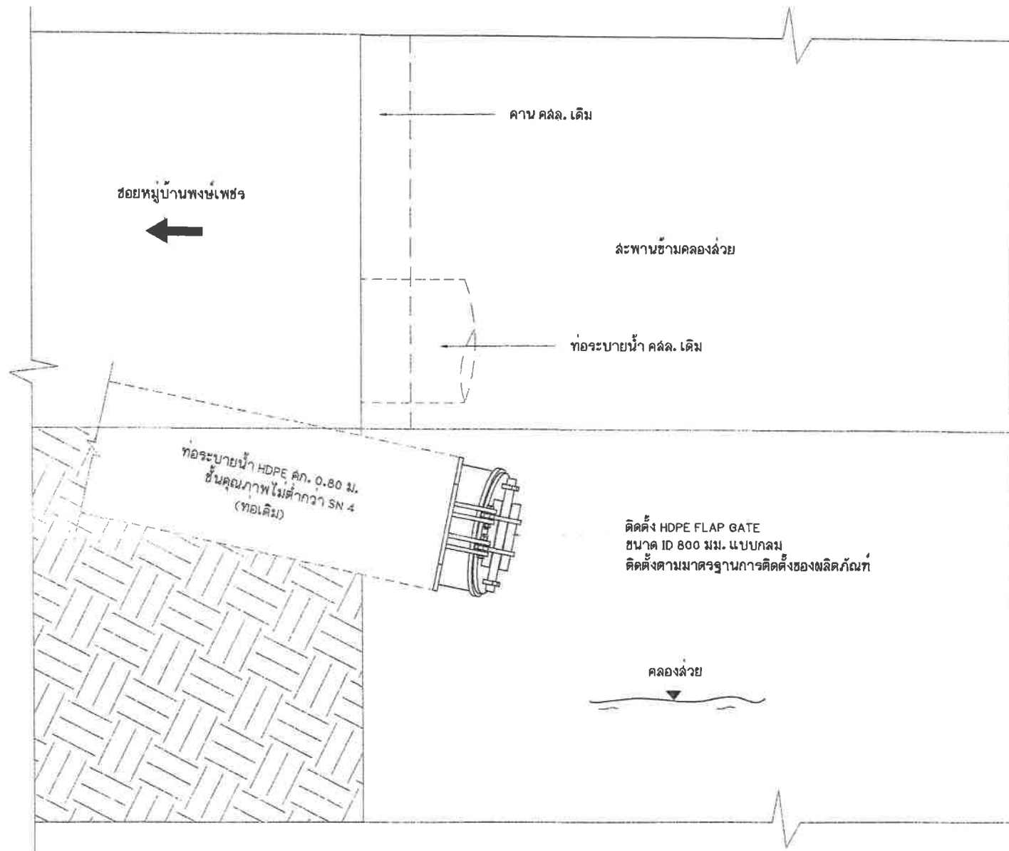
แบบขยาย A (แปลนขยายการติดตั้ง Flap Gate พังखा) มาตราส่วน 1 : 25
