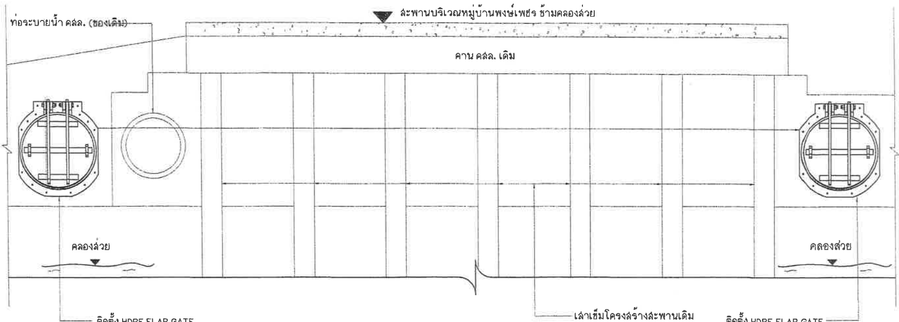
รูปตัด C รูปตัดตามขวางแสดงการติดตั้ง FLAP GATE มาตราส่วน 1:30
