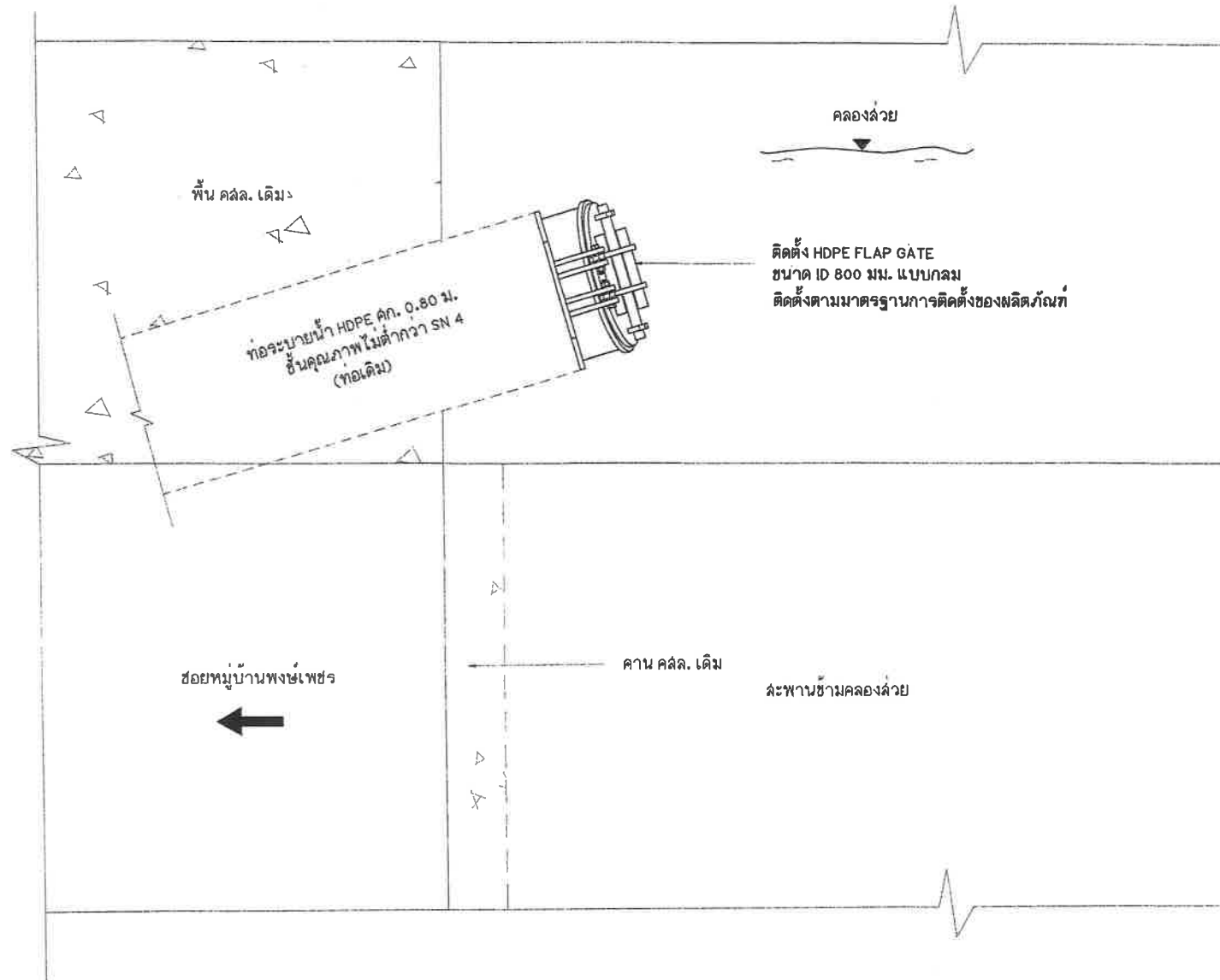
แบบขยาย B (แปลนขยายการติดตั้ง Flap Gate ฝั่งซ้าย) มาตราส่วน 1 : 25
