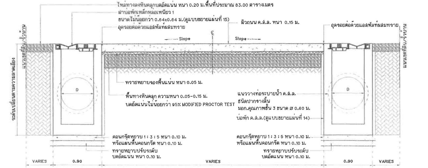
แบบขยายรูปตัด 2 (แบบมีโหล่ทางหินคลุก) มาตราส่วน 1:25
