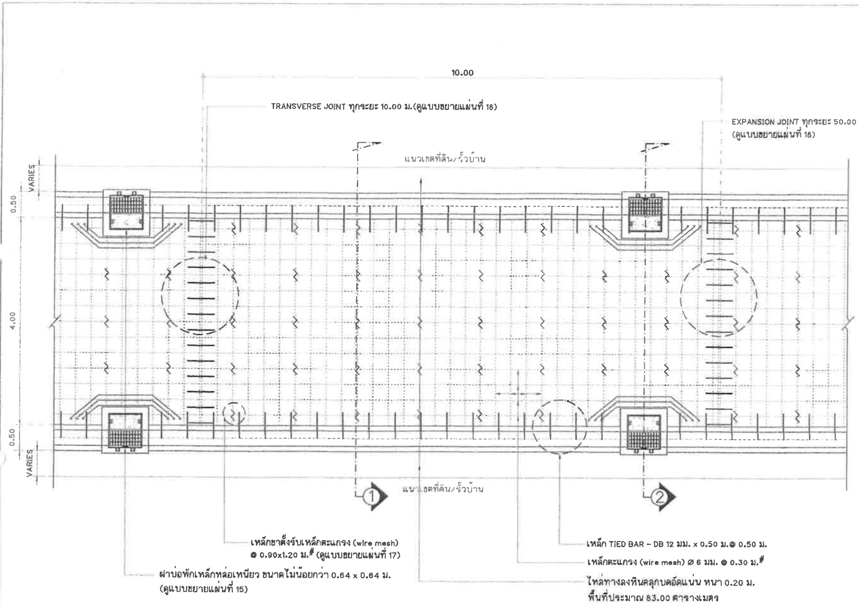
แปลนการวางเหล็กตะแกรงและรอยต่อถนน คสล. (แบบมีโหลทางหินคลุก)
