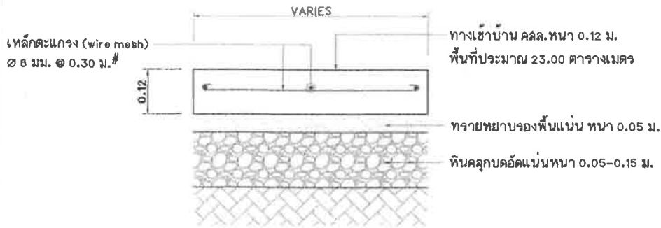
แบบขยายรูปตัดทางเข้าบ้าน คสล.หนา 0.12 ม. มาตรฐาน 1 : 30
