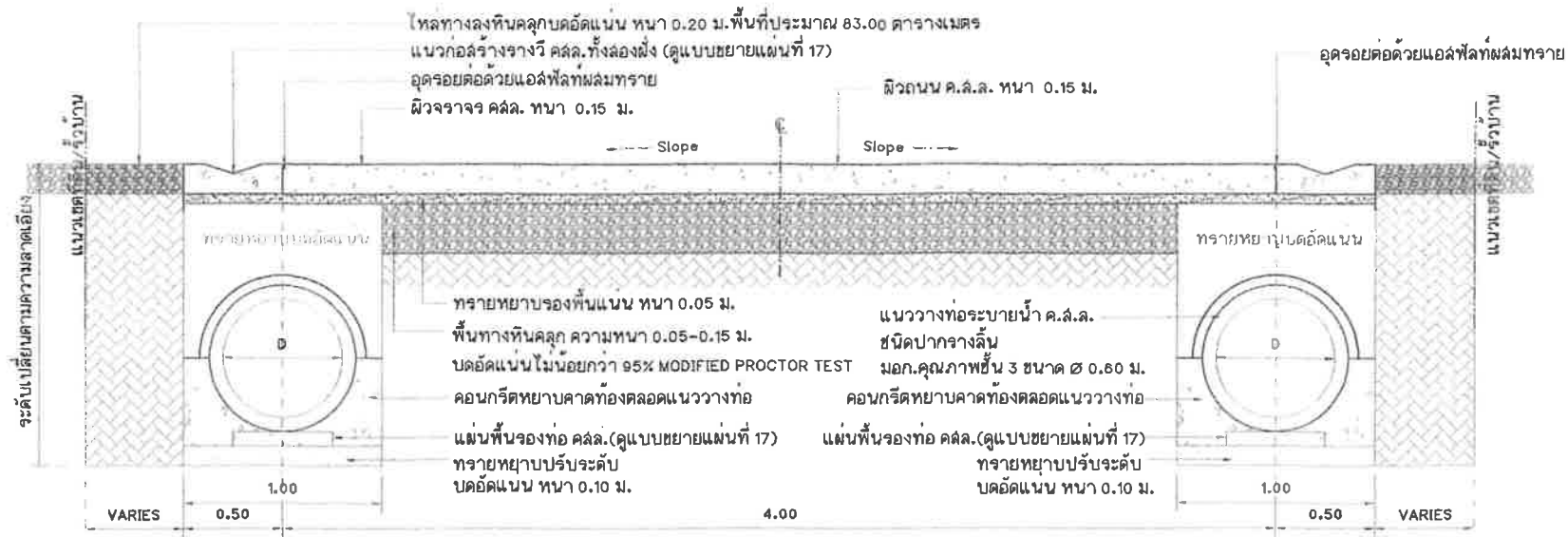
แบบขยายรูปตัด 1 (แบบมีโหล่ทางหินคลุก) มาตราส่วน 1:25
