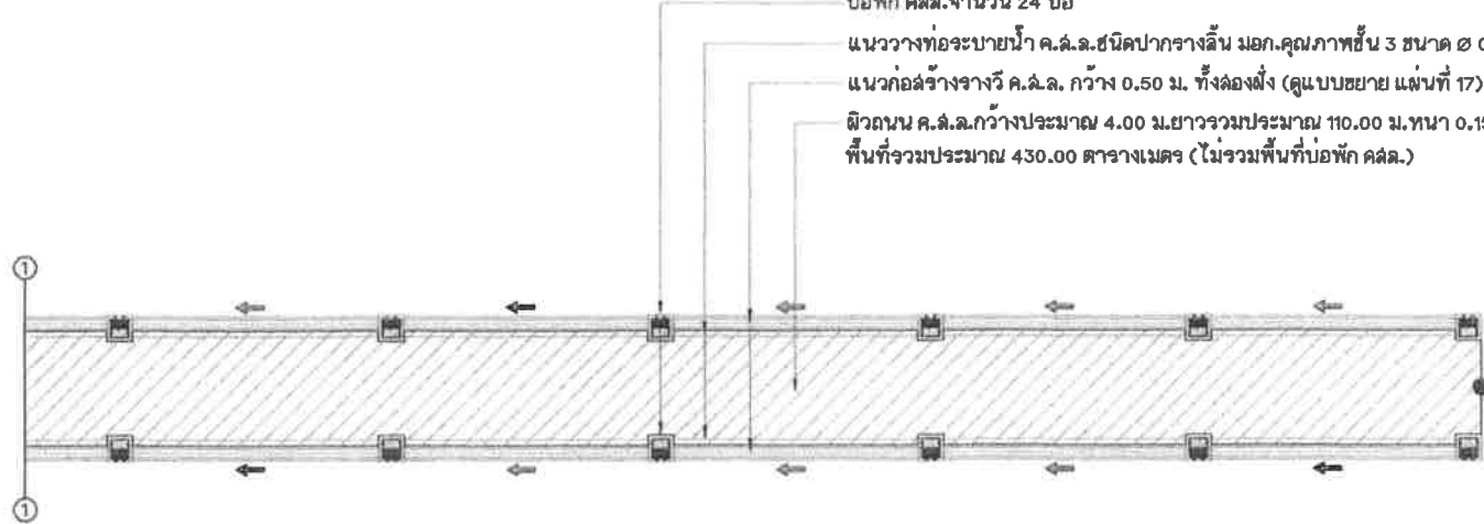
แปลนก่อสร้างถนน คลส.และท่อระบายน้ำ มาตรฐาน 1:200
