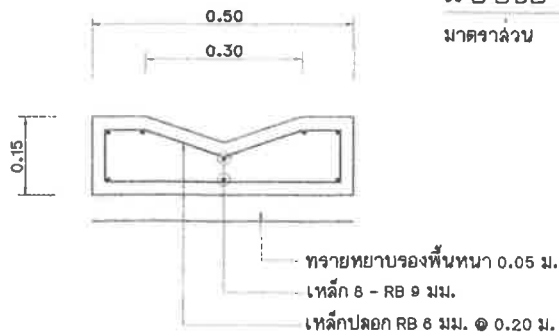
แบบขยายตัดรางวี คสล. มาตรฐาน 1 : 10
