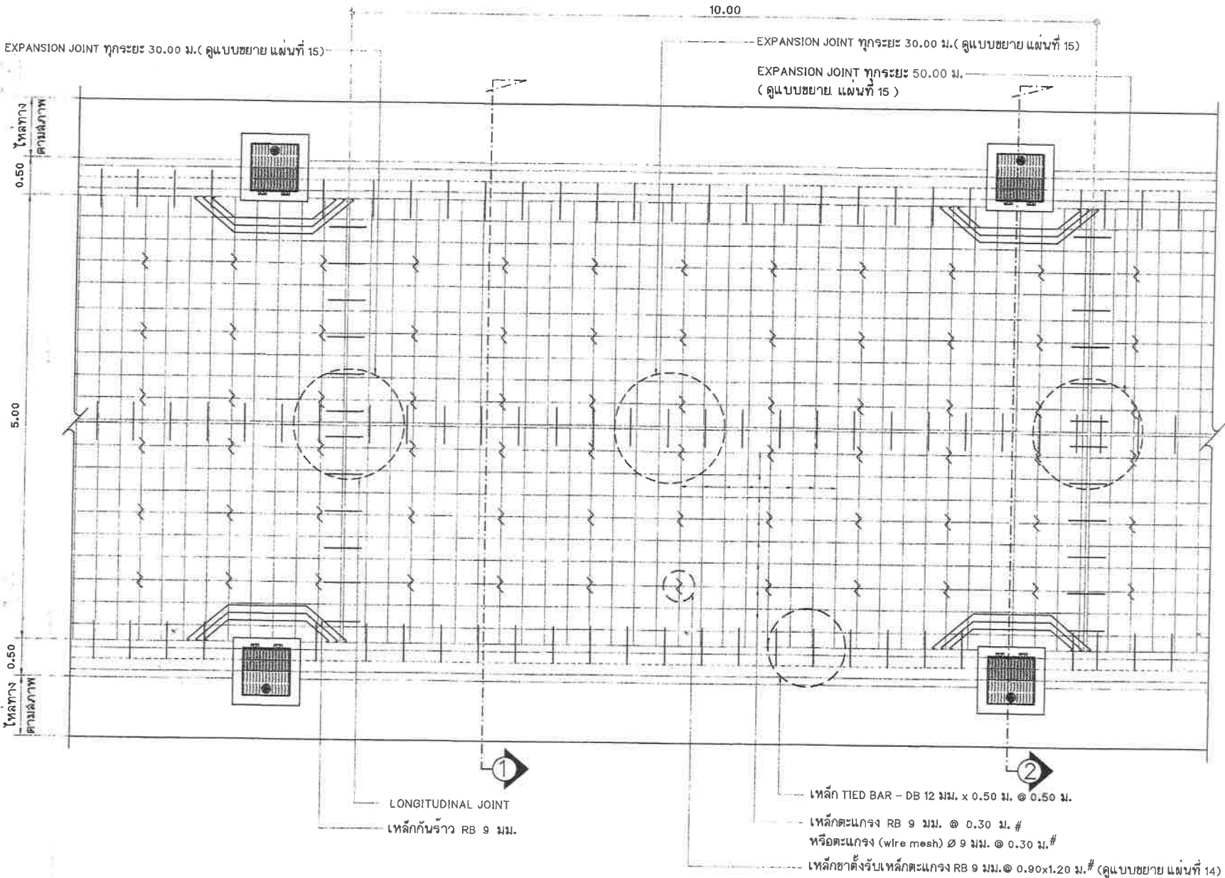
แปลนการวางเหล็กตะแกรงและรอยต่อถนน คสล. มาตรฐาน
