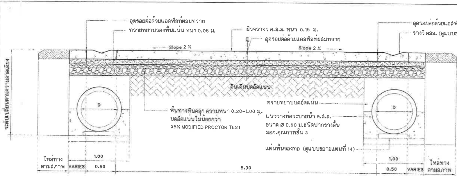
แบบขยายรูปตัด 1 มาตราส่วน 1:20
