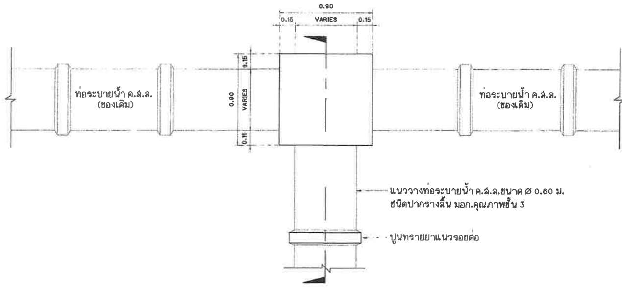
แปลนการเชื่อมต่อในกรณีเชื่อมกับท่อน้ำของเดิม มาตราส่วน 1:25
