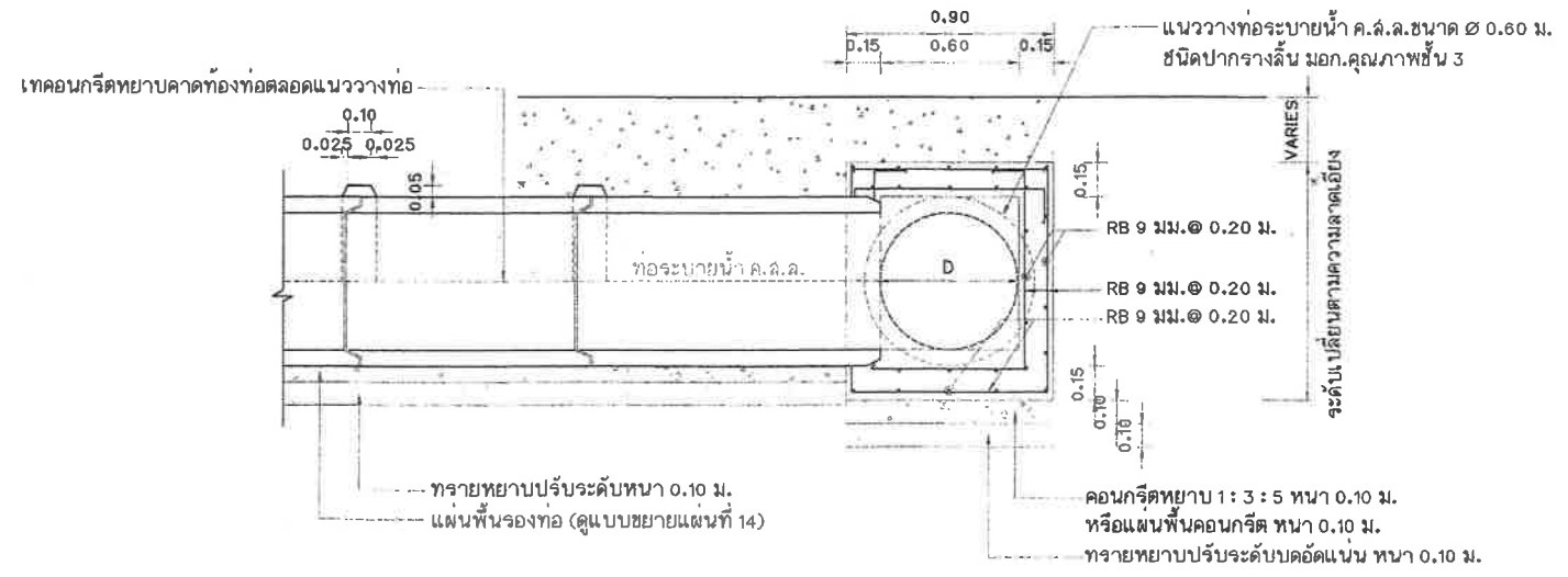
รูปตัดการเชื่อมต่อท่อน้ำของเดิม มาตราส่วน 1:25
