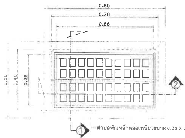
แบบขยายฝาบ่อพักรางวีเหล็กหล่อเหลี่ยม มาตราส่วน 1 : 10
