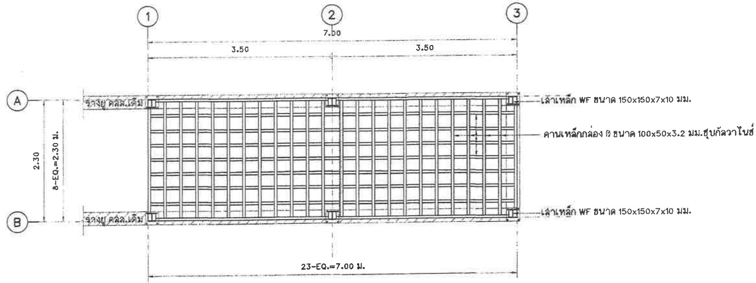
แปลนโครงสร้างพื้น มาตราส่วน 1:50
