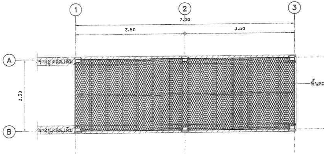
แปลนพื้นตะแกรงเหล็กฉีก มาตราส่วน 1:50
