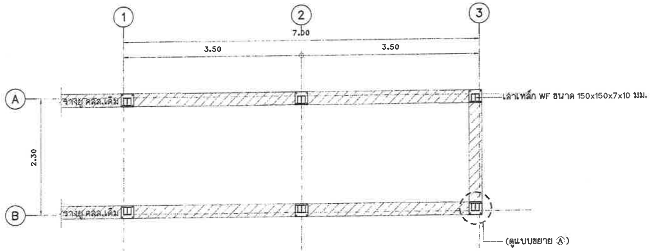
แปลนติดตั้งเสากับโครงยู่ คสล.เดิม มาตราส่วน 1:50
