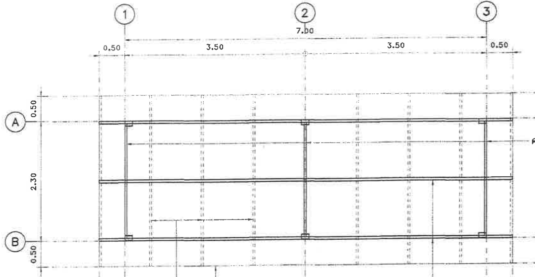
แปลนโครงสร้างหลังคา มาตราส่วน 1:50
