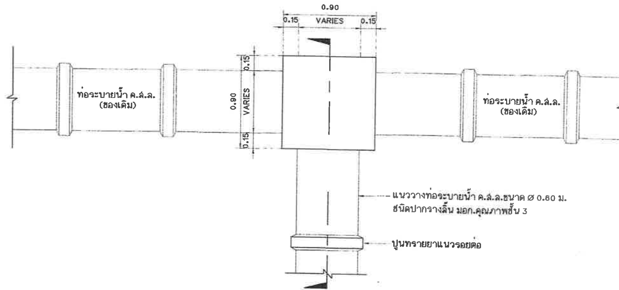
แปลนการเชื่อมต่อในกรณีเชื่อมกับทอระบายน้ำช่องเดิม มาตราส่วน 1: 25
