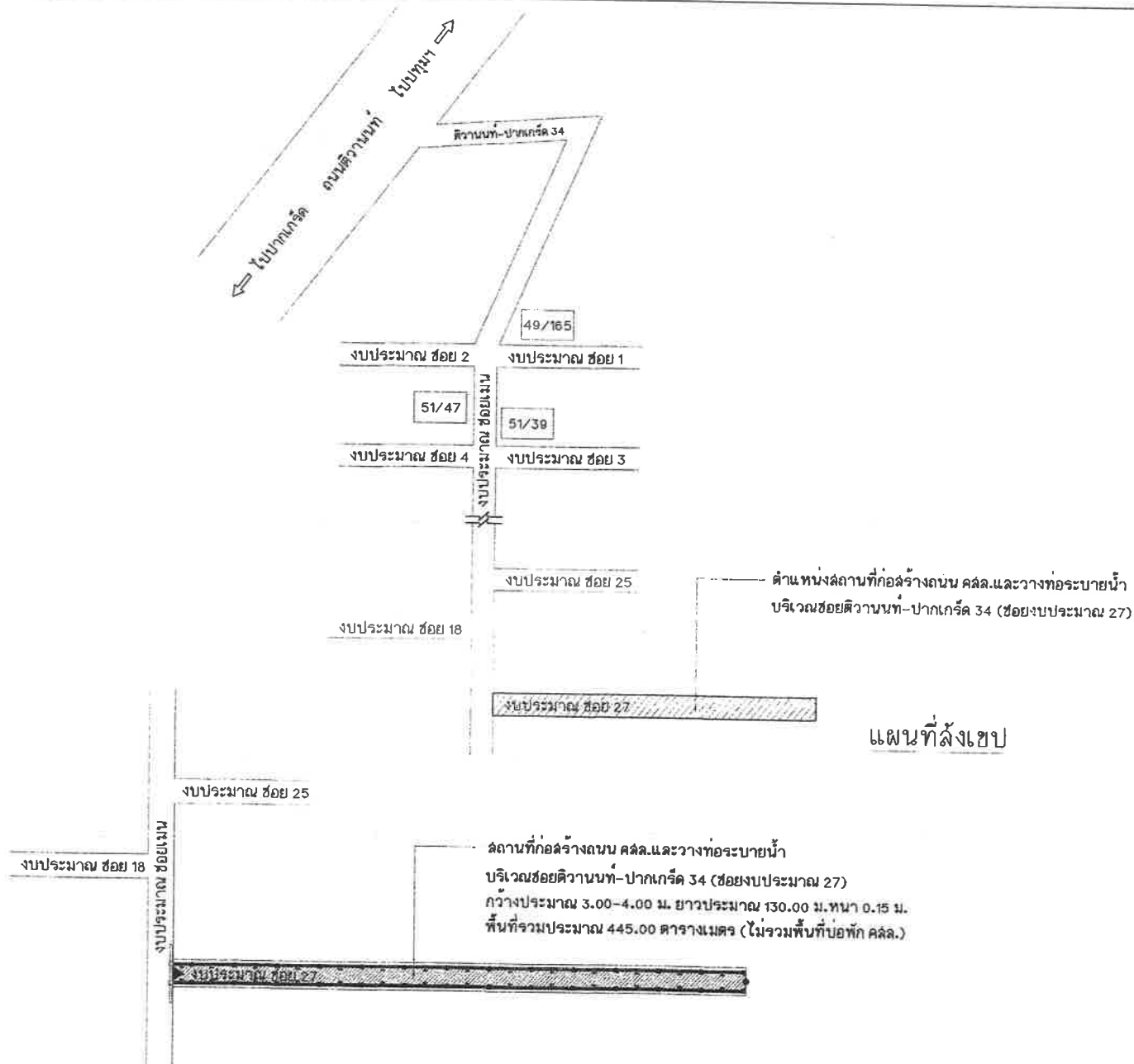
ผังบริเวณก่อสร้างถนน คสล.และวางท่อระบายน้ำ มาตราส่วน 1 : 1000
