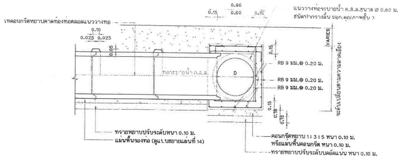
รูปตัดการเชื่อมต่อทอระบายน้ำช่องเดิม มาตราส่วน 1: 25
