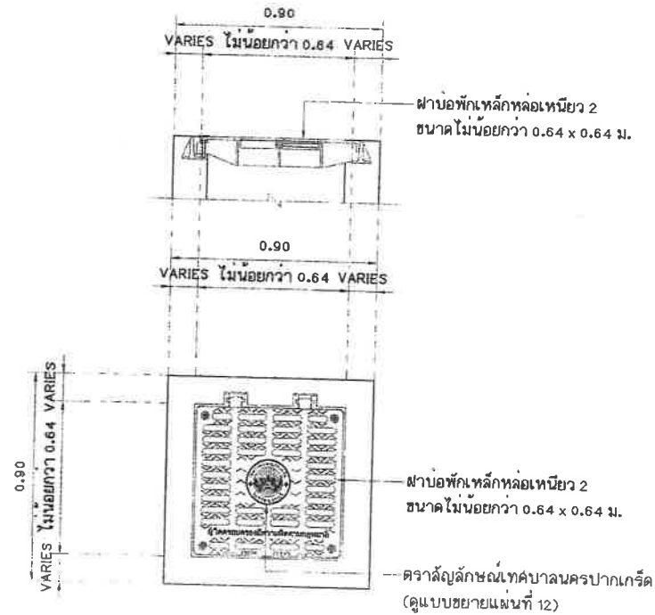
แบบขยายฝาบ่อพักเหล็กหล่อเหนียว 2 มาตราส่วน 1:20 (ฝาบ่อพัก และกรอบเป็นชนิดกั้นเสียงโดยเฉพาะ)
