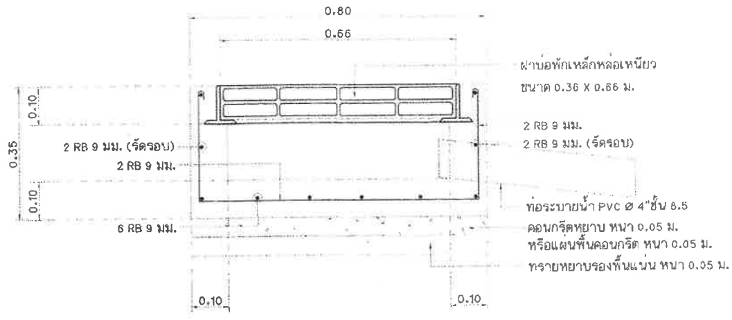
แบบขยายรูปตัด ② บ่อพักระบายน้ำ คล.ด. พร้อม ฝาบ่อพักรางวี มาตราส่วน 1:10
