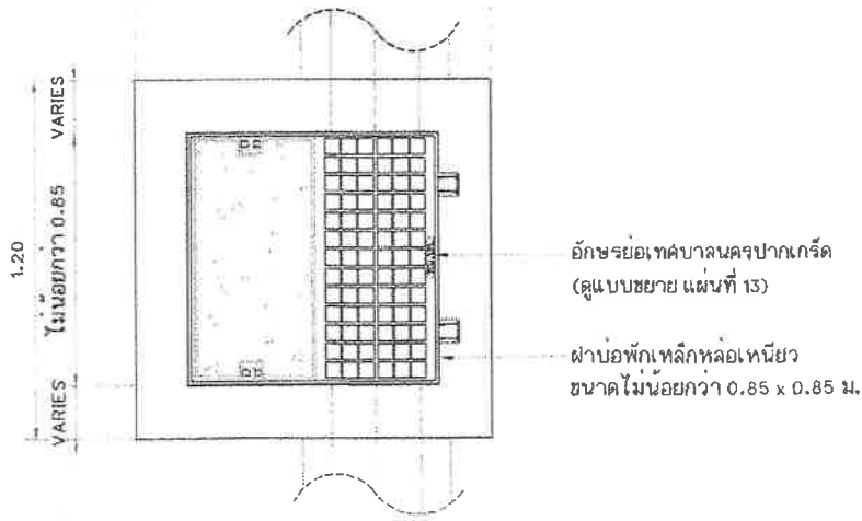
แบบขยายฝาบ่อพักเหล็กหล่อเหนียว 1 มาตราส่วน 1:20
