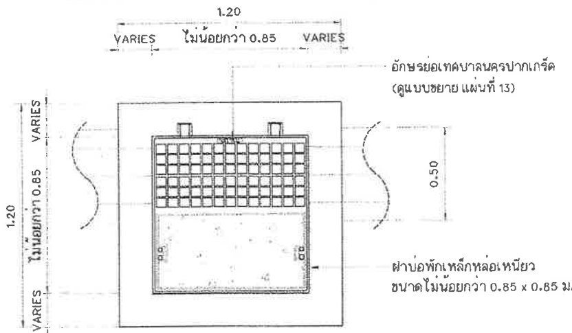
แบบขยายฝาบ่อพักเหล็กหล่อเหนียว 1 มาตราส่วน 1:20
