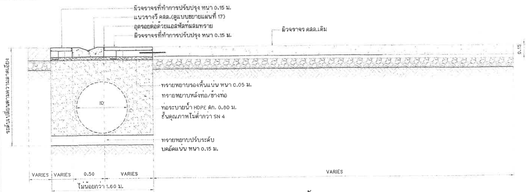
แบบขยายรูปตัด 1
