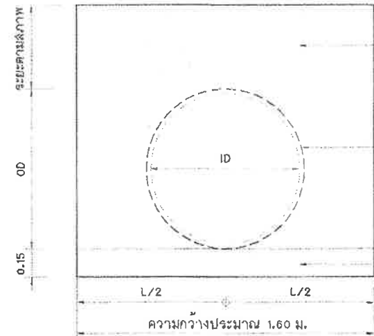
แบบขยายการวางท่อระบายน้ำ HDPE มาตราส่วน 1 : 20
