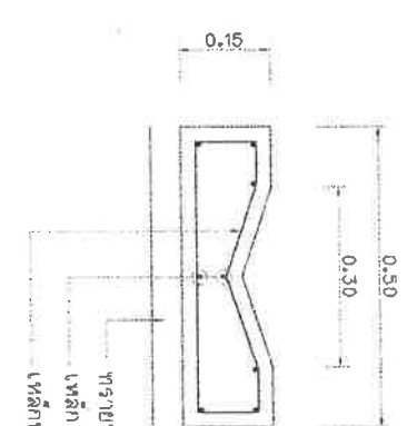
ขยายตัดรางวี คลื่น
