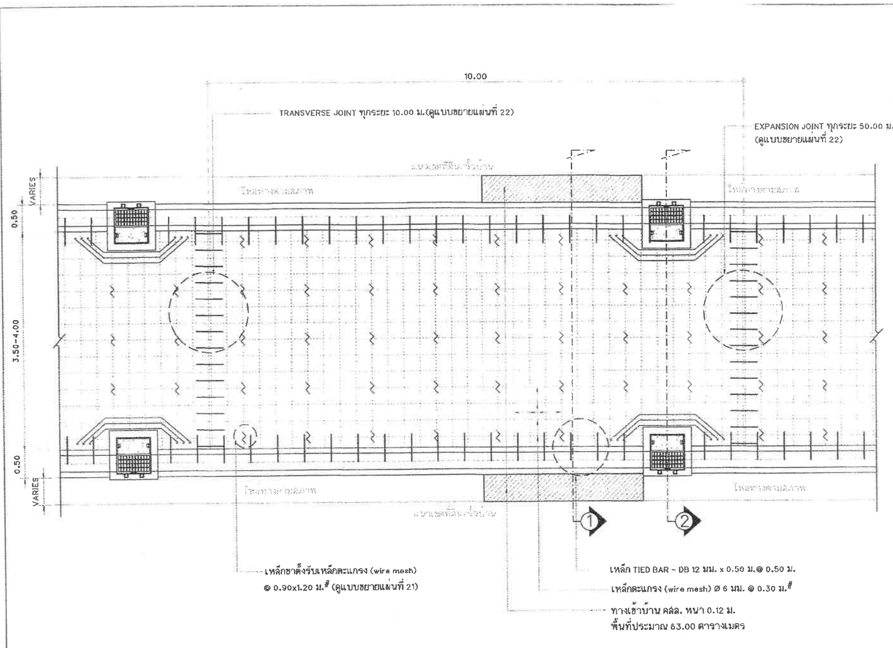
แปลนการวางเหล็กตะแกรงและรอยต่อถนน คสล. (แบบมีทางเข้าบ้าน คสล.) มาตรฐาน 1 : 50
