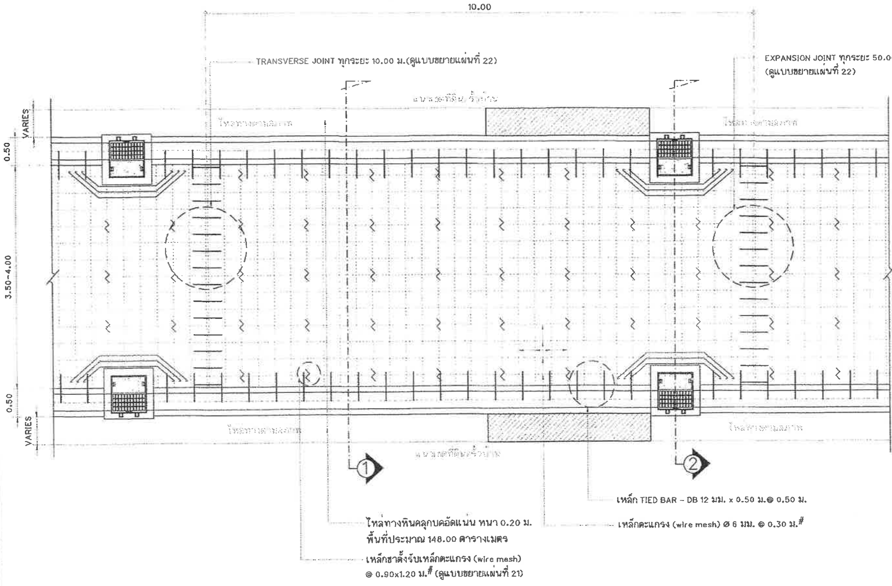
แปลนการวางเหล็กตะแกรงและรอยต่อถนนวน คสล. (แบบมีโหลทางหินคลุก)
