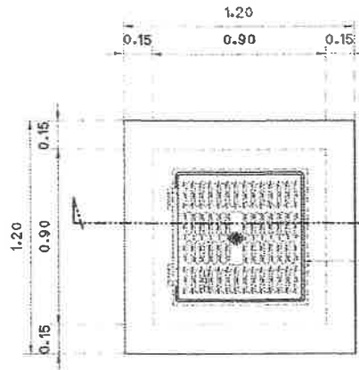
ฝาบ่อพักเหล็กหล่อเหลี่ยม 2 ขนาดไม่น้อยกว่า 0.64 x 0.64 ม.(ดูแบบขยายแผนที่ 16)
