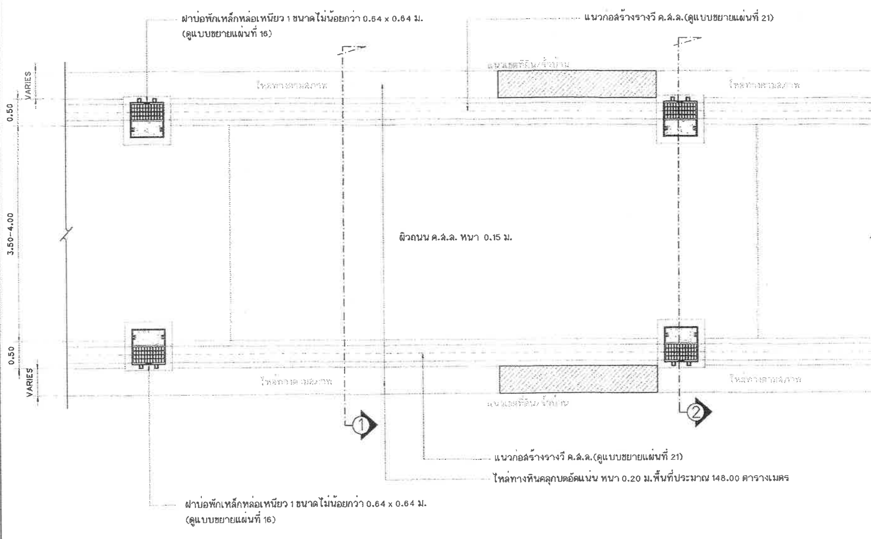
แปลนถนน และการวางข้อหัก คสล. (แบบมีไหล่ทางหินคลุก) มาตราส่วน 1 : 50
