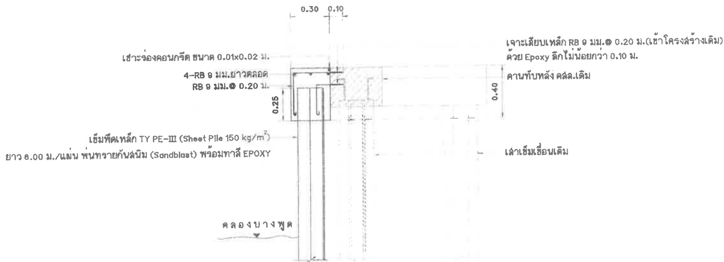
รูปตัด มาตราส่วน 1:20
