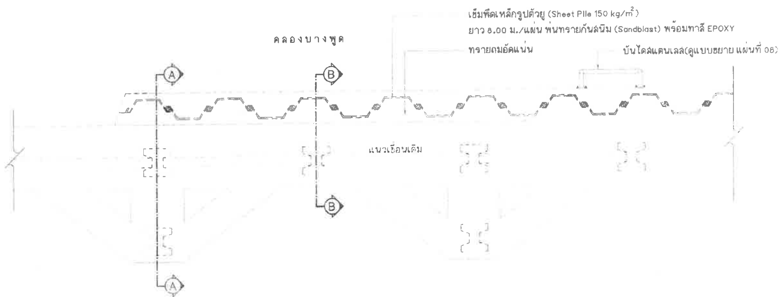
แปลนเข็มพืดเหล็ก TY PE-III มาตราส่วน 1: 25
