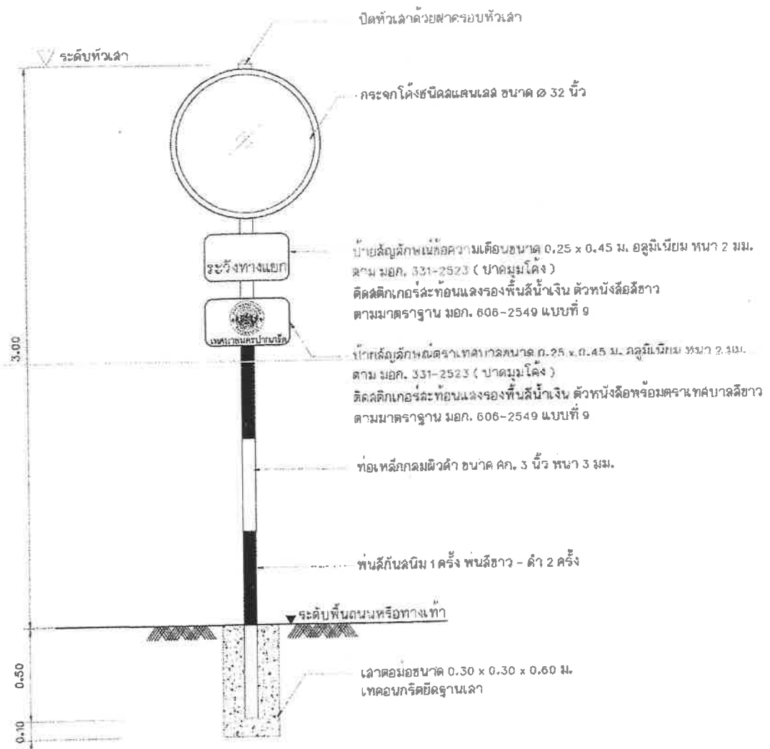
แบบขยายกระจกโค้ง มาตรฐาน 1:20
