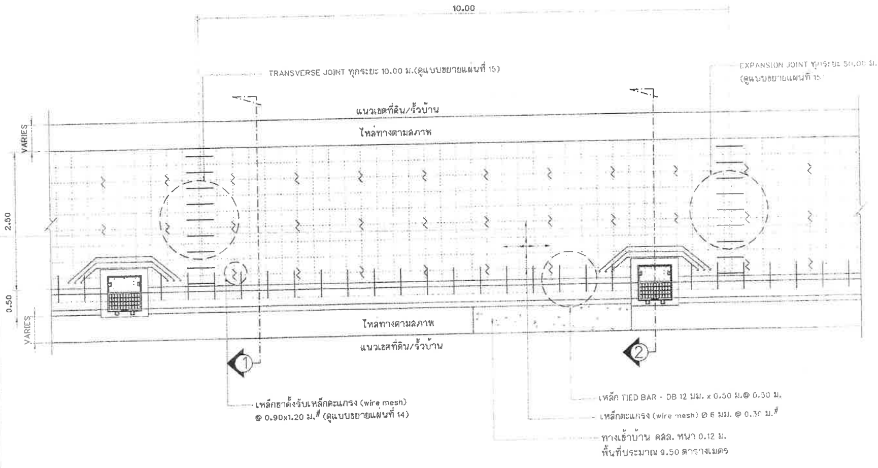
แปลนการวางเหล็กคานกรงและรอยต่อถนน คสล. มาตรฐาน 1 : 50
