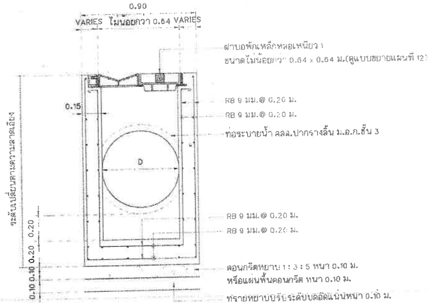
แบบขยายบดพิก คลล. มาตราส่วน 1 : 20
