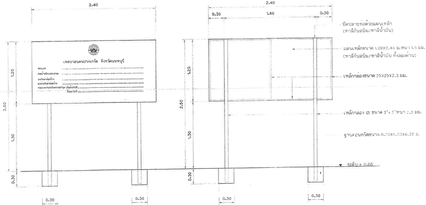
แบบป้ายโครงการ มาตรฐาน 1:25
