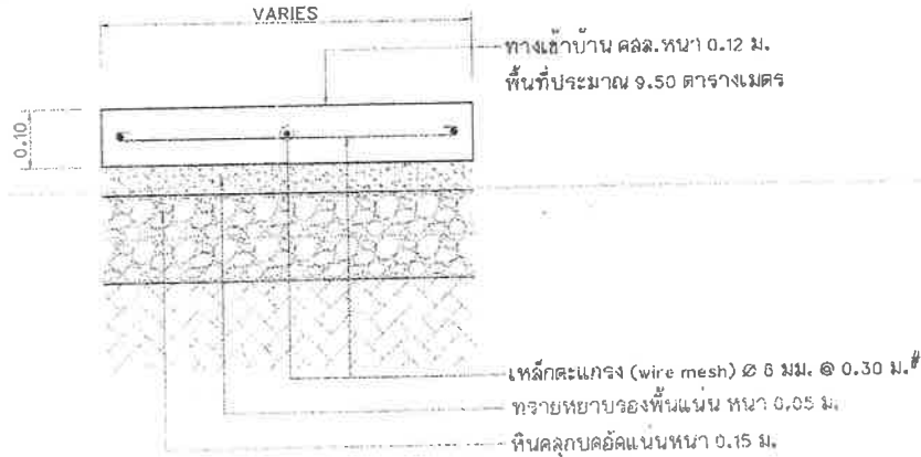
แบบขยายรูปตัดทางเข้าบ้าน คสล.หนา 0.12 ม.
