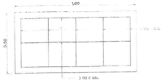
แบบขยายแปลนแผ่นพื้นรองทอ
