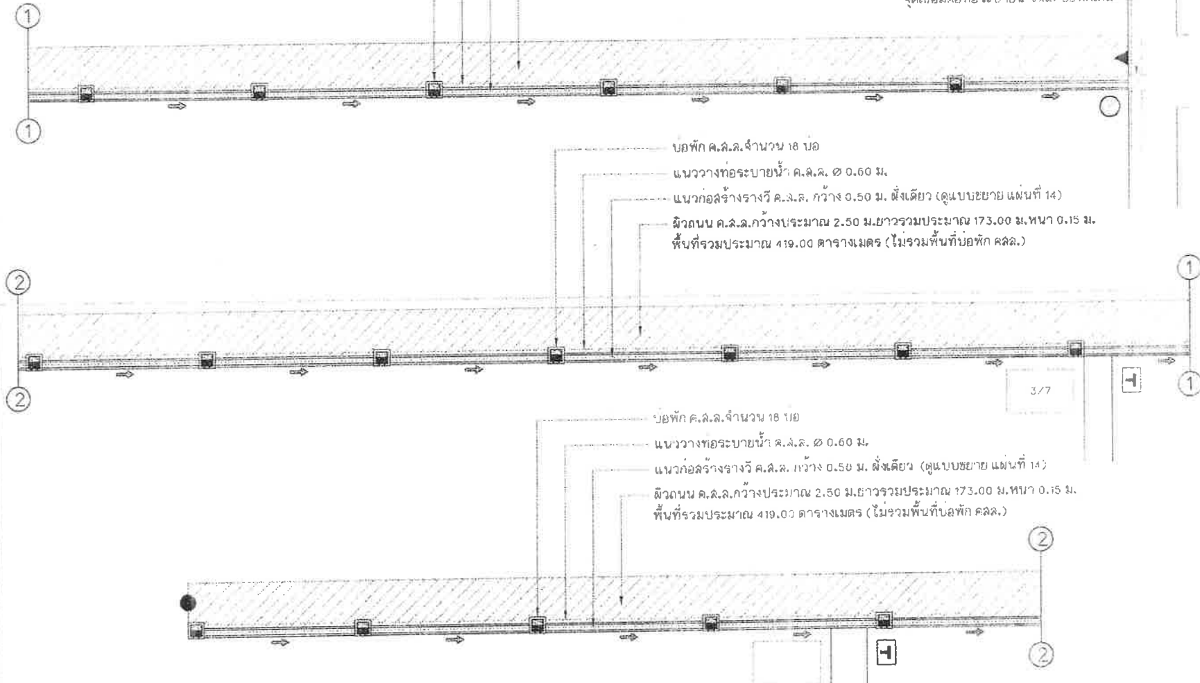
แปลนก่อสร้างปรับปรุงถนน และวางท่อระบายน้ำ มาตราส่วน 1:200
