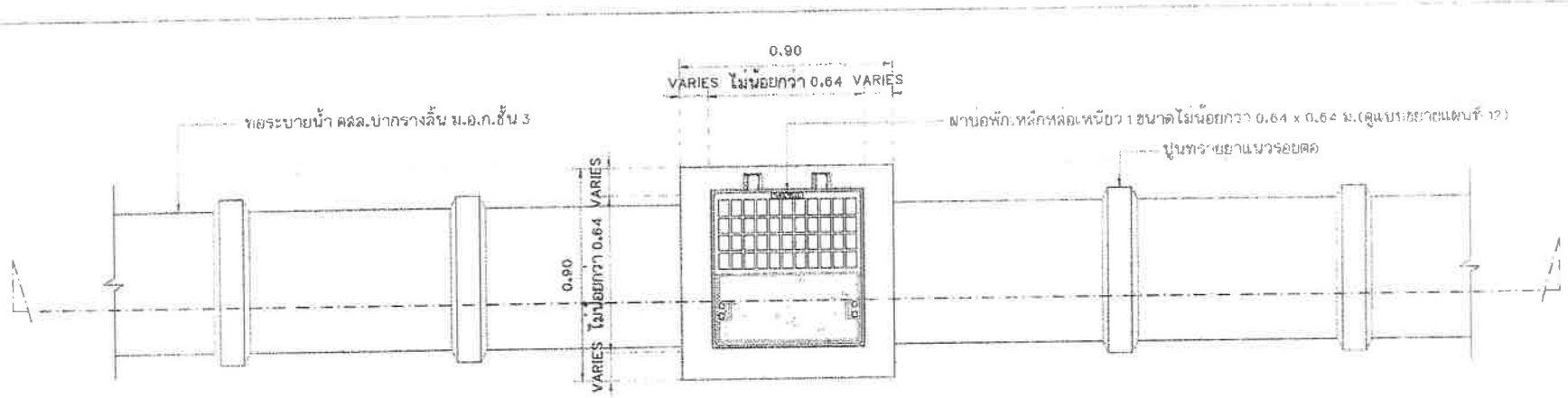
แปลนการวางท่อระบายน้ำ มาตรฐาน 1:20
