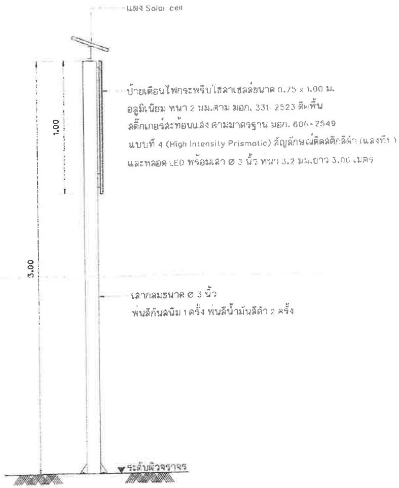
รูปด้านข้างป้ายเตือนไฟกระพริบโซล่าเซลล์ มาตรฐาน 1:20
