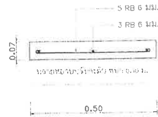
แบบขยายรูปตัดแผ่นพื้นรองทอ
