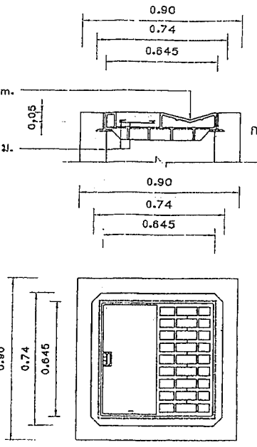
แบบขยายฝาบ่อพักเหล็กหล่อเหนียว 1 มาตราส่วน 1:20
