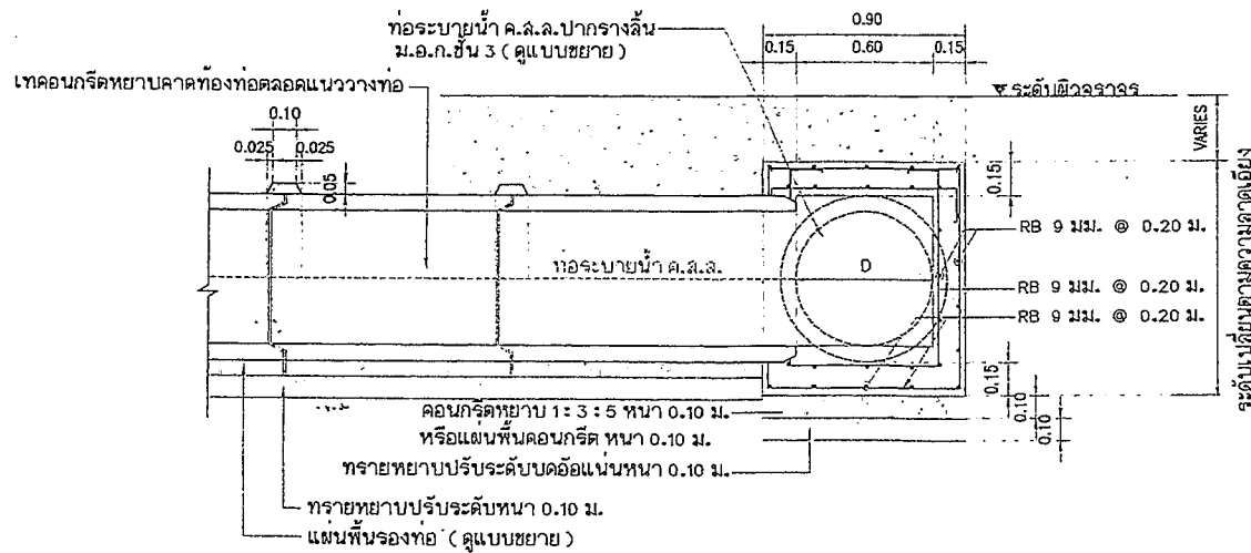
รูปตัดการเชื่อมต่อในกรณีเชื่อมกับท่อระบายน้ำของเดิม มาตราส่วน 1:25
