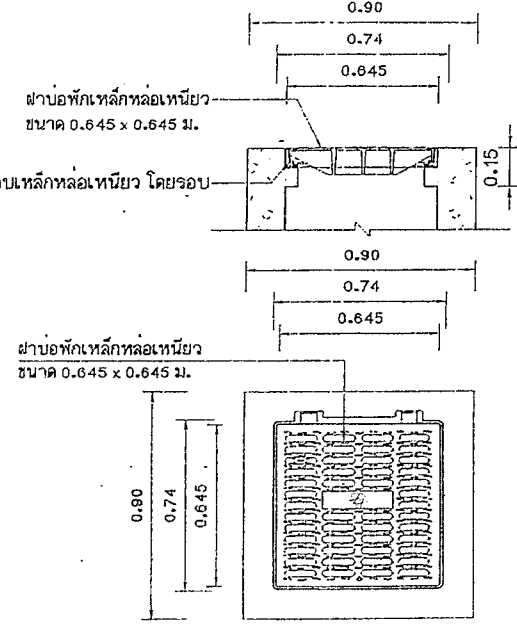
แบบขยายฝาบ่อพักเหล็กหล่อเหนียว 2 มาตราส่วน 1:20
