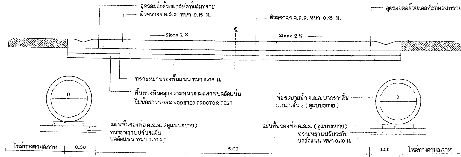
แบบขยายรูปตัด 1 มาตราส่วน 1:20
