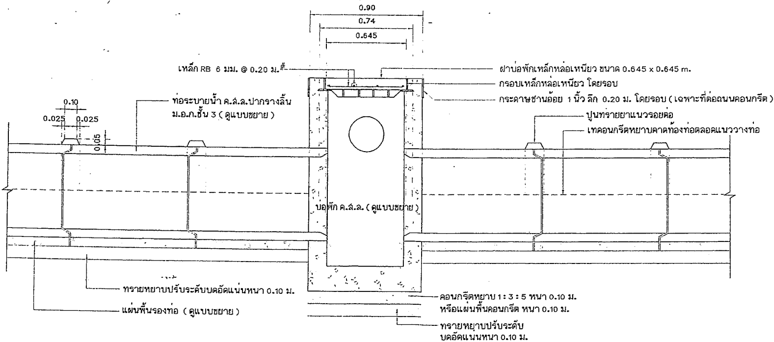
รูปตัดตามยาวการวางท่อระบายน้ำ
