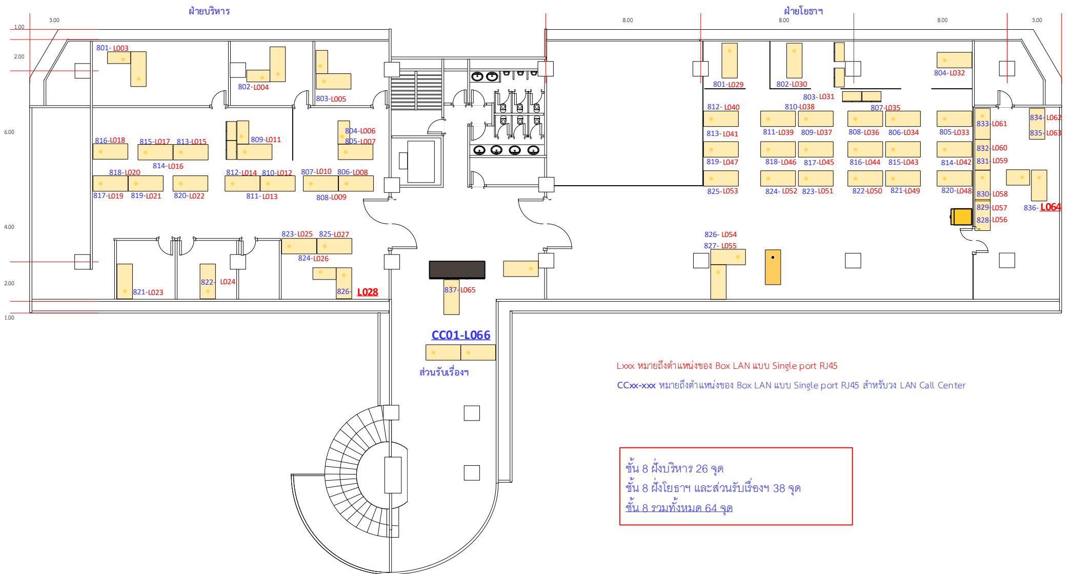
ผังแสดงตำแหน่งจุดติดตั้ง LAN Outlet
