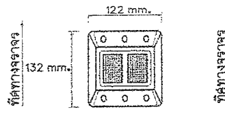
แปลนแสงปุ่มสะท้อนแสงชนิดล่องด้าน (ชนิดพลังงานแสงอาทิตย์)
