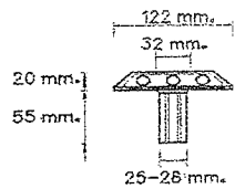
รูปด้านข้างปุ่มสะท้อนแสงชนิดล่องด้าน (ชนิดพลังงานแสงอาทิตย์)
