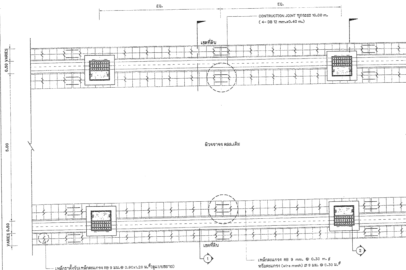
แบบขยายเหล็กขาค้างรับเหล็กตะแกรงและรอยต่อถนน มาตราส่วน 1:50
