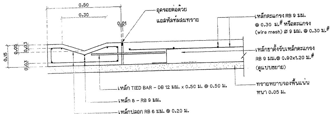
แบบขยายตัดขวางวิ คศล. มาตราส่วน 1 : 10
