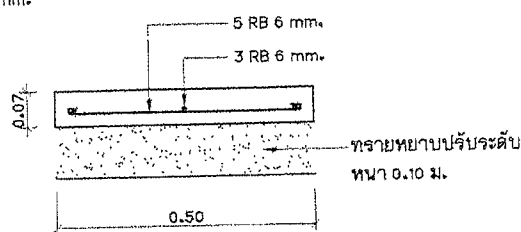
รูปตัด มาตราส่วน 1 : 10
