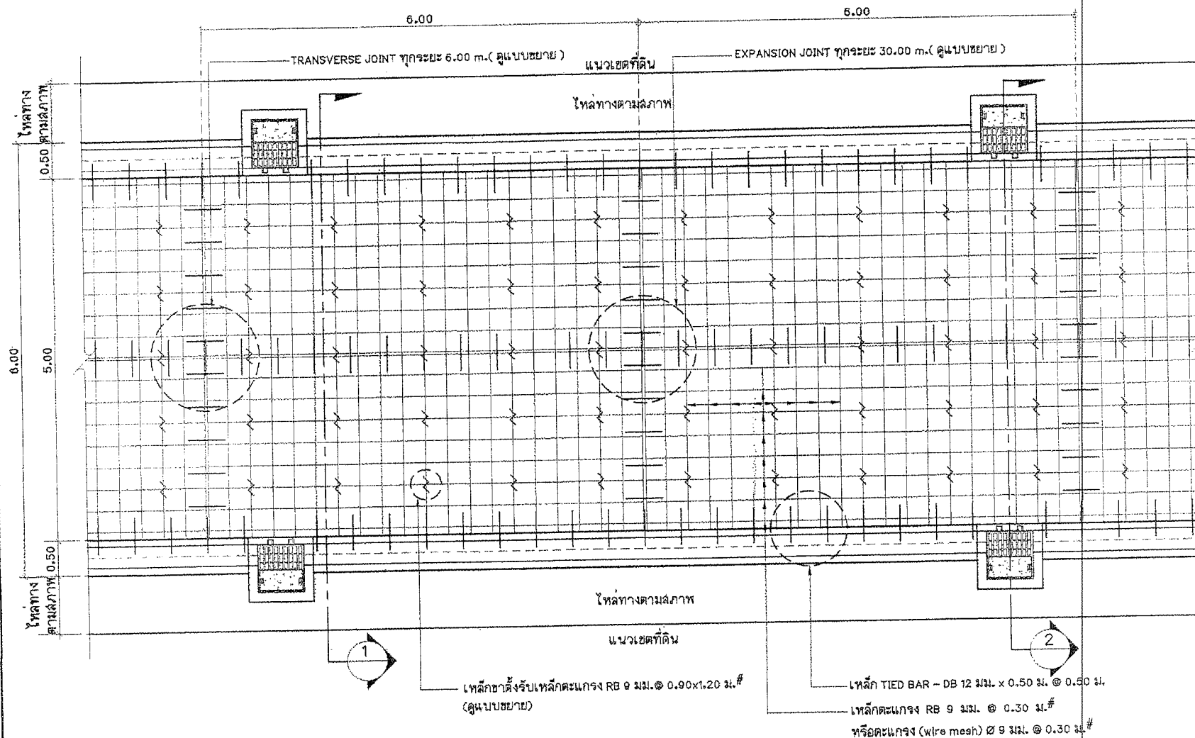
แปลนการวางเหล็กตะแกรงและรอยต่อถนน คลัด. มาตราส่วน 1 : 50
