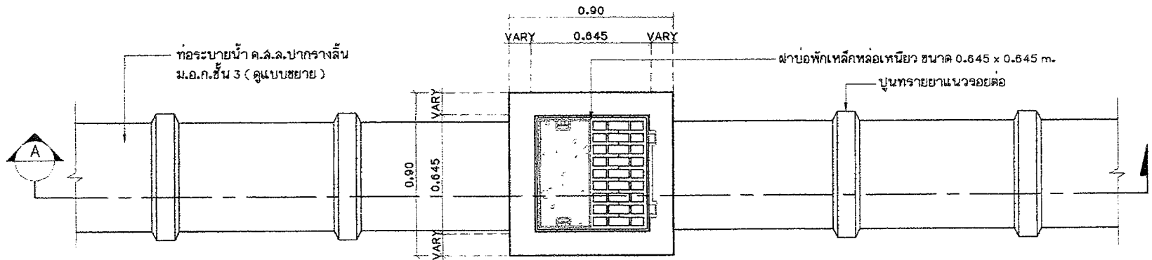
แปลนการวางท่อน้ำ มาตราส่วน 1 : 20
