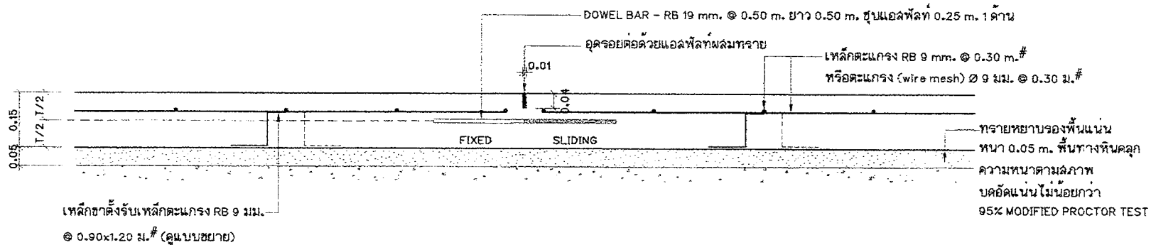
แบบขยาย TRANSVERSE JOINT
