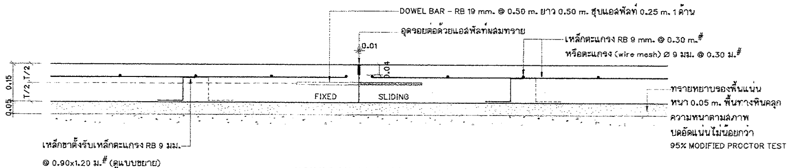
แบบขยาย CONSTRUCTION JOINT
