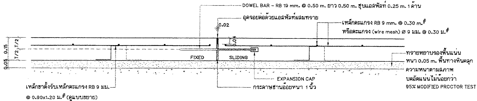
แบบขยาย EXPANSION JOINT
