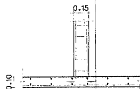
แบบขยายเสริมเหล็กเสา C1 มาตราส่วน 1:25
