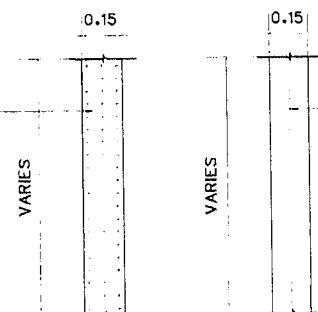
แปลนขยายรางระบายน้ำล้นแดนเลด มาตราส่วน 1:20
