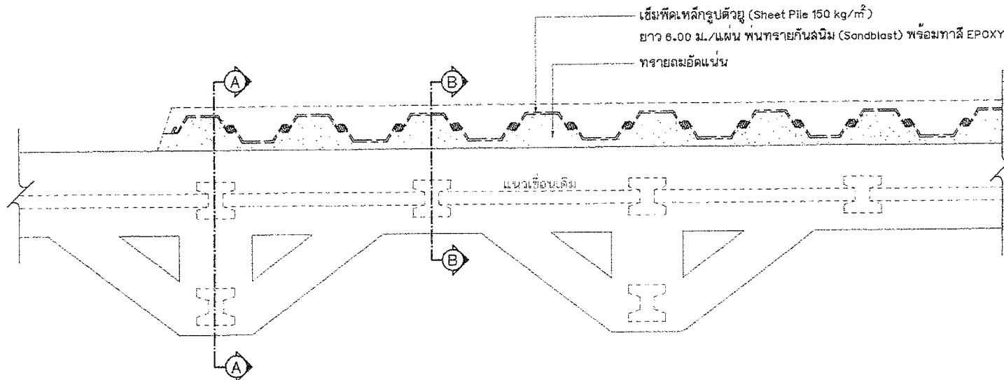
แปลนเข็มพืดเหล็กรูปตัวยู
