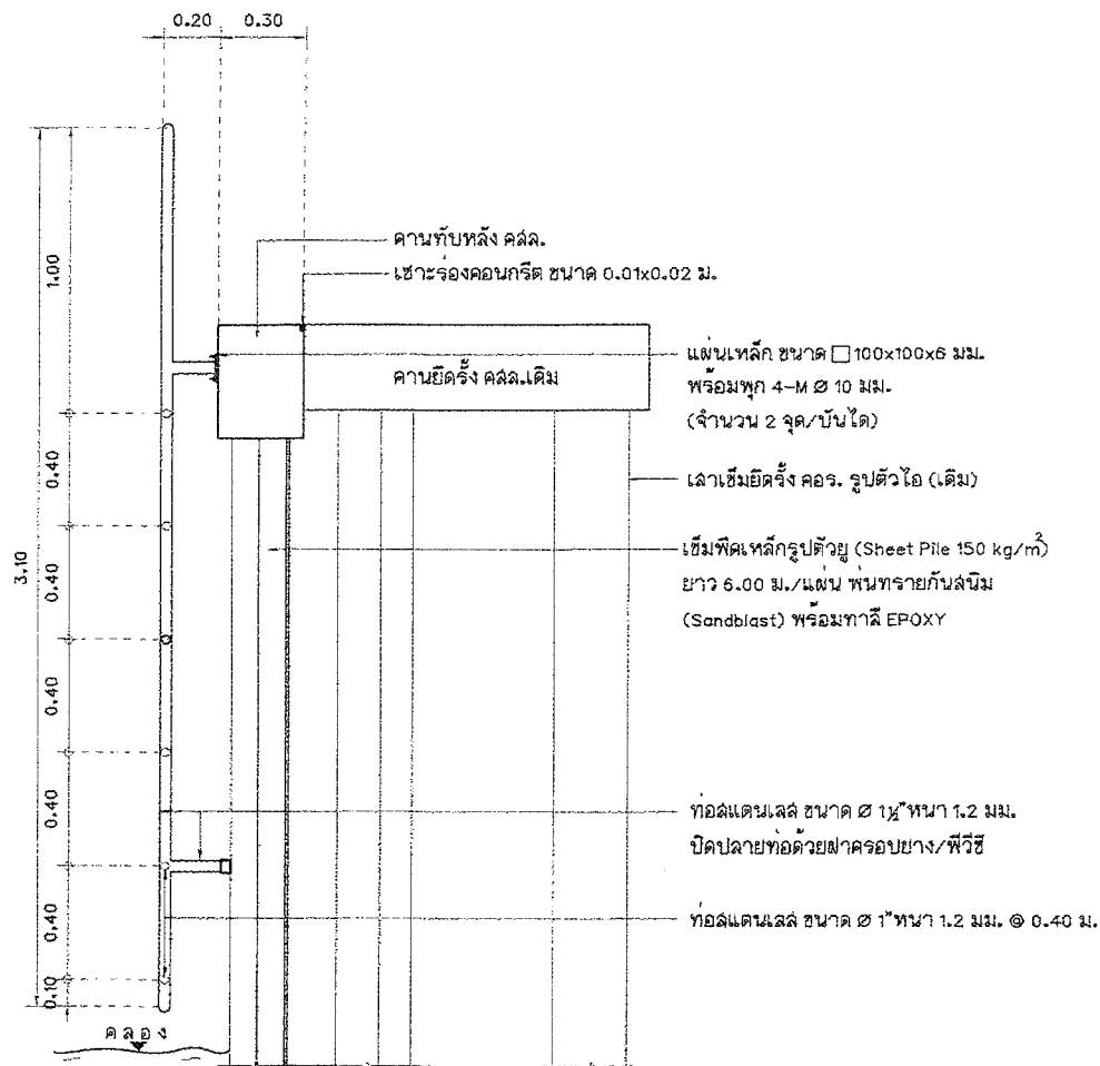
รูปตัด ด้านข้างบ้านใต้ถุน
