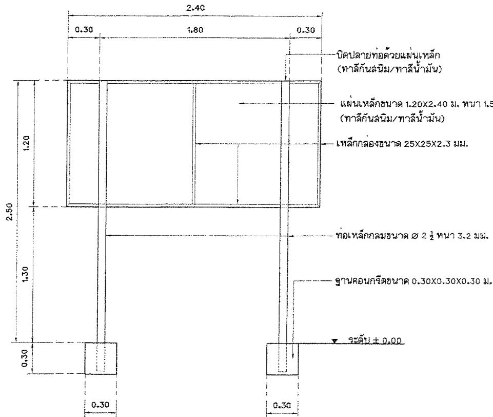
รูปด้านหลังป้ายโครงการ มาตราส่วน 1:25
