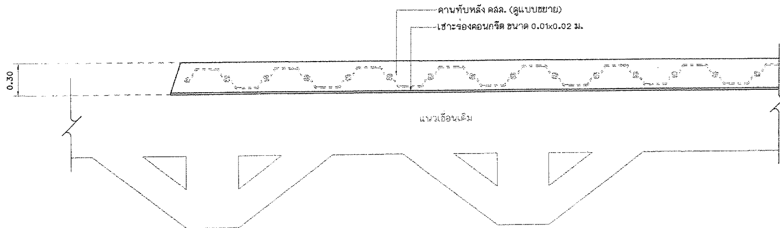
แปลนคานทับหลัง ค.ล.ล.
