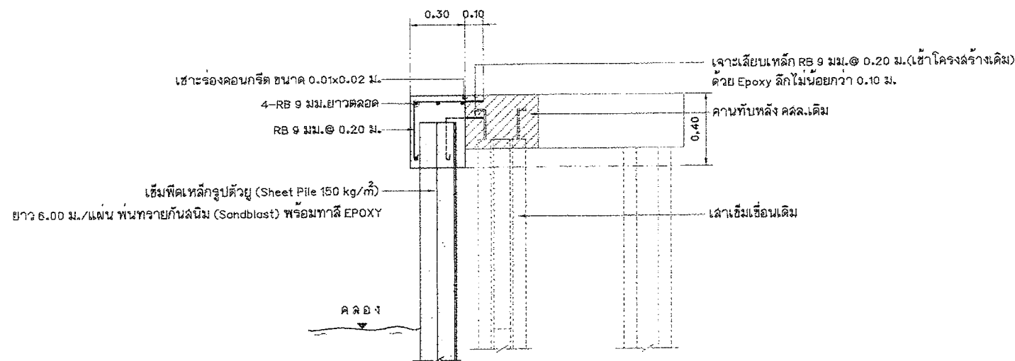
รูปตัด มาตราส่วน 1:20
