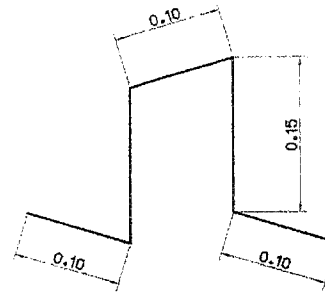
แบบขยายเหล็กขาตั้งรับเหล็กตะแกรง มาตราส่วน 1 : 5
