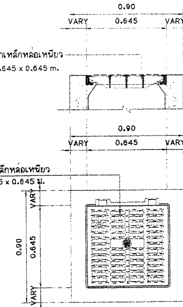
แบบขยายฝาบ่อพักเหล็กหล่อเหนียว 2
