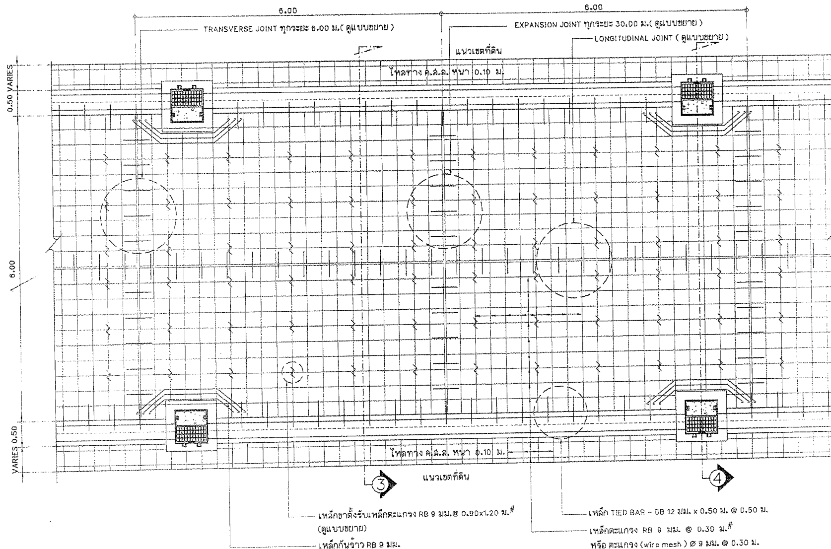
แปลนการวางเหล็กตะแกรงและรอยต่อถนน ค.ล.ล. ช่วง 6.00 เมตร
