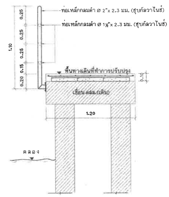
รูปตัด A มาตรฐาน 1:20
