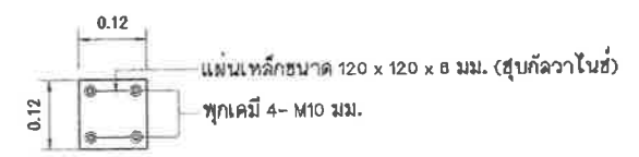
แบบขยายแผ่นเหล็ก มาตรฐาน 1:10
