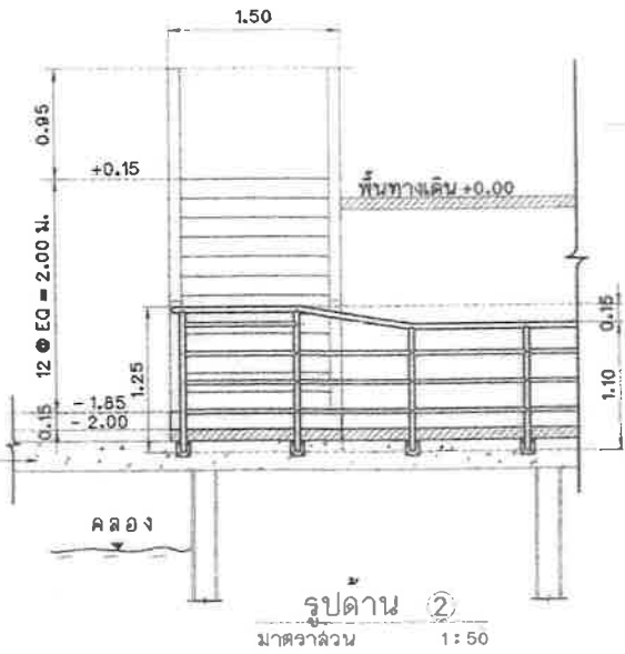
แปลนโครงสร้างบันไดเหล็ก มาตราส่วน 1:50
