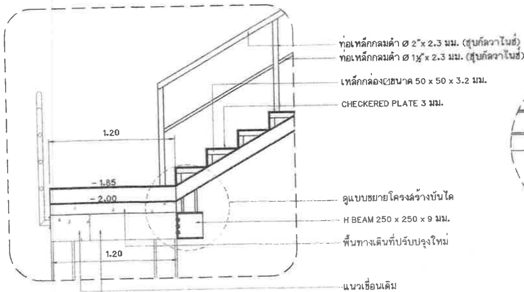
แบบขยาย (๒) มาตราส่วน 1:25
