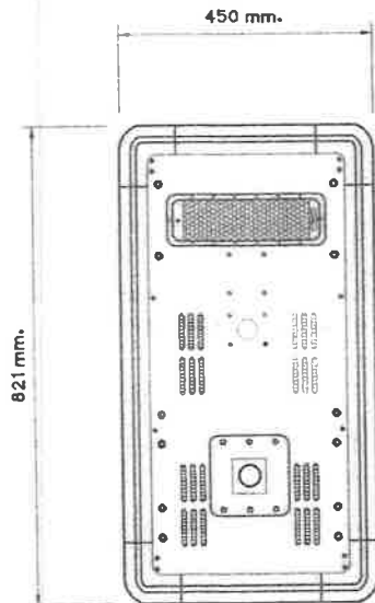
แบบขยายโคมไฟถนนโซล่าเซลล์ มาตราส่วน 1:10
