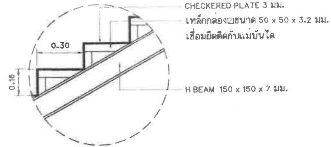
แบบขยายโครงสร้างบันได ไม่มีมาตราส่วน
