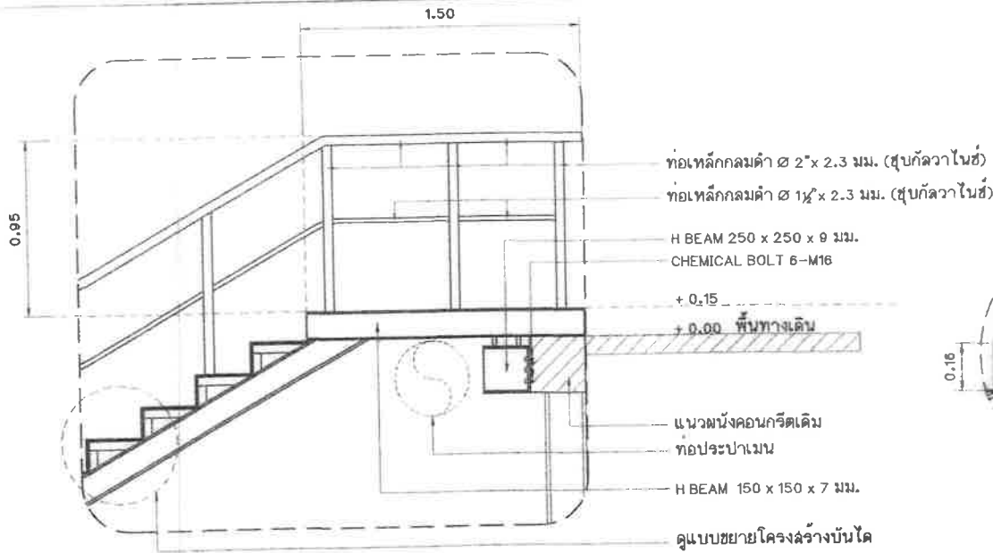
แบบขยาย (๑) มาตราส่วน 1:25
