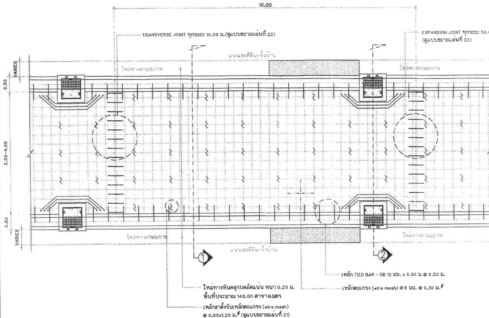
แปลนการวางเหล็กตะแกรงและรอยต่อถนน คสล. (แบบมีไหล่ทางหินคลุก) มาตราส่วน 1 : 50
