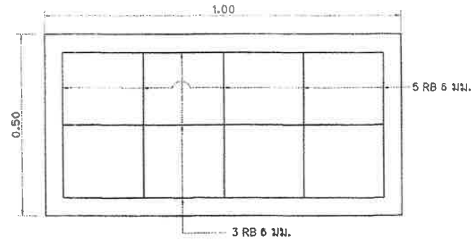
แบบขยายแปลนพื้นพื้นรองท่อ มาตราส่วน 1 : 10
