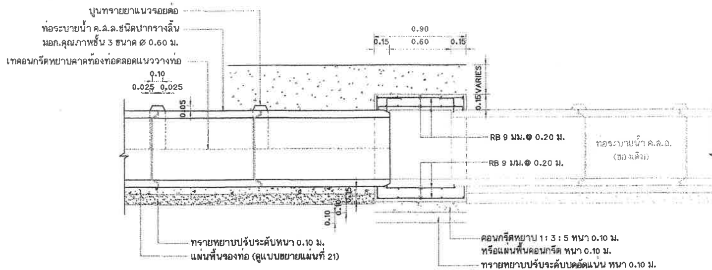
รูปตัดการเชื่อมท่อระบายน้ำของเดิม มาตราส่วน 1:25
