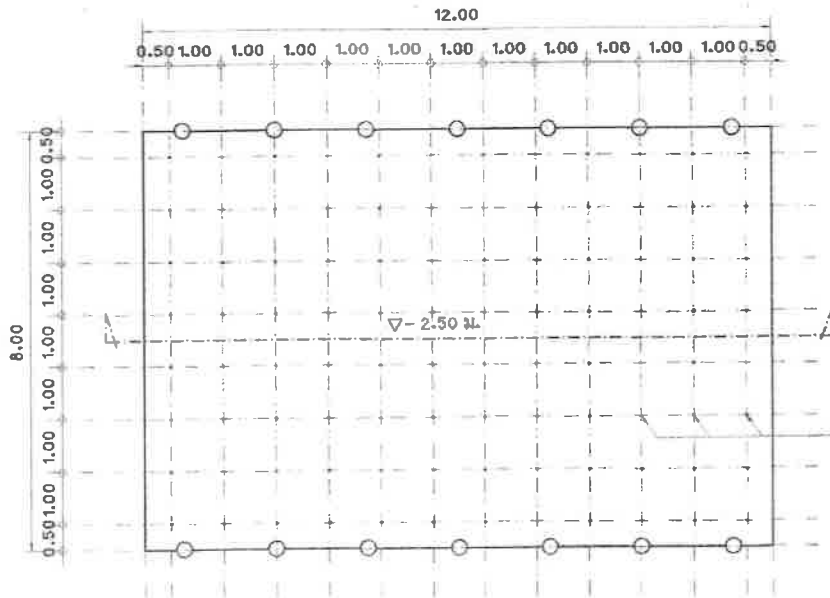
แปลนเสาเข็มดาดท้องคลอง (สะพานที่ 2)
