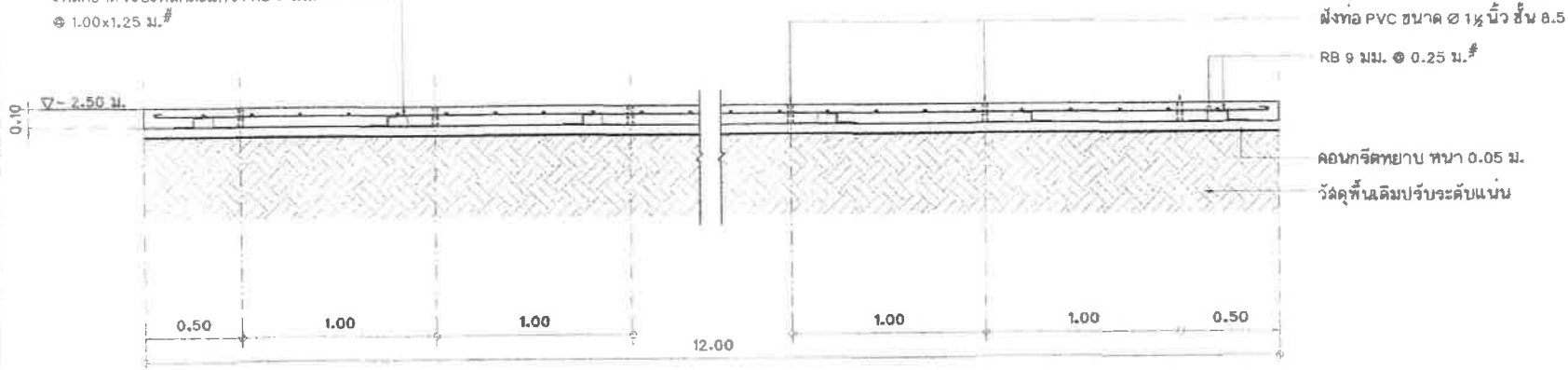
รูปตัดดาดท้องคลอง (สะพานที่ 1) มาตรฐาน 1:25
