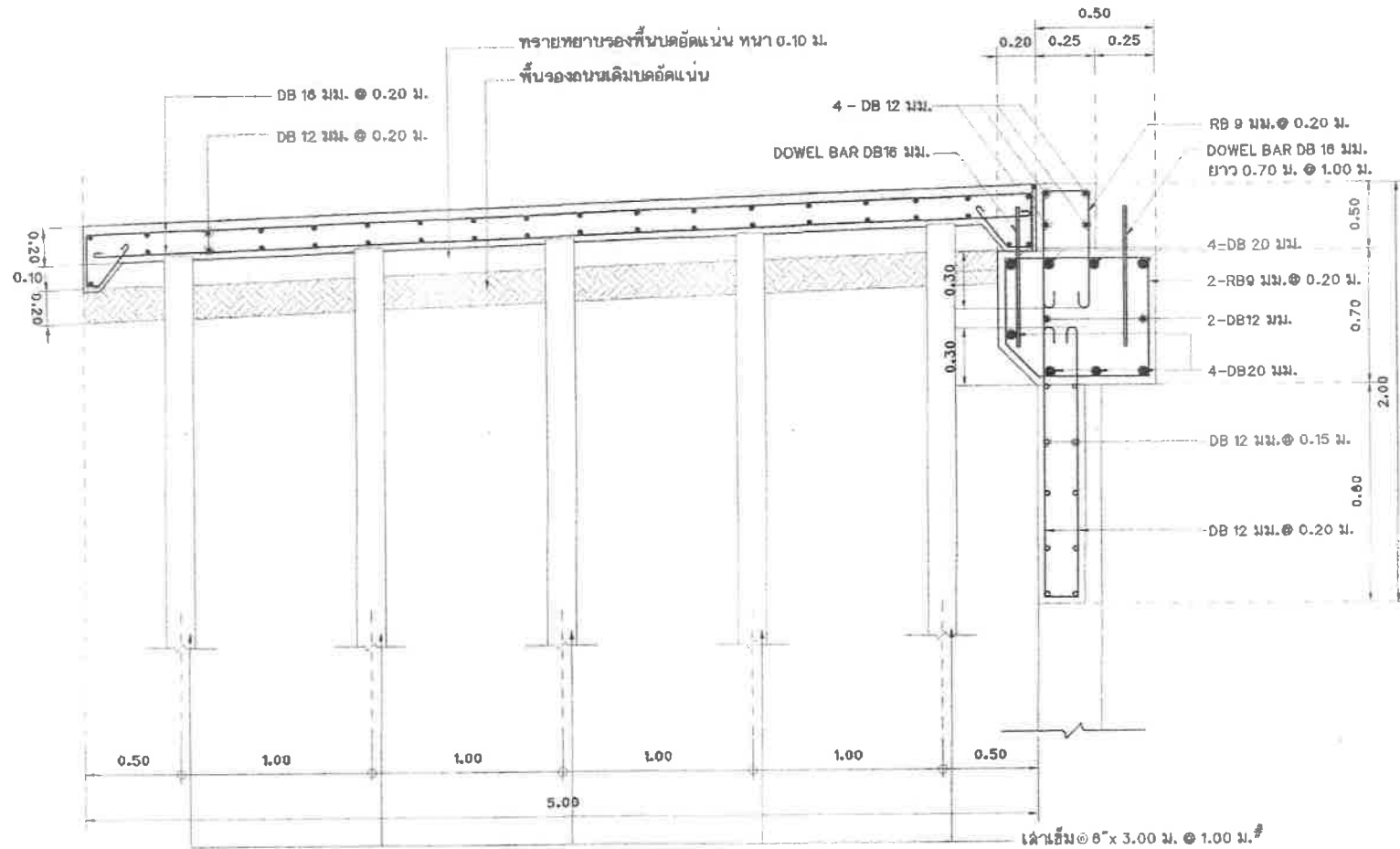
รูปตัดการเชื่อมสะพาน และตีถนบน คลล.(ฝั่งหมู่บ้านประชานีเวค่น 2 ระยะ 3)
