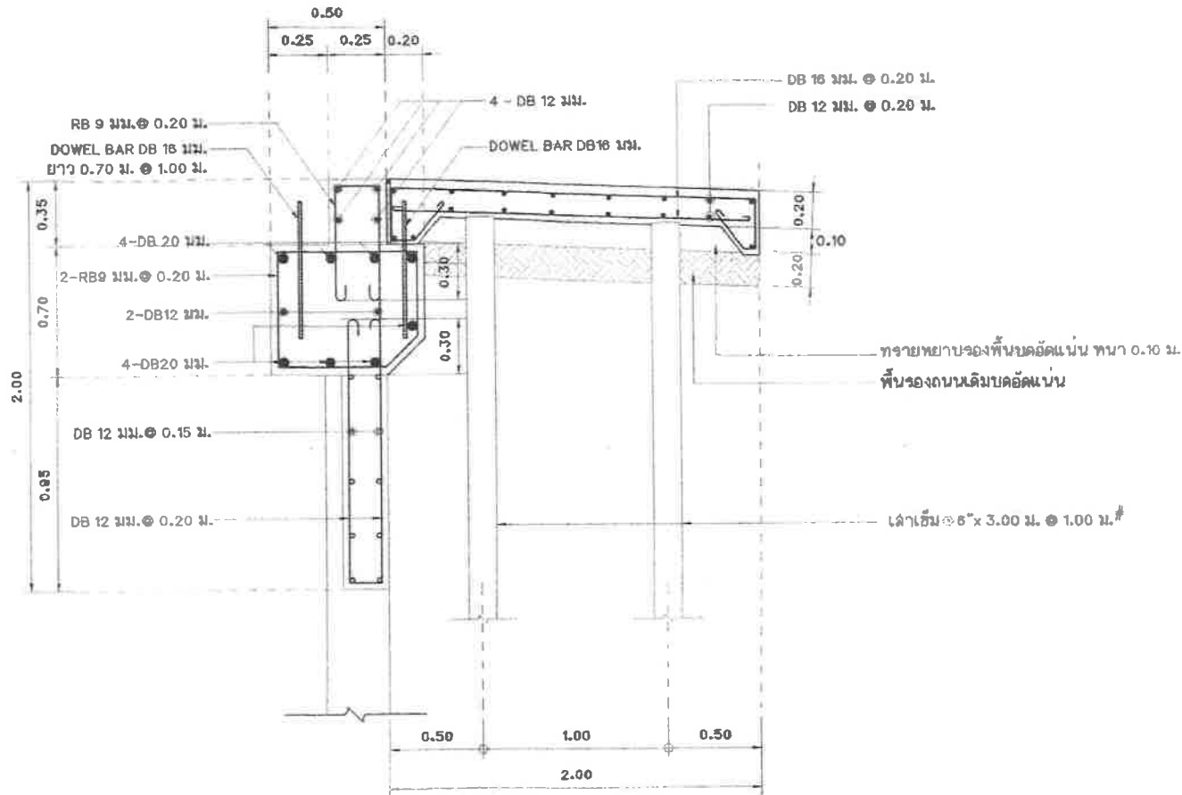
รูปตัดการเชื่อมสะพาน และผิวถนน คสล. มาตรฐาน 1:25
