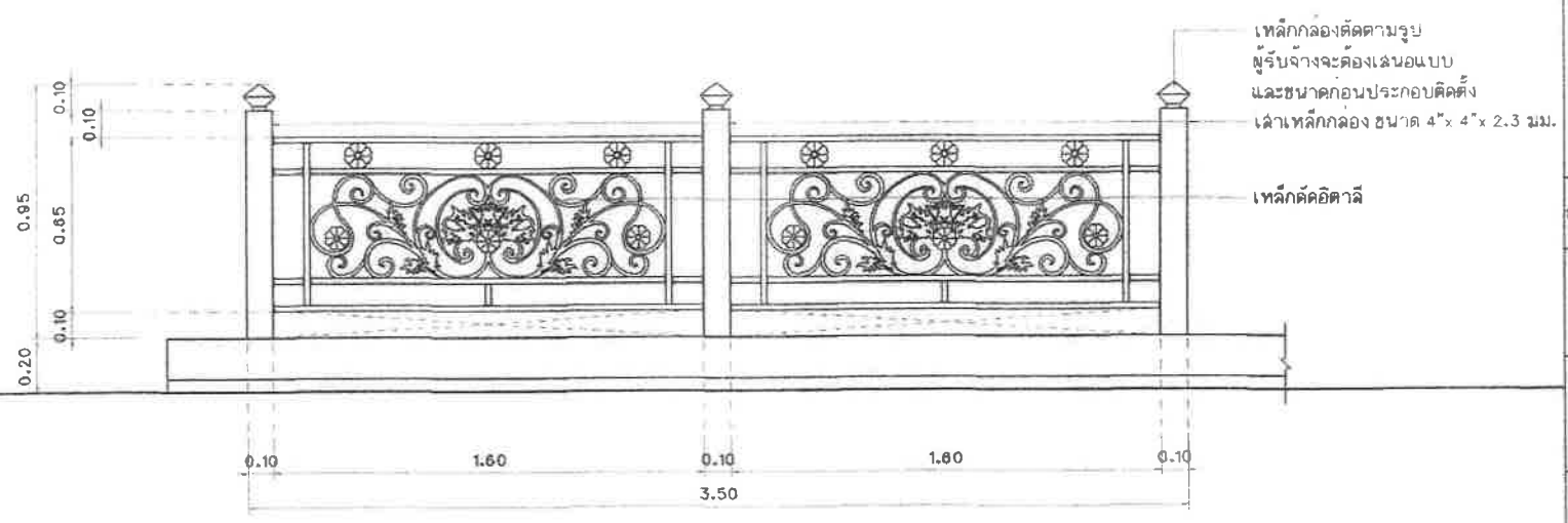
แบบขยายรูปด้านหน้าราวสะพานเหล็กดัดอิตาลี (สะพานที่ 1) มาตราส่วน 1 : 20
