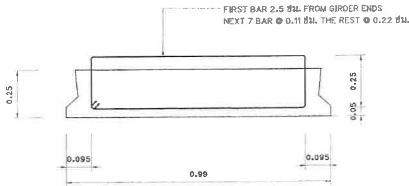
PLANK 8.00 ม. SPAN
