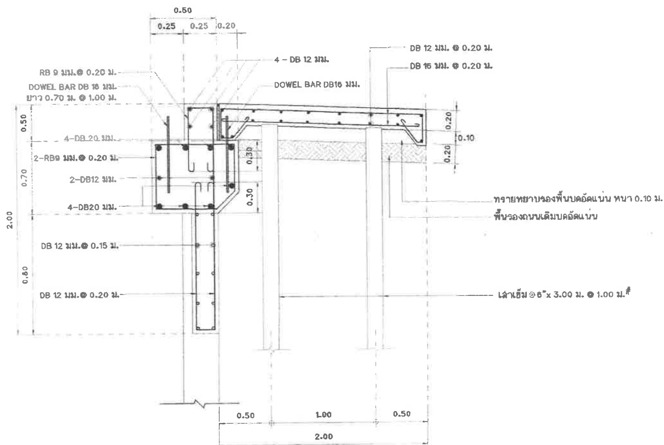
รูปตัดการเชื่อมสะพาน และผิวถนน คสล. (ฝั่งถนนล้ามคคี) มาตราส่วน 1:25
