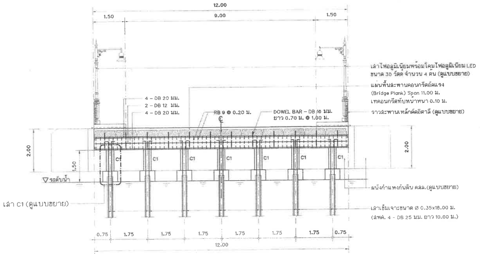
รูปตัดโครงสร้าง A - A (สะพานที่ 1) มาตราส่วน 1:75
