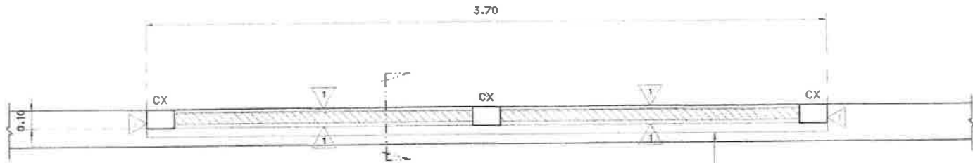
แบบขยายแปลนโครงสร้างป้ายสะพาน คสล. มาตรฐาน 1: 20
