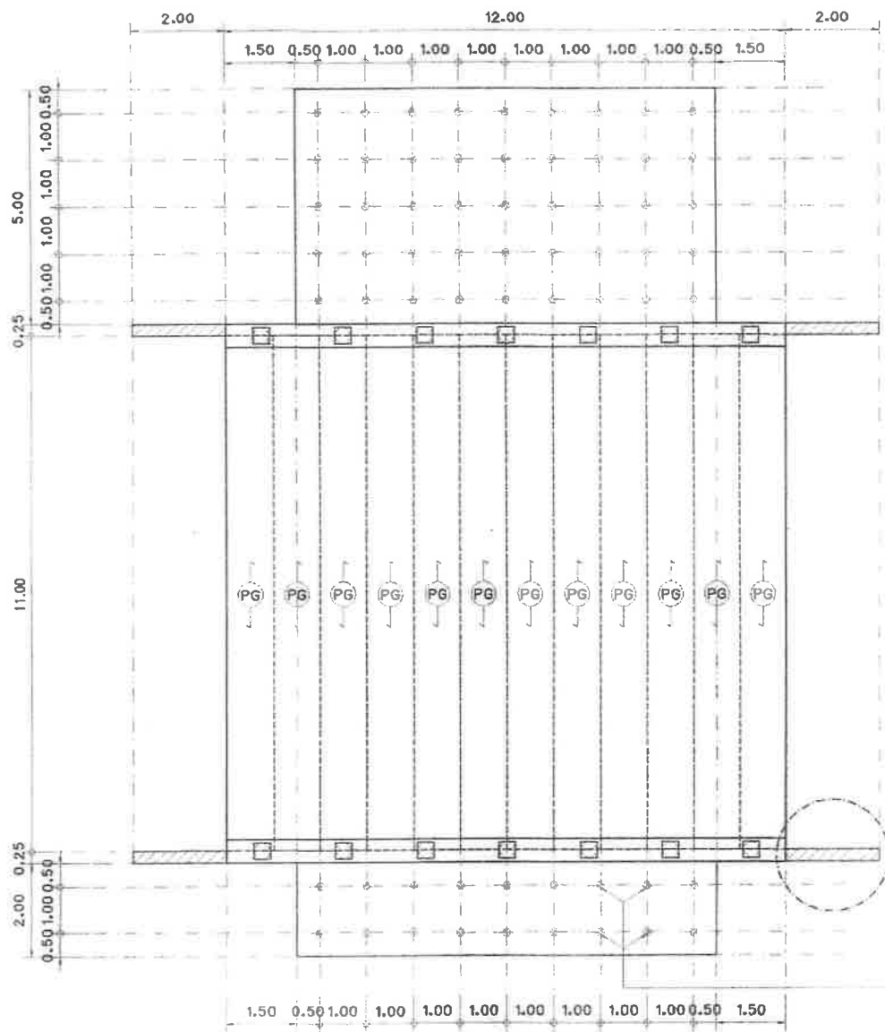
แปลนโครงสร้างสะพาน คสล. (สะพานที่ 1) มาตรฐาน 1 : 100
