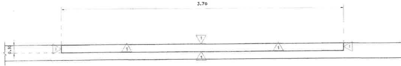
แบบขยายแปลนป้ายสะพาน คลล์. มาตราส่วน 1:20
