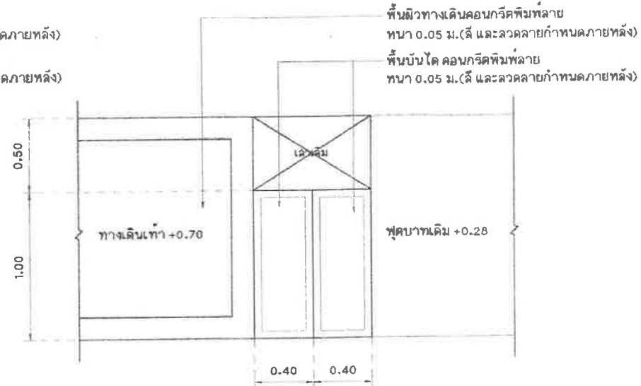
แบบขยายรูปตัดบันได ST2 มาตราส่วน 1:25
