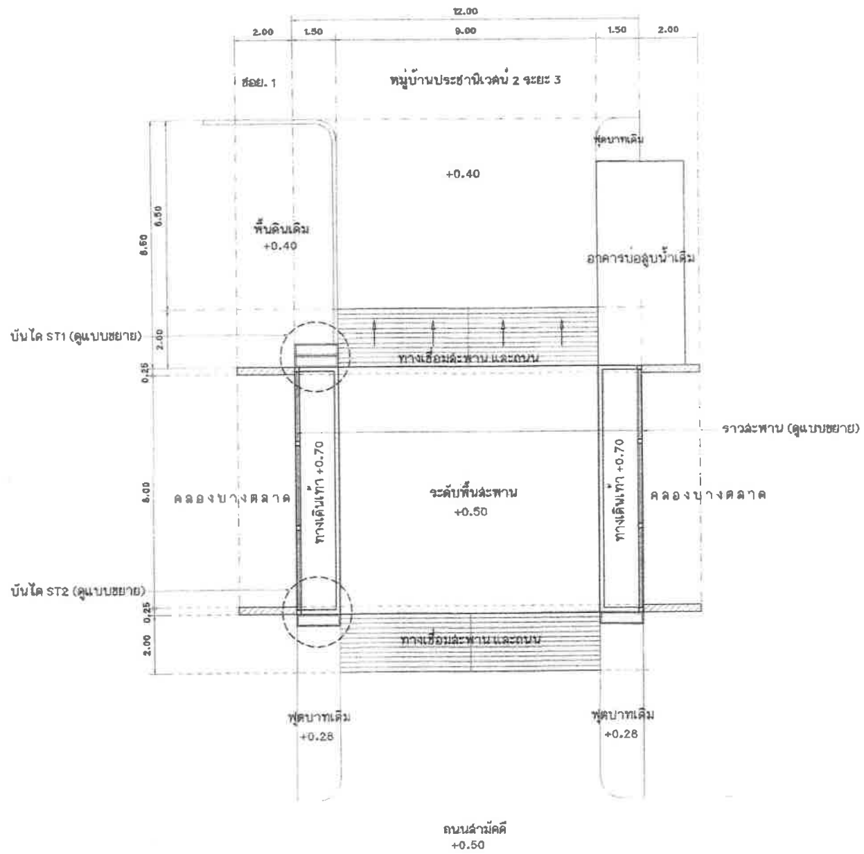
แปลนสะพาน คสล. (สะพานที่ 2) มาตรฐาน 1:125
