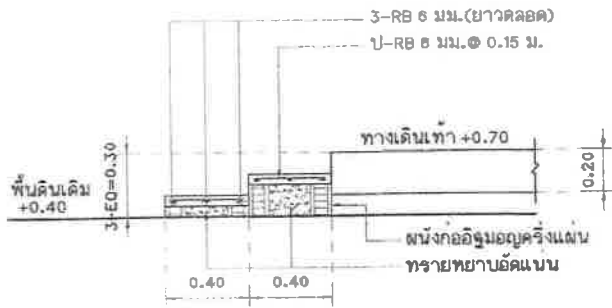
แบบขยายรูปตัดบันได ST1 มาตราส่วน 1:25
