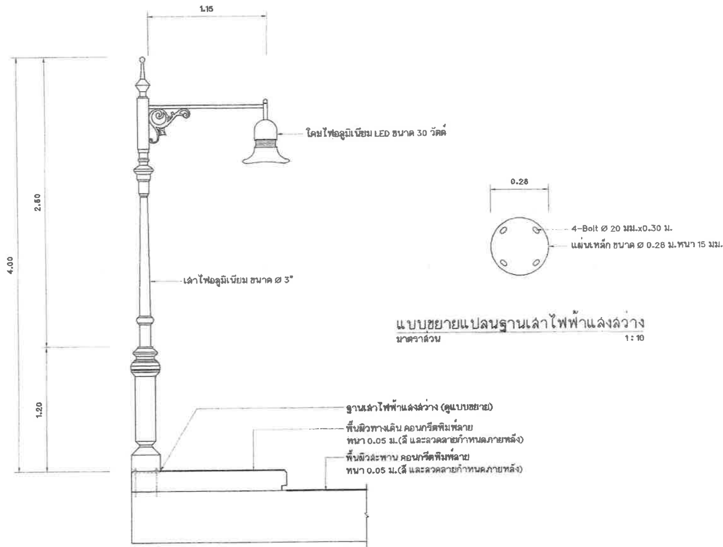
แบบขยายโคมไฟฟ้าแสงสว่าง มาตราส่วน 1 : 25
