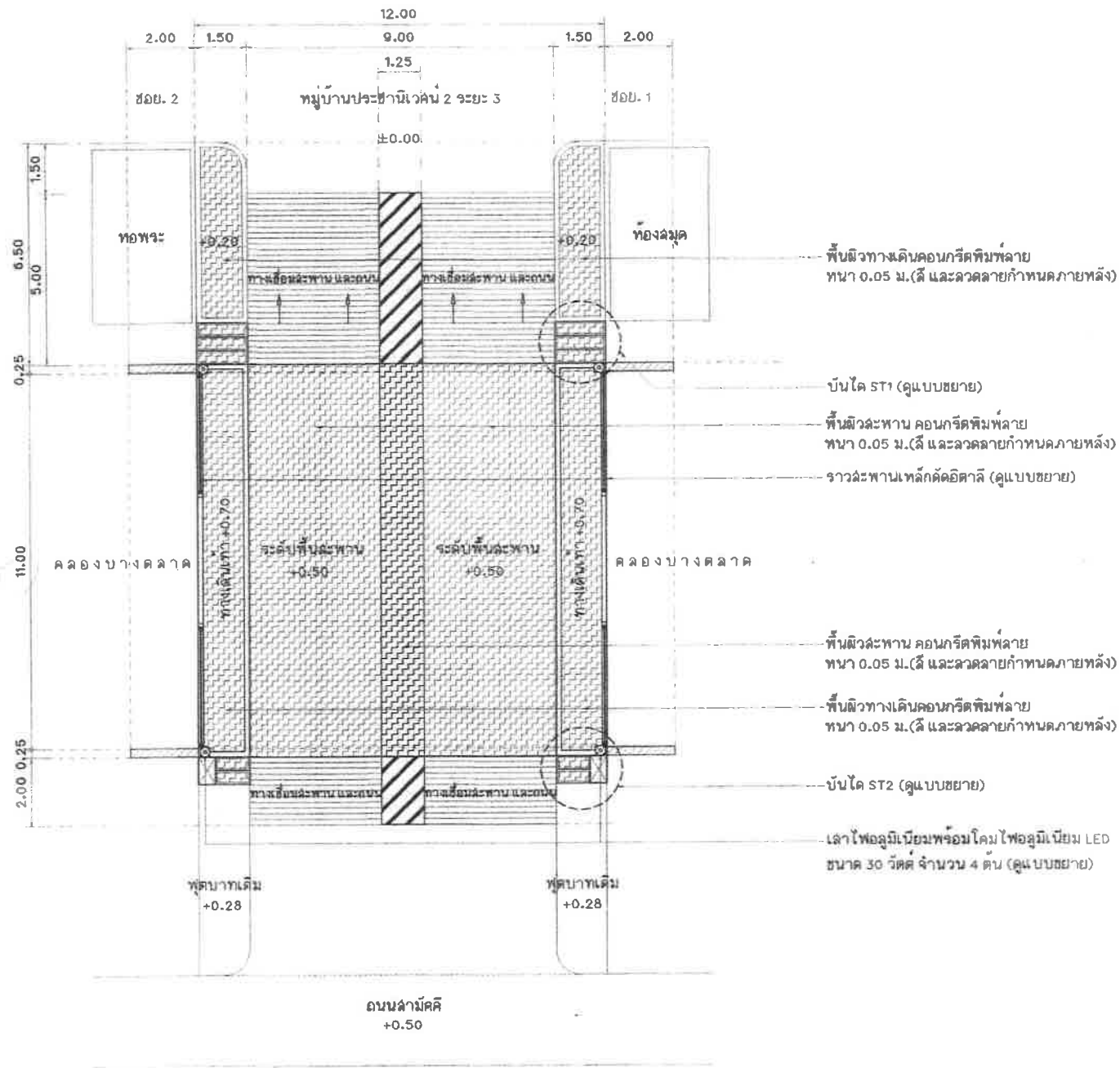
ถนนลำคิ +0.50 แปลนสะพาน คสล. (สะพานที่ 1) มาตราส่วน 1 : 125
