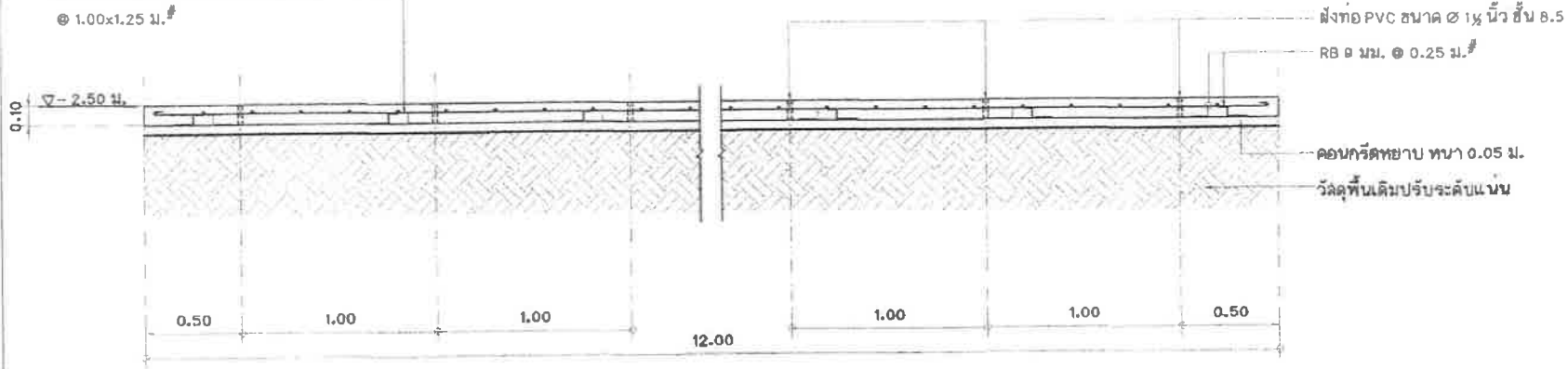
รูปตัดดาดท้องคลอง (สะพานที่ 2)
