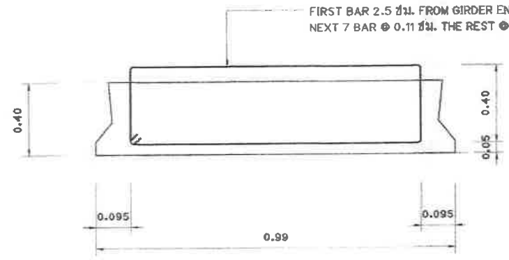
PLANK 11.00 ม. SPAN
