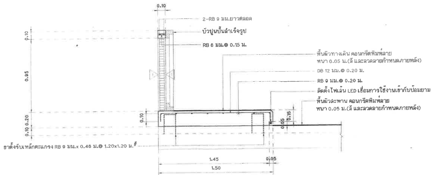
แบบขยายรูปตัดโครงสร้างป้ายสะพาน คสล. พื้นทางเท้า มาตรฐาน 1: 20
