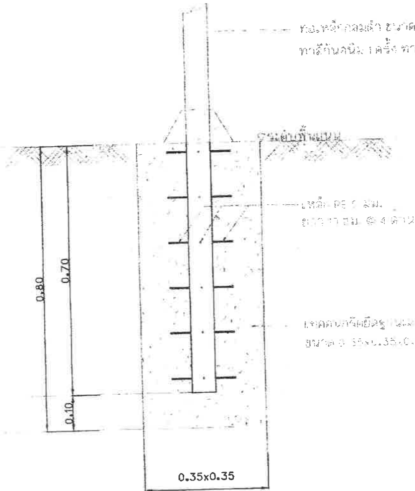
แบบขยายฐานราก ② (ในกรณีเจาะยึดคอนกรีต)
