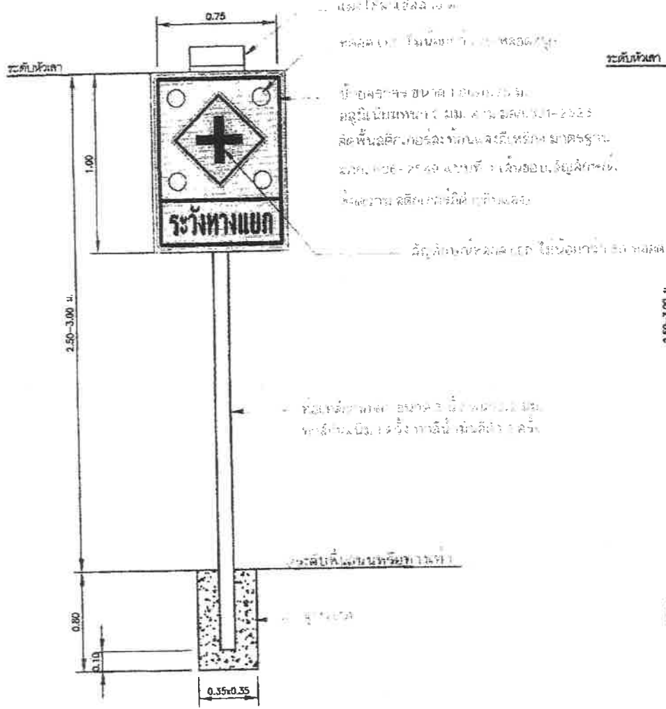
แบบร่าง 103-01-01-01 ระวังทางแยก (ระวังไฟจราจร)
