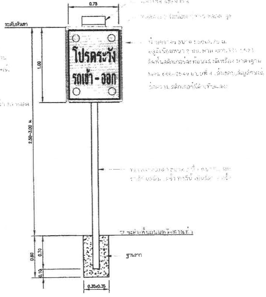
แบบร่าง 103-01-01-02 ระวังรถเข้า-ออก
