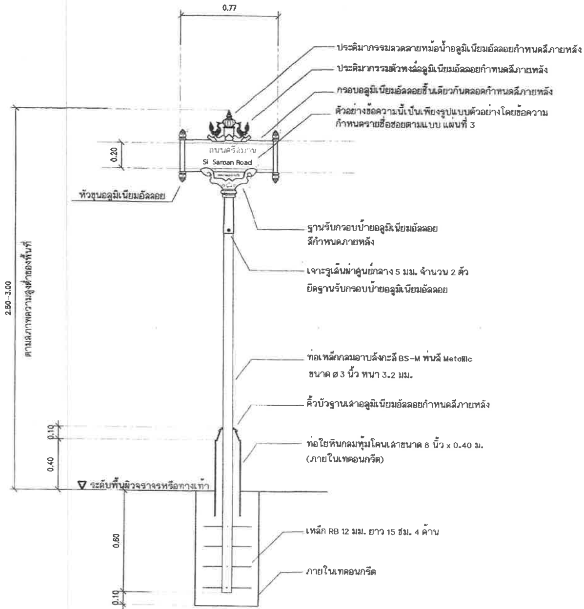
รูปตัดการติดตั้ง (แบบที่1) มาตราส่วน 1:20
