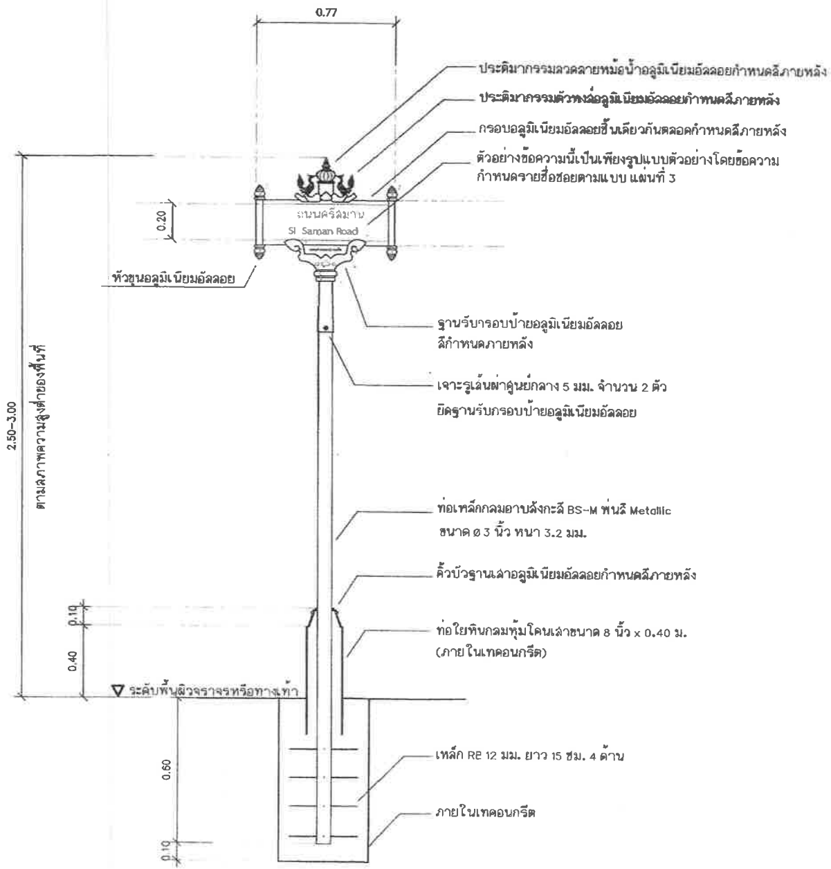
รูปตัดการติดตั้ง (แบบที่ 1) มาตรฐาน 1:20
