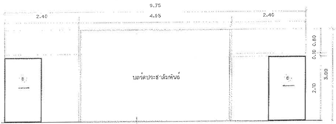
รูปด้านนอกผนังสำเร็จรูป (เวทึ) มาตราส่วน 1:50
