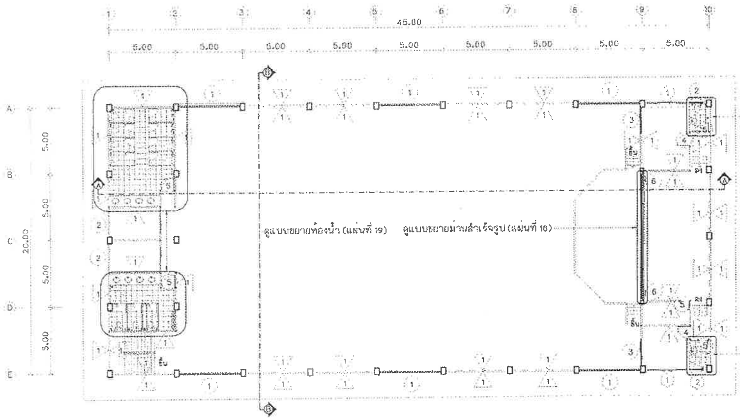
แปลนพื้นที่ชั้นกลางที่ปรับปรุง มาตรฐาน 1:200
