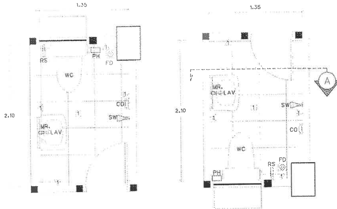
แบบขยายห้องน้ำ ขนาดกว้าง ๒:25
