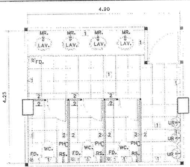
แบบขยายห้องน้ำ มาตรฐาน ขนาดจริง 1:50
