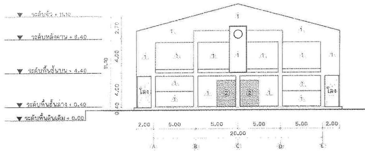
รูปด้าน 1 ที่ปรับปรุง มาตราส่วน 1:200
