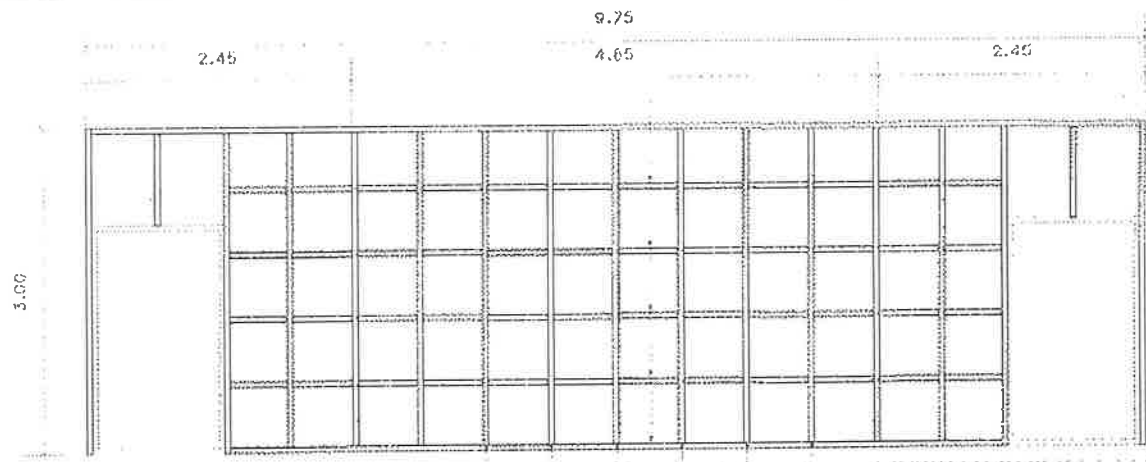
ขยายโครงสร้างผนังสำเร็จรูป (เวทท์) มาตราส่วน 1:50
