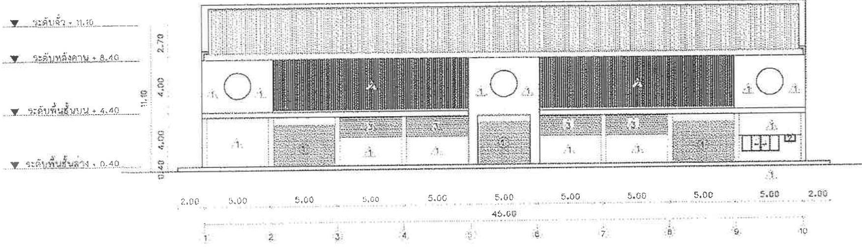
รูปด้าน 3 ที่ปรับปรุง มาตราส่วน 1:200
