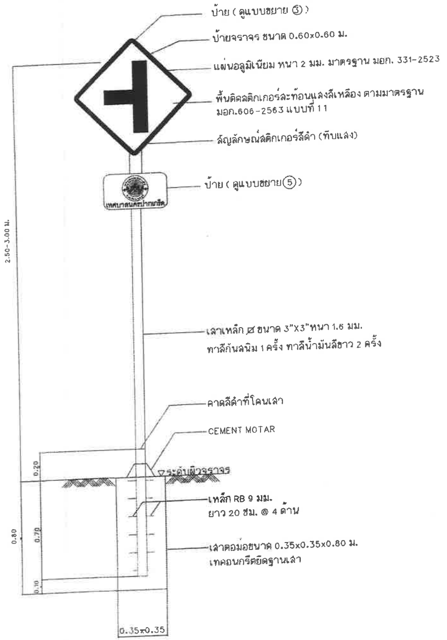
รูปด้านหน้า-ด้านหลังแบบติดตั้งป้ายจราจร (รูปแบบที่ 3)
