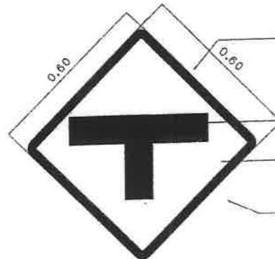
แบบขยายป้าย ④
