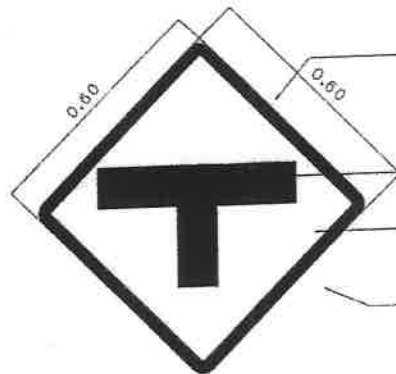
แบบขยายป้าย ④ มาตราส่วน 1:10
