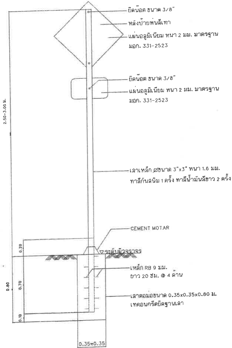
รูปด้านหน้า-ด้านหลังแบบติดตั้งป้ายจราจร (รูปแบบที่ 8)
