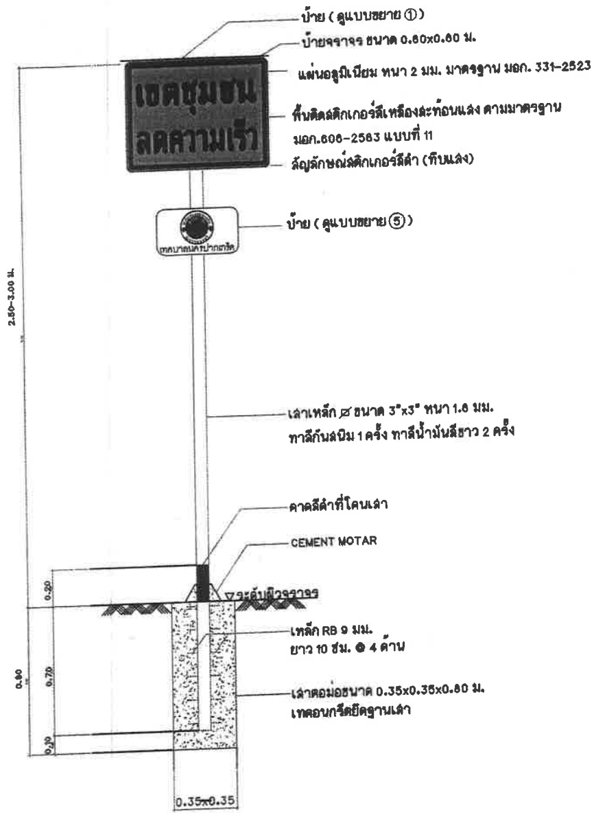
รูปด้านหน้า-ด้านหลังแบบติดตั้งป้ายจราจร (รูปแบบที่ 1) มาตรฐาน 1:20
