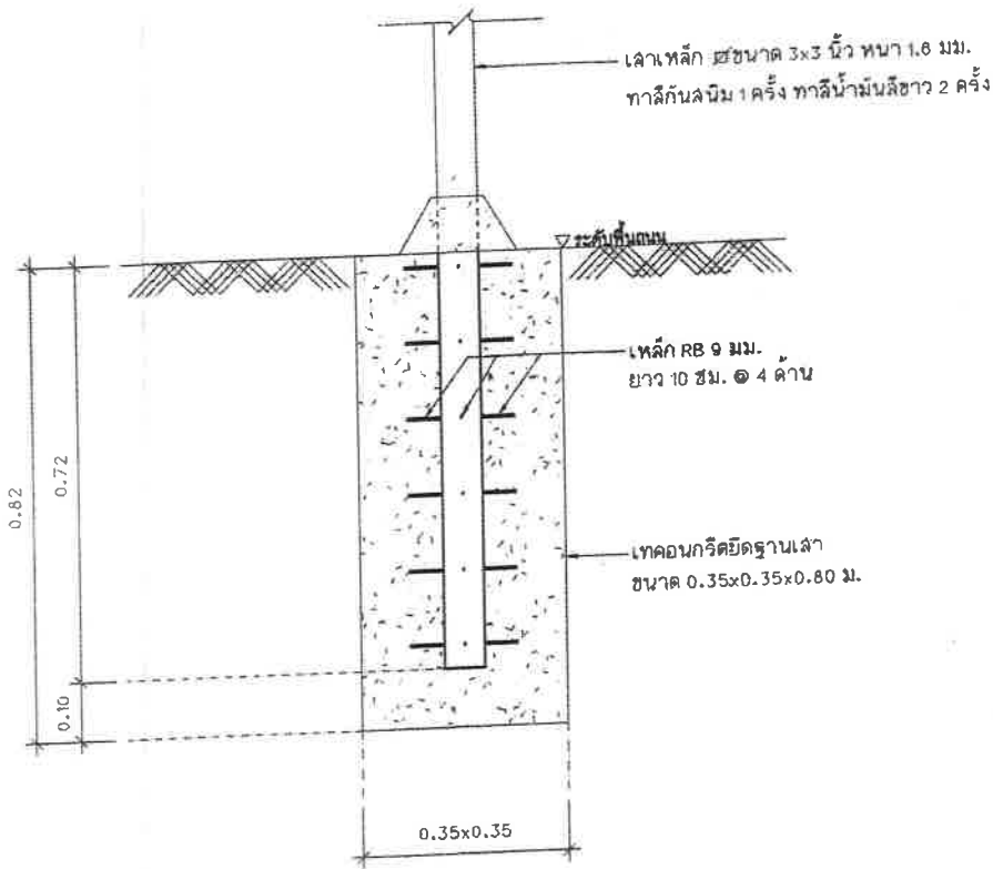
แบบขยายฐานราก มาตราส่วน 1:10
