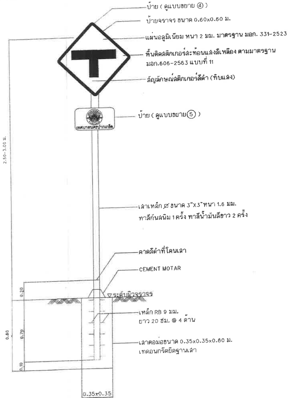
รูปด้านหน้า-ด้านหลังแบบติดตั้งป้ายจราจร (รูปแบบที่ 8) มาตรฐาน 1:20
