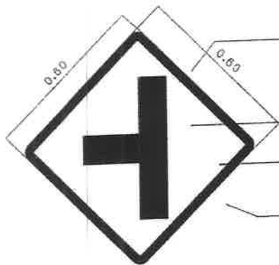
แบบขยายป้าย ③ มาตราส่วน 1:10
