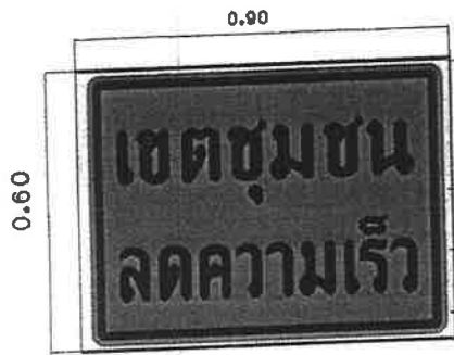
แบบขยายป้าย ① มาตราส่วน 1:10
