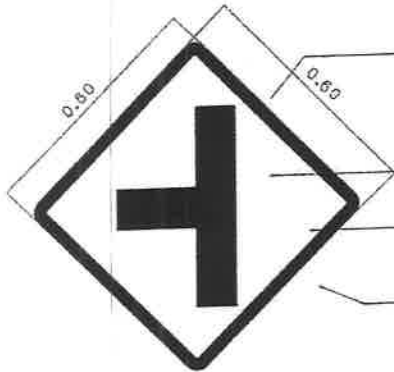
แบบขยายป้าย ③
