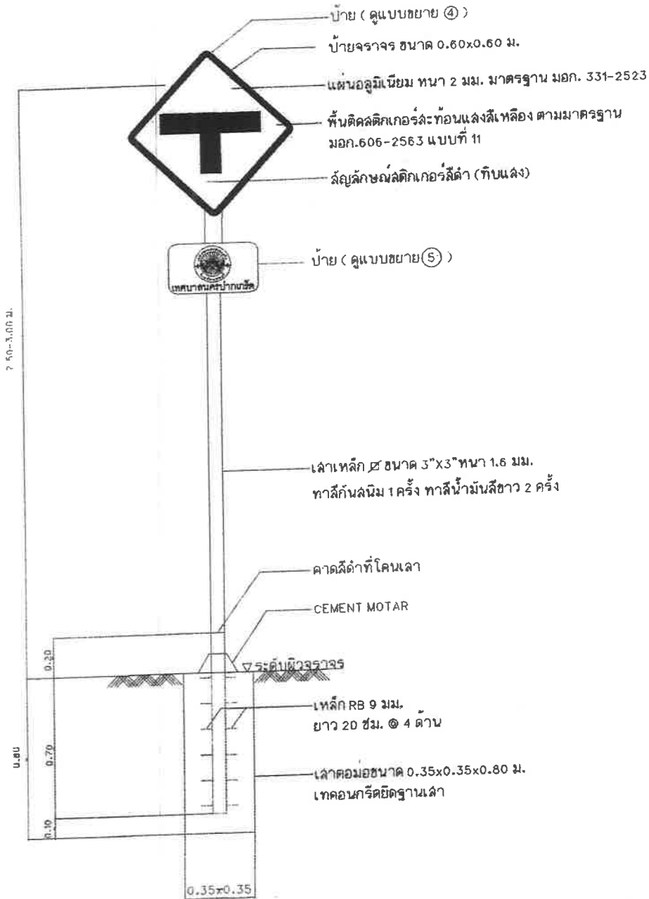
รูปด้านหน้า-ด้านหลังแบบติดตั้งป้ายจราจร (รูปแบบที่ 8)
