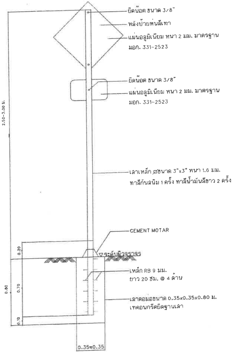
รูปด้านหน้า-ด้านหลังแบบติดตั้งป้ายจราจร (รูปแบบที่ 8) มาตรฐาน 1:20
