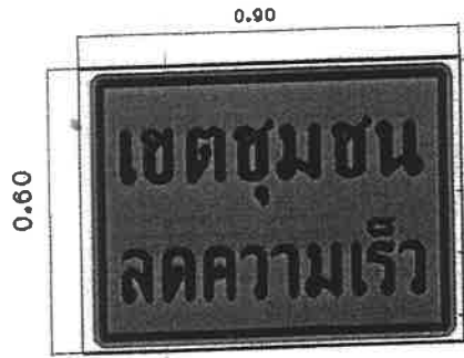
แบบขยายป้าย ①
